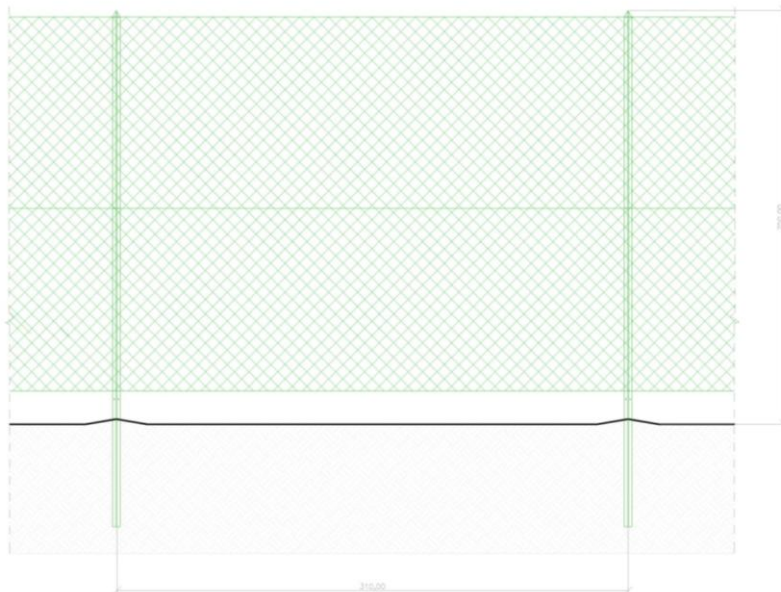
Figura 12: Prospetto tipo recinzione perimetrale con apertura inferiore (20-30 cm) per il passaggio della piccola fauna.
