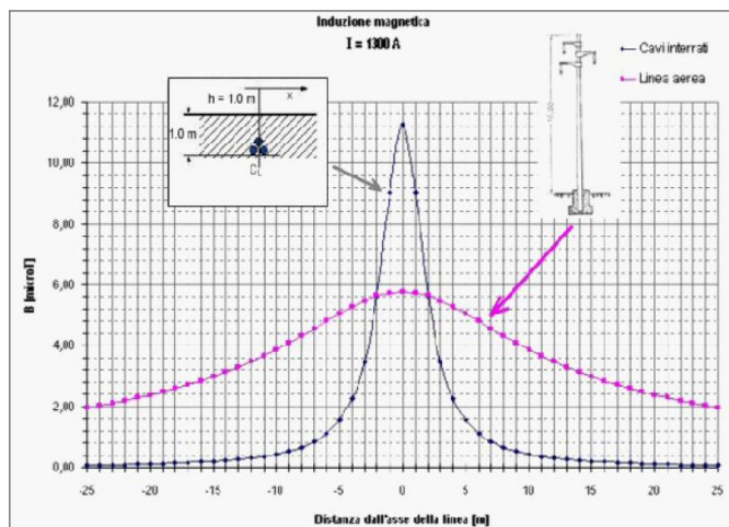
Figura 24: Attenuazione dell'induzione magnetica dovuta all'interrimento dei cavi.
