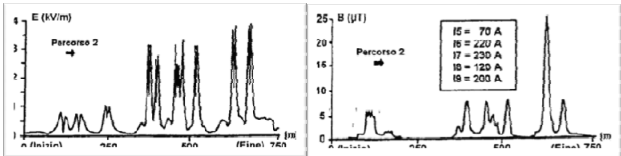
Fig. 4 - Risultati della misura dei campi elettrici e magnetici effettuate lungo le vie interne della sezione a 132 kV della stazione riportata in fig. 1
