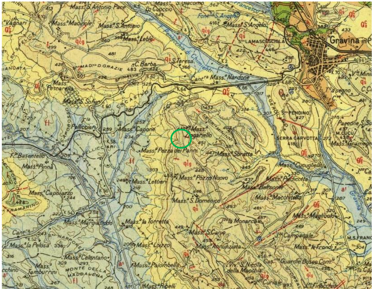
Fig. 1 – Carta geologica di Italia 188 "Gravina in Puglia" – con indicazione dell'area di realizzazione della nuova stazione elettrica.
