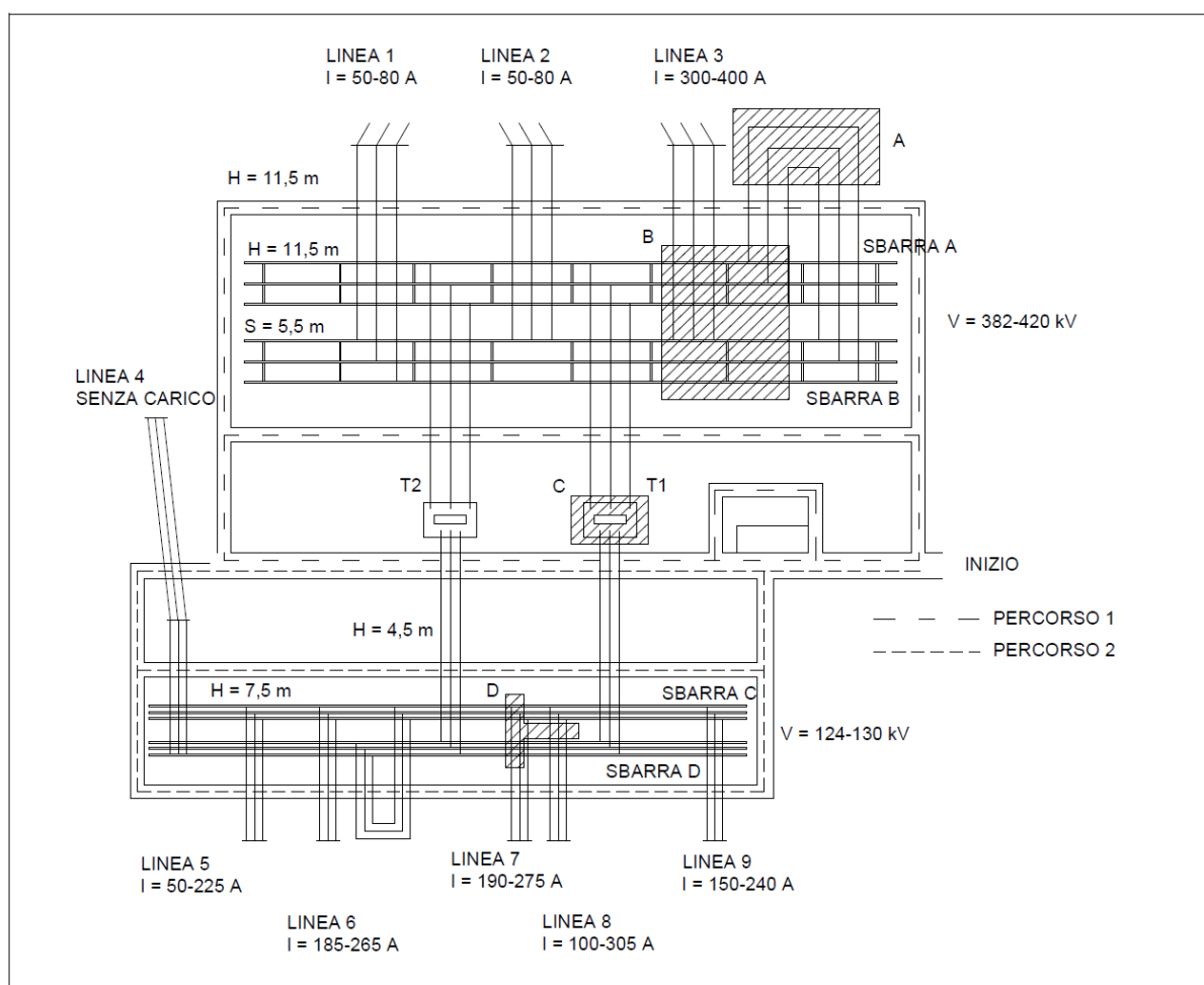
Fig. 2 – Pianta di una tipica stazione 380/150/132 kV con l'indicazione delle principali distanze fase-fase ( S ) e fase-terra ( H ) e delle variazioni delle tensioni e delle correnti durante la fase di misurazioni di campo elettrico e magnetico.
