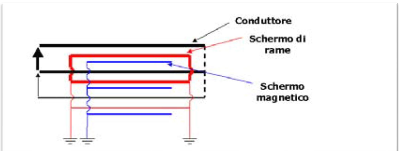
Figura 22: schema bidimensionale del cavo unipolare e della messa a terra degli schermi- tecnica "solid bonding"
