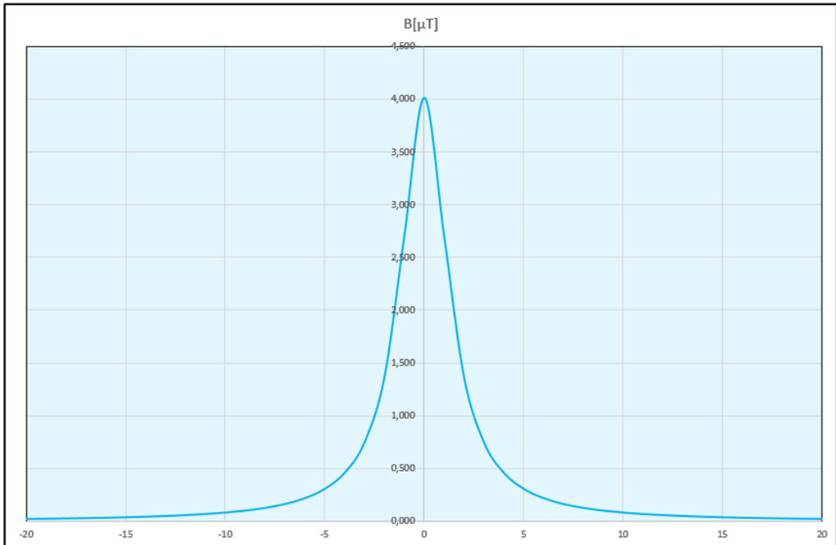
Figura 8: Induzione magnetica generata durante l'esercizio dalla dorsale MT 30 kV da 630 mm 2 valutata ai sensi della Norma CEI 211-4 – Guida ai metodi di calcolo dei campi elettrici e magnetici generati da linee elettriche. Fasi disposte a trifoglio, intensità di corrente I = 578 A, profondità di posa 1,40 m
