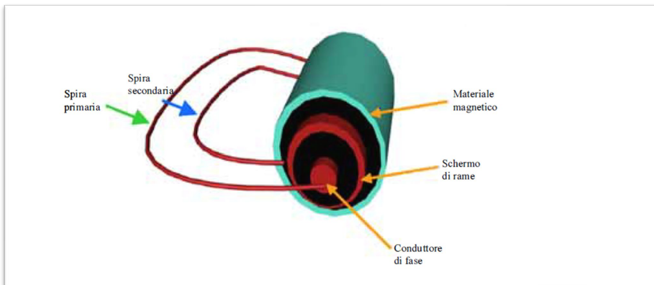
Figura 23: schema tridimensionale del cavo a debole emissione di campo magnetico- tecnica "Solid-bonding"
