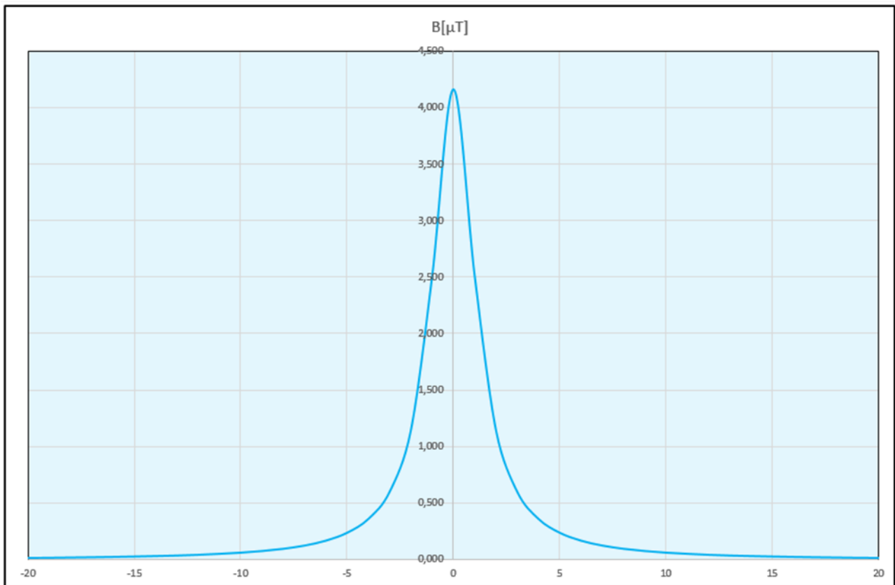
Figura 7: Induzione magnetica generata durante l'esercizio dalla linea MT 30 kV n° 2 da 500 mm 2 valutata ai sensi della Norma CEI 211-4 – Guida ai metodi di calcolo dei campi elettrici e magnetici generati da linee elettriche. Fasi disposte a trifoglio, intensità di corrente I = 482 A, profondità di posa 1,20 m
