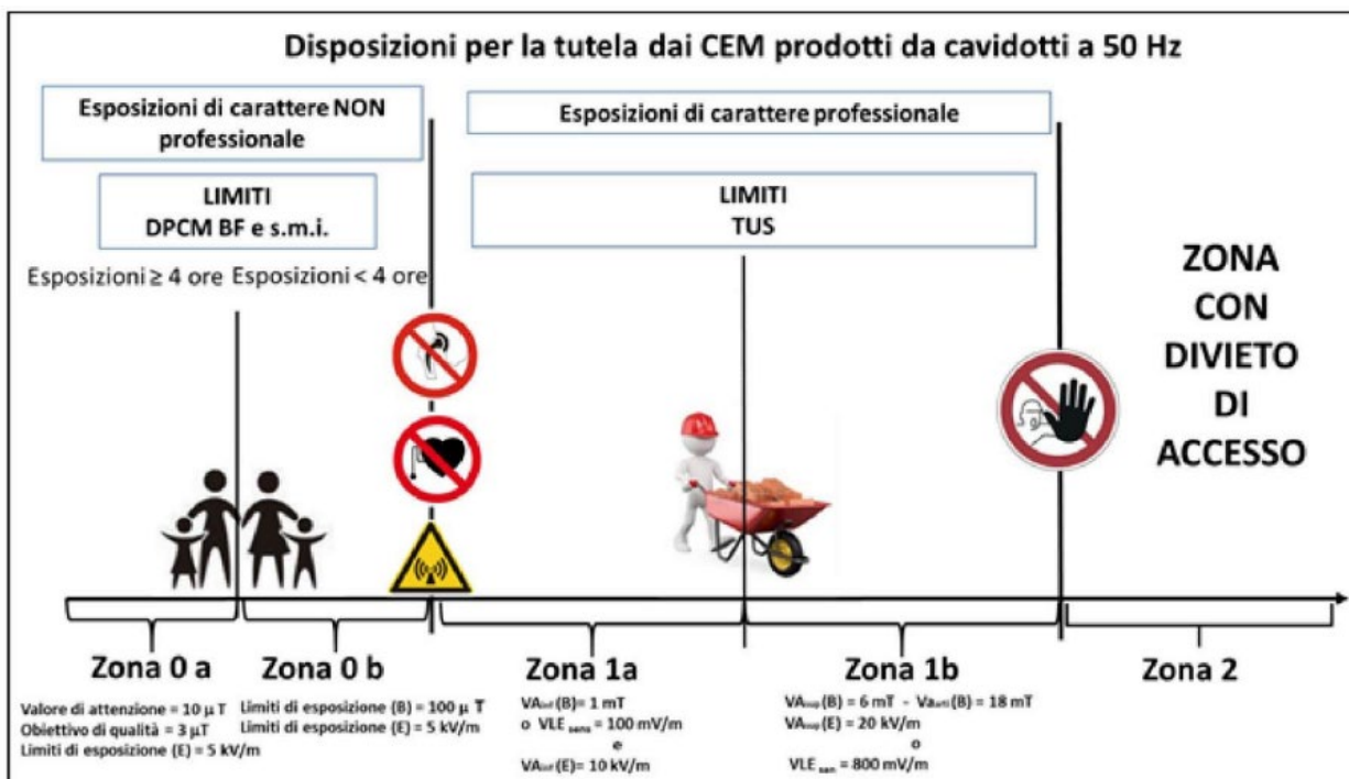
Figura 16: Misure di prevenzione e protezione per la tutela dai CEM prodotti da cavidotti a 50 Hz
