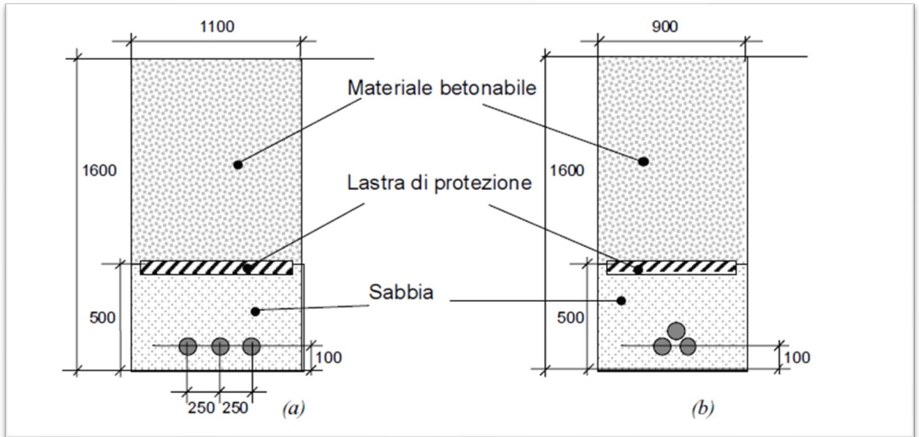
Figura 21: schermatura cavi elettrici interrati
