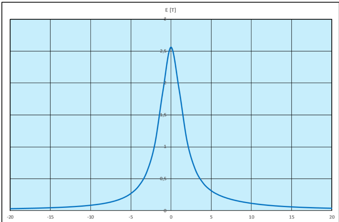
Figura 14: Campo elettrico generato dalla Linea durante l'esercizio valutato applicando la procedura della Norma CEI 211-4 - Guida ai metodi di calcolo dei campi elettrici e magnetici generati da linee elettriche
