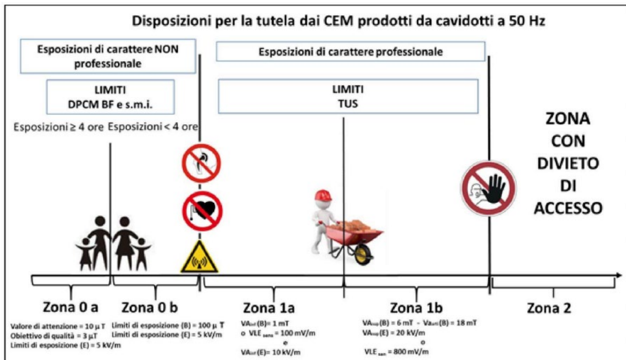
Figura 9: Misure di prevenzione e protezione per la tutela dai CEM prodotti da cavidotti a 50 Hz
