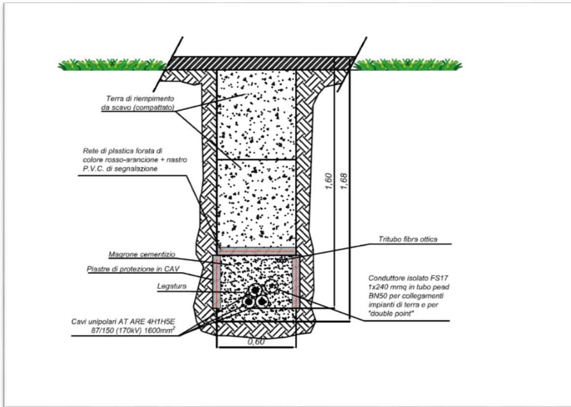
Figura 13: tipico di posa cavo AT 150 kV di collegamento con la Stazione Elettrica RTN
