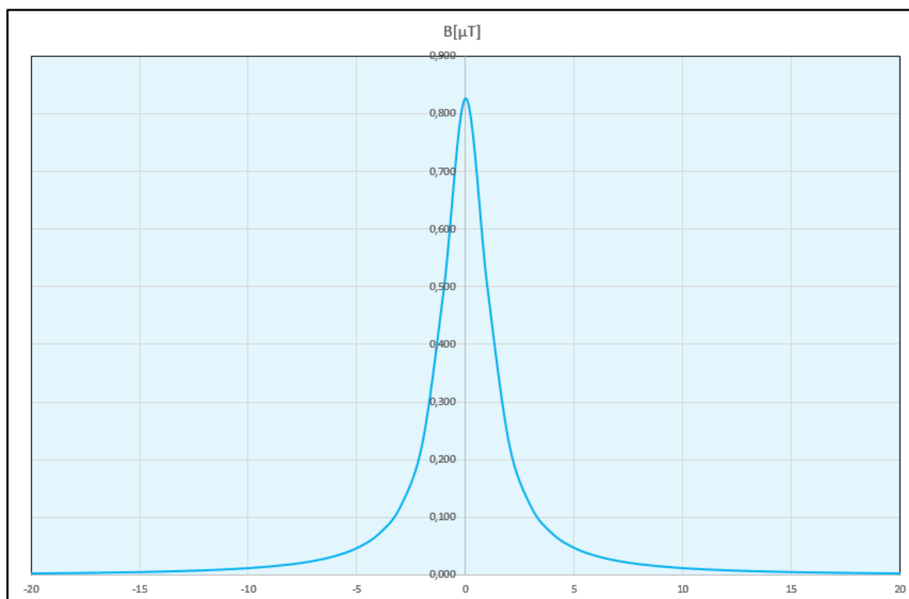
Figura 6: Induzione magnetica generata durante l'esercizio dalla linea MT 30 kV n° 1 da 150 mm 2 valutata ai sensi della Norma CEI 211-4 – Guida ai metodi di calcolo dei campi elettrici e magnetici generati da linee elettriche. Fasi disposte a trifoglio, intensità di corrente I = 97 A, profondità di posa 1,20 m
