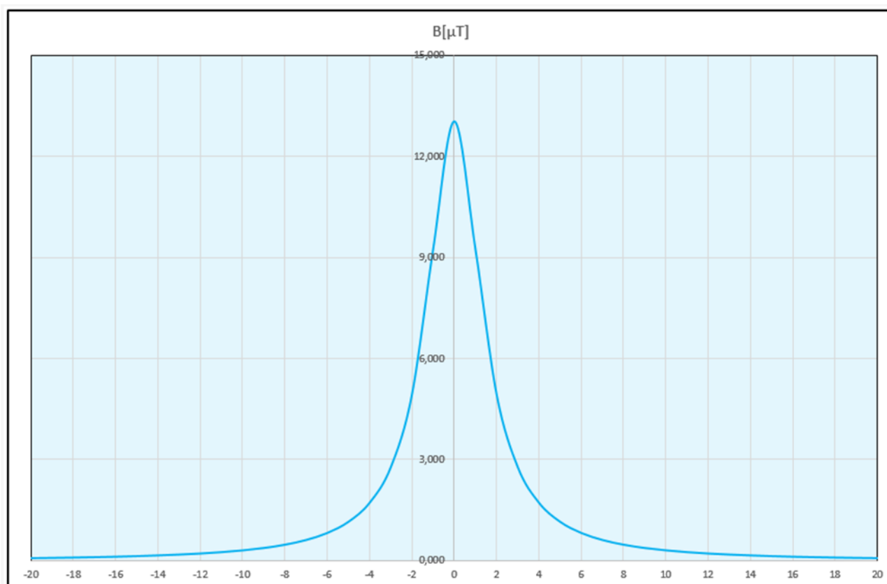
Figura 15: induzione magnetica generata durante l'esercizio dalla linea AT 150 kV di collegamento con la Stazione Elettrica Terna, valutata applicando la procedura delle Norma CEI 211-4 – Guida ai metodi di calcolo dei campi elettrici e magnetici generati da linee elettriche
