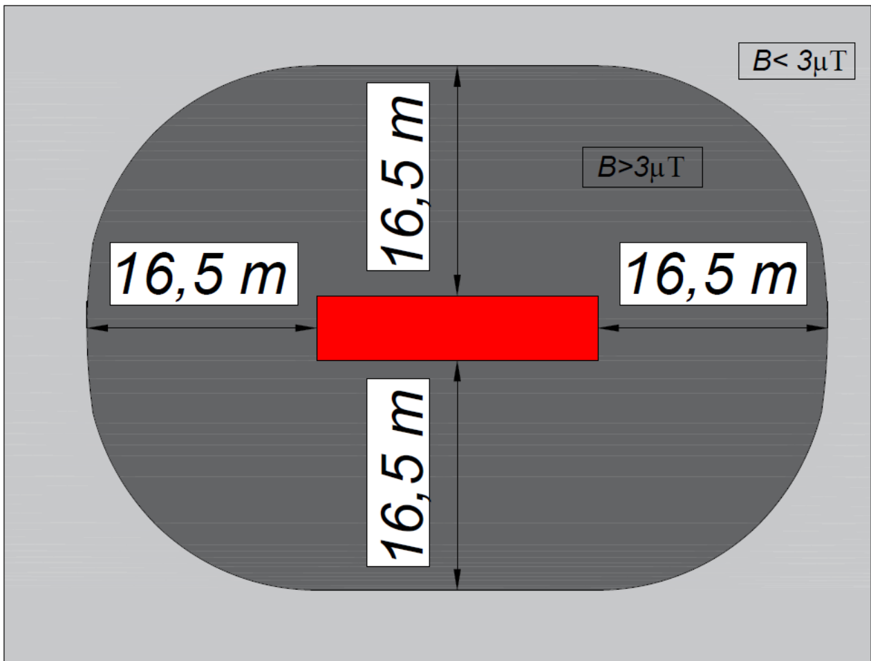
Figura 4: Distanza di prima approssimazione cabina elettrica equipaggiata con trasformatori da 5000 kVA
