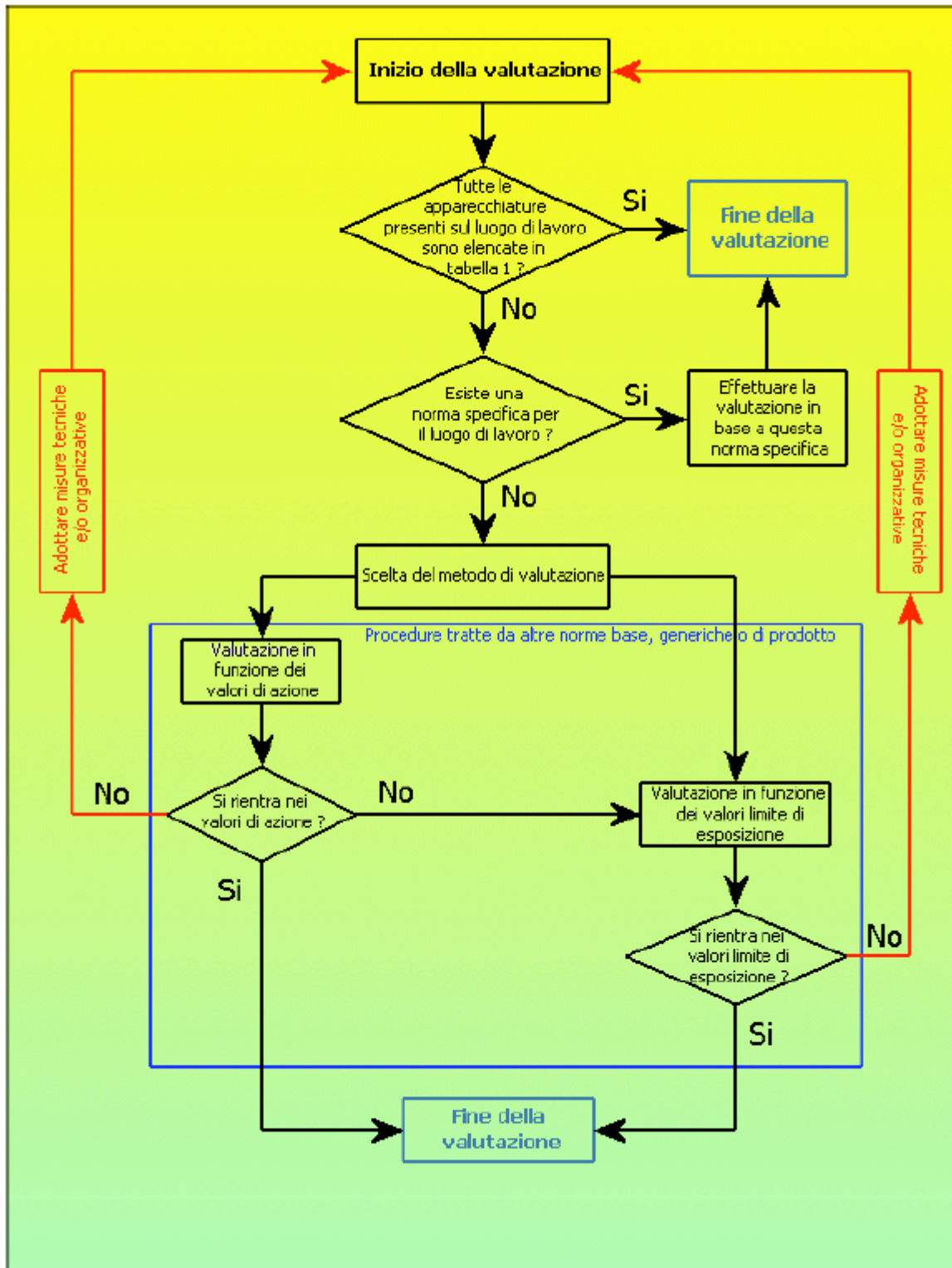
Figura 17: Diagramma di flusso del processo di valutazione del rischio elettromagnetico (CEI EN 50499)
