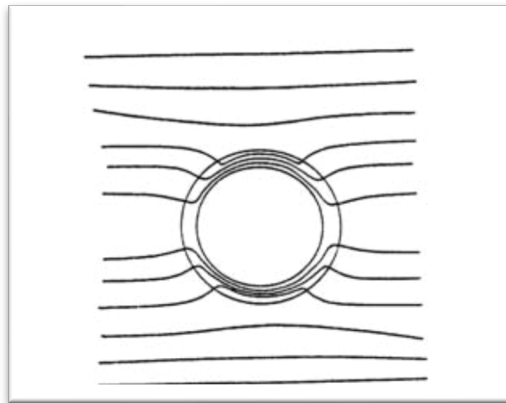
Figura 20: andamento qualitativo della deformazione delle linee di forza di un campo magnetico uniforme per effetto di un nucleo in materiale ferromagnetico
