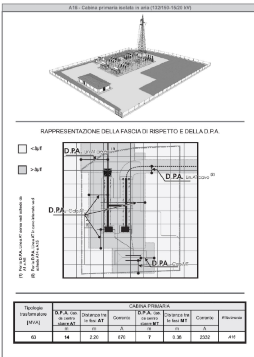
Figura 10: DPA Cabina Primaria AT/MT Enel equipaggiata con n° 2 trasformatori AT/MT da 63 MVA- Linea Guida per l'applicazione del § 5.1.3 dell'Allegato al D.M. 29.05.08 – Distanza di prima approssimazione da linee e cabine elettriche
