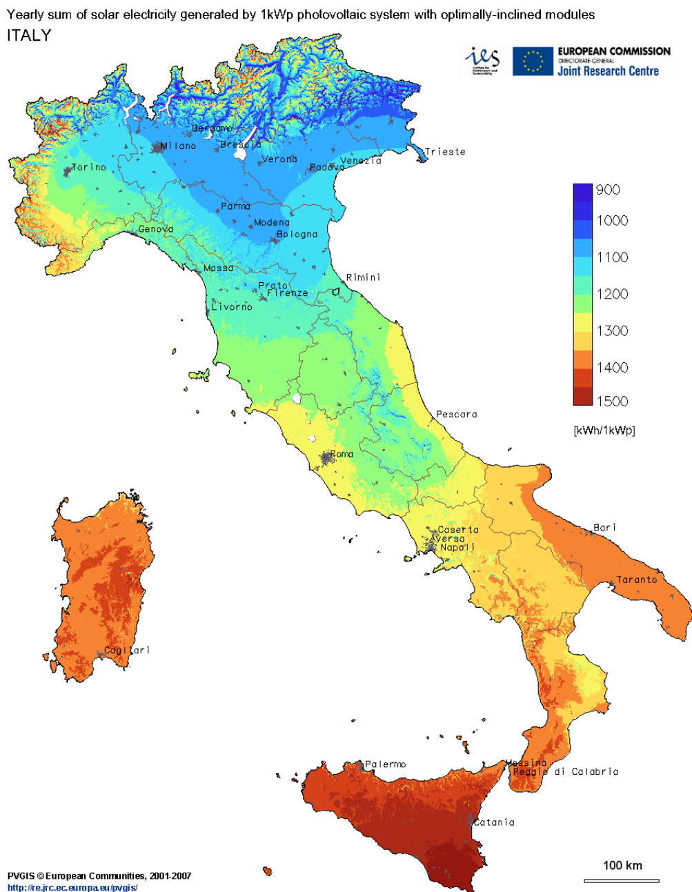
Figura 8 - Valori della Radiazione solare annua (fonte: PVGIS).
