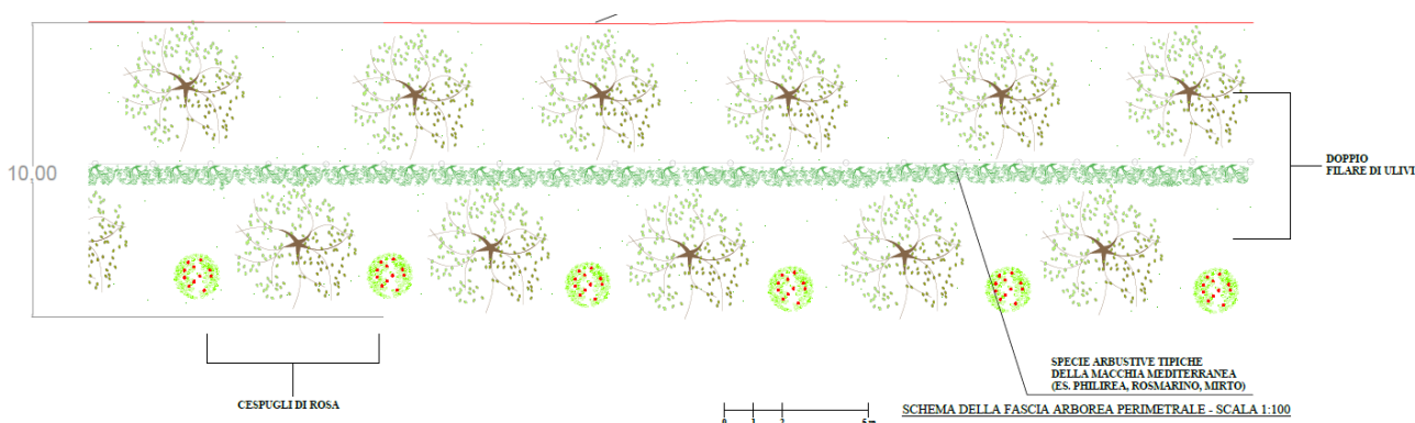
Figura 27 – Schema della fascia di mitigazione ambientale perimetrale
