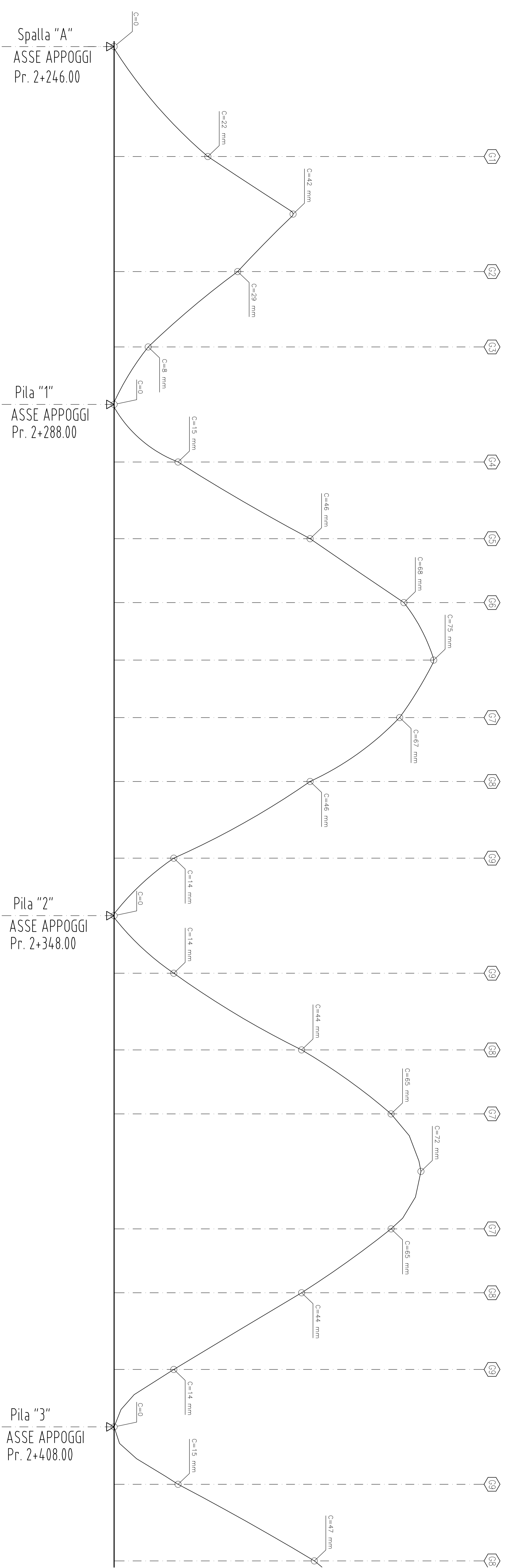
SCHEMA CONTROFRECCE PER DEFORMATA ELASTICA: TRAVE ESTERNO CURVA
