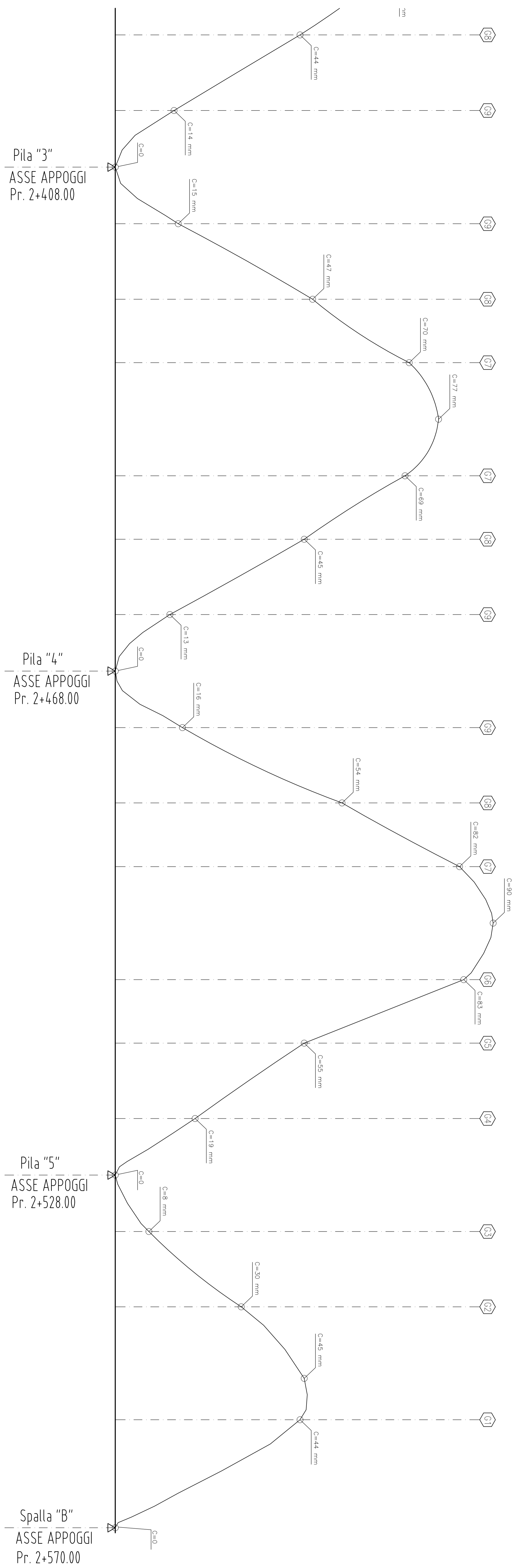
SCHEMA CONTROFRECCE PER DEFORMATA ELASTICA: TRAVE ESTERNO CURVA Scala 1:200
