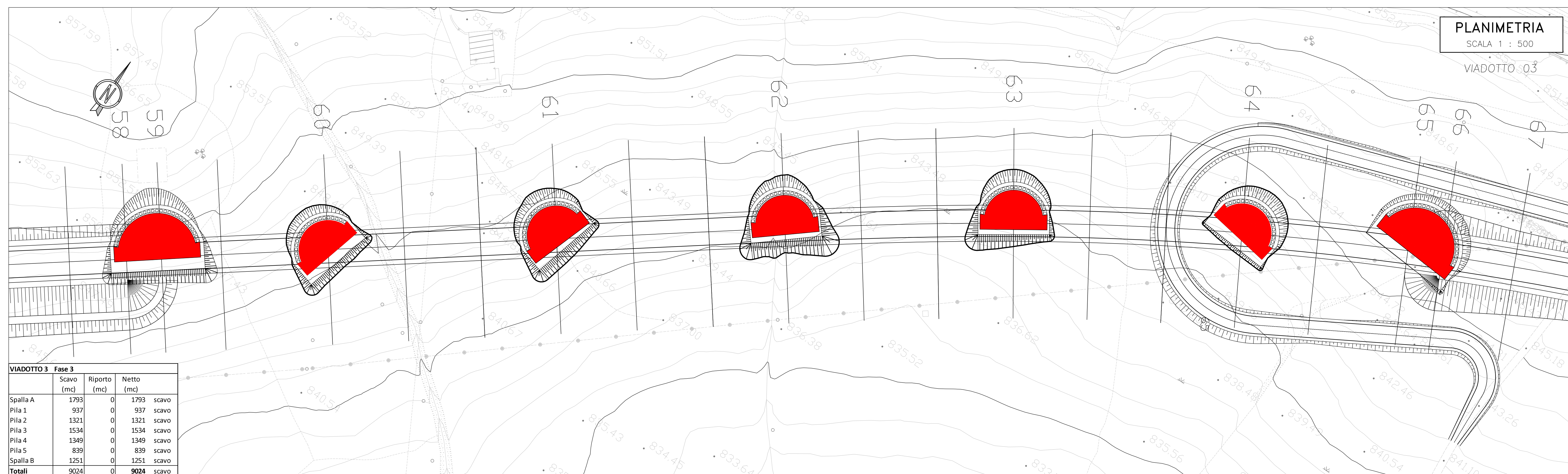
Fase 3: approfondimento scavo per realizzazione tiranti
