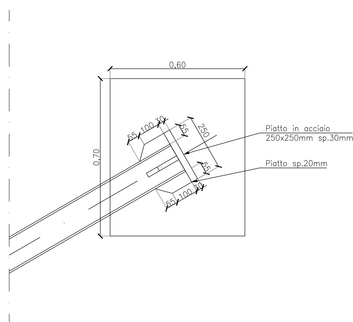
DETTAGLIO SCALA 1 : 10
