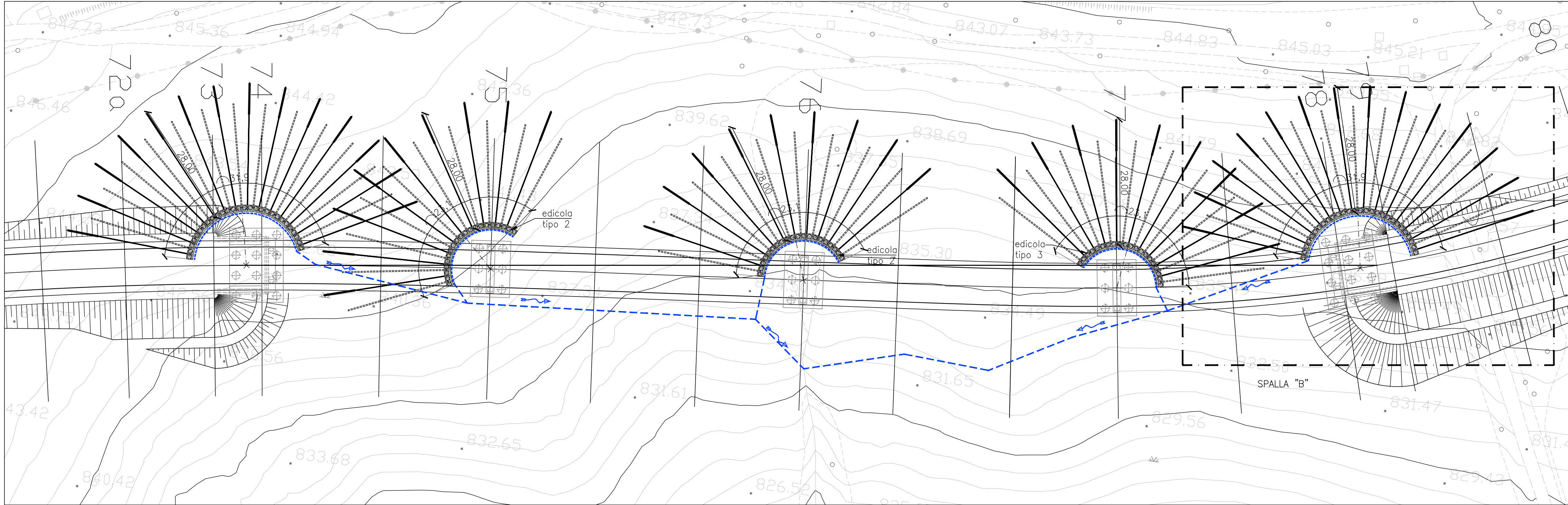
PLANIMETRIA SCALA 1 : 500
