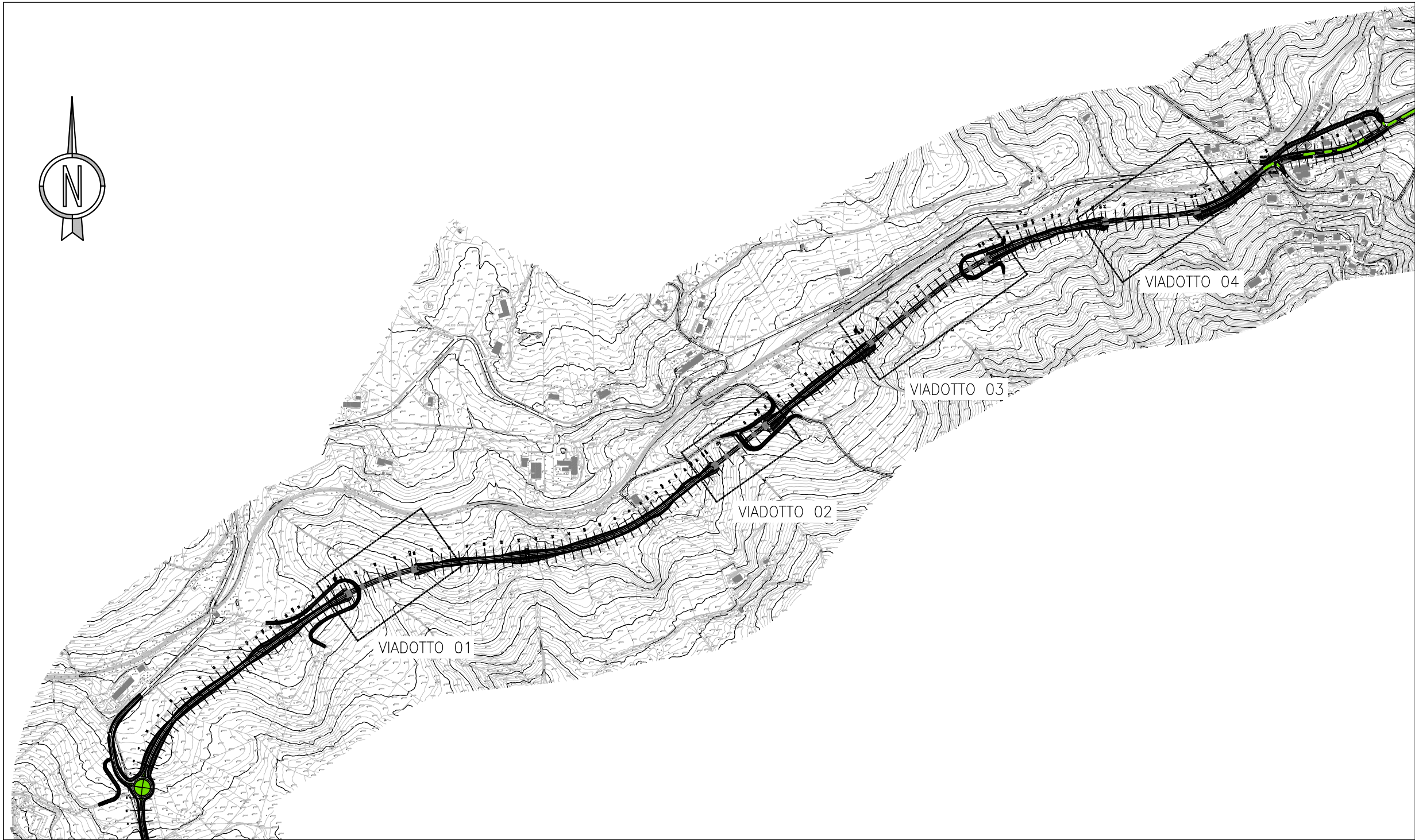
KEYPLAN SCALA 1 : 10000
