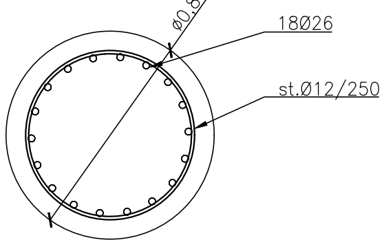
ARMATURA PALI SCALA 1 : 20
