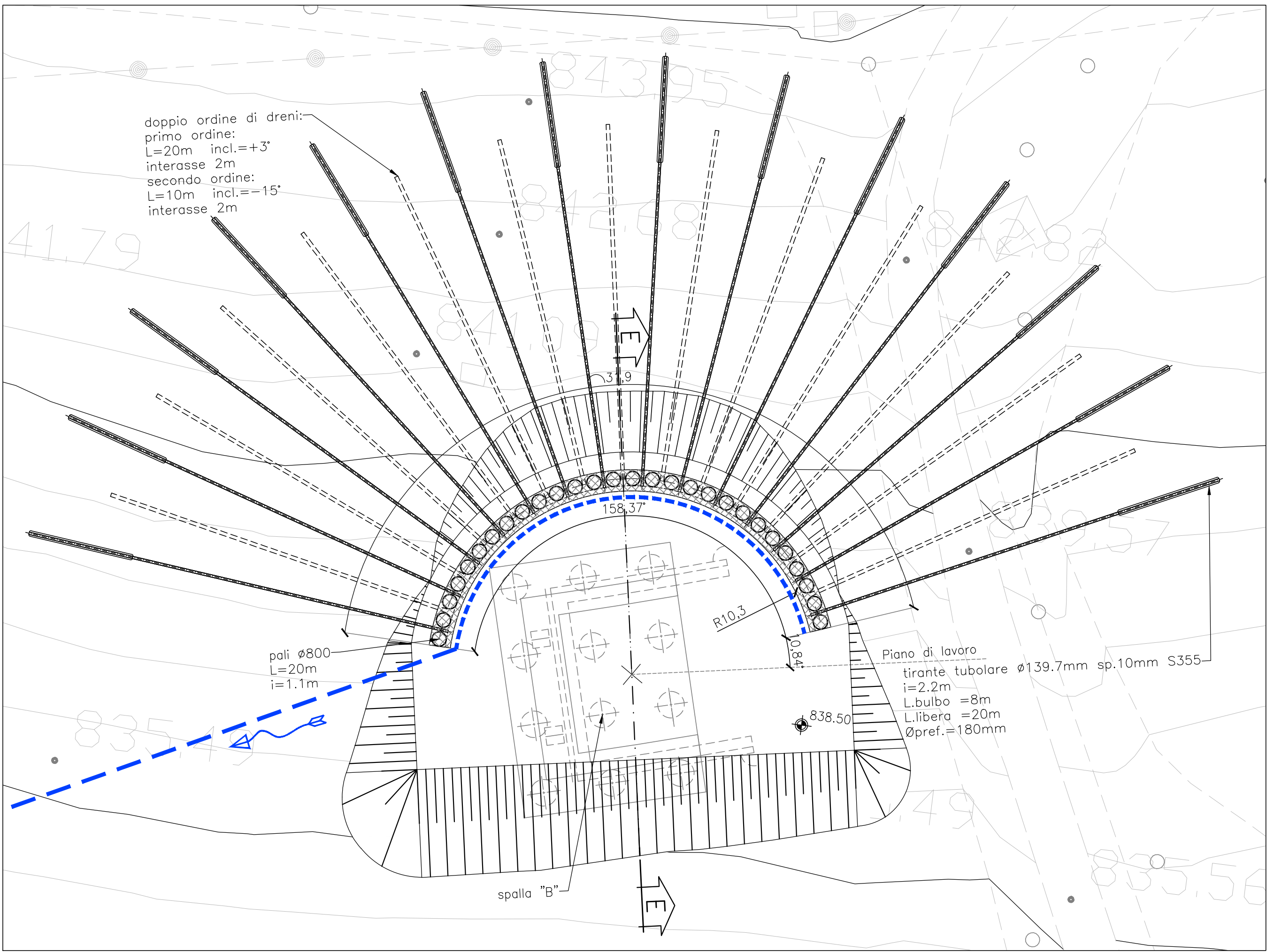
PIANTA SCALA 1 : 200
