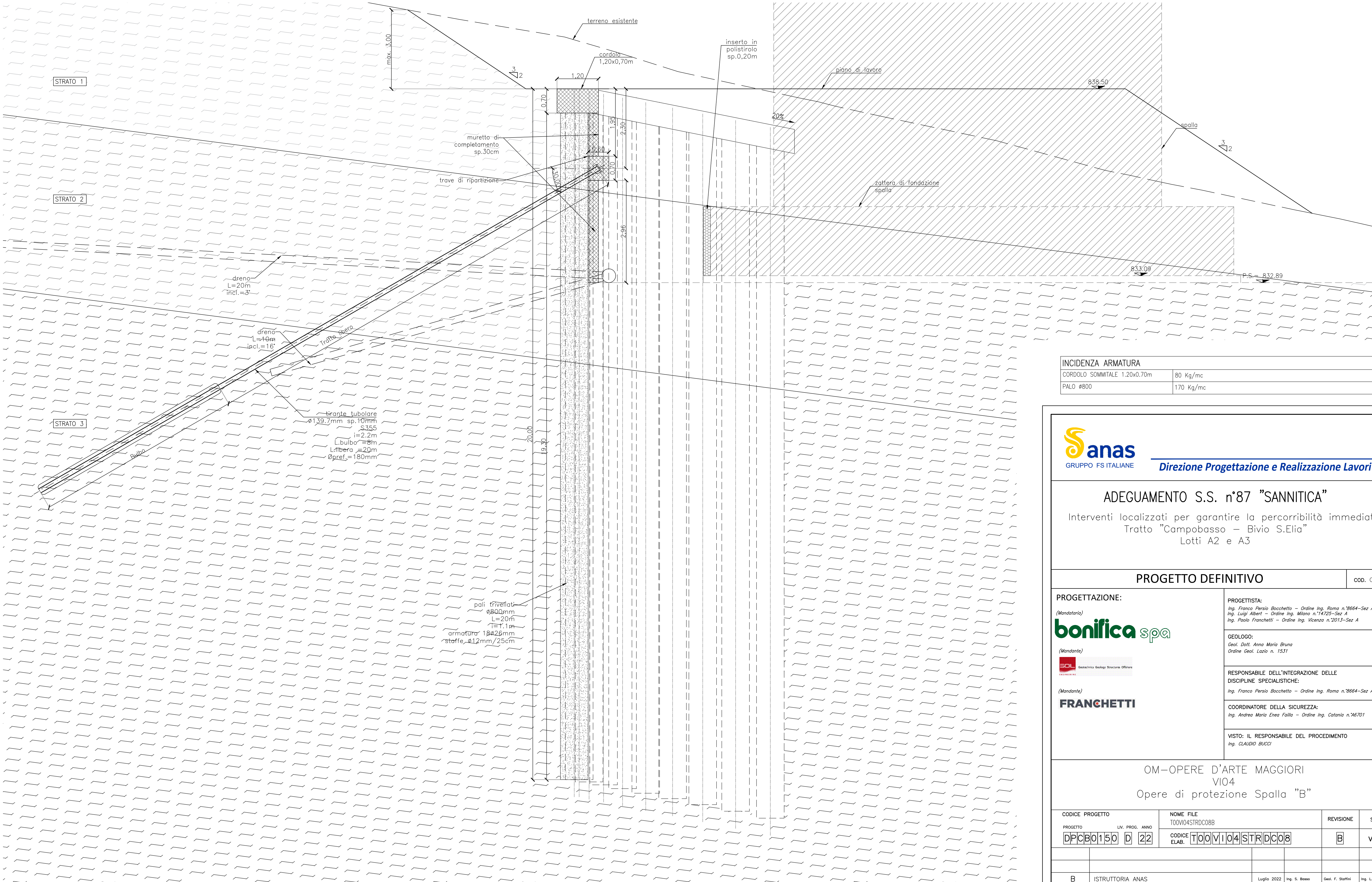
SEZIONE E-E SCALA 1 : 50
