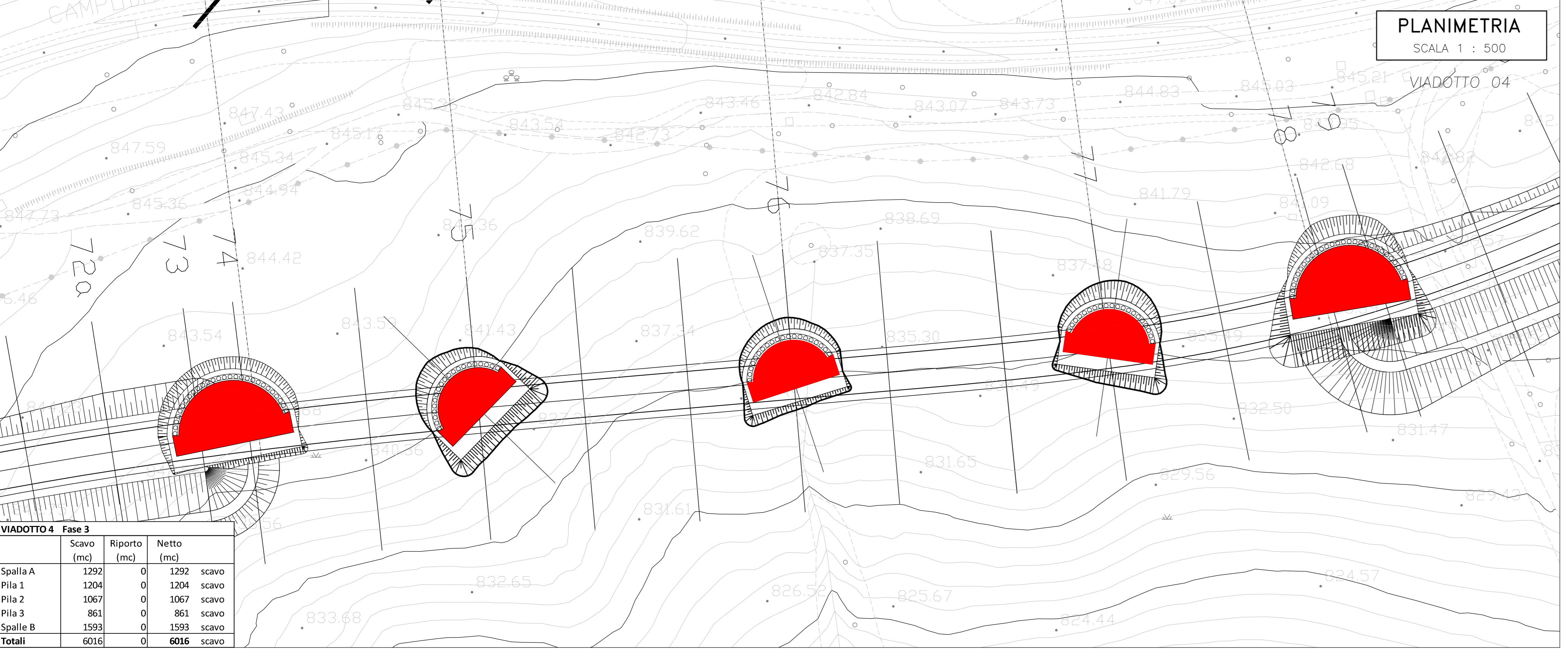
Fase 3: approfondimento scavo per realizzazione tiranti
