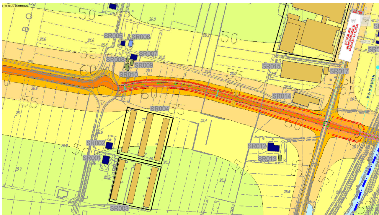
FIGURA 8.3-1 – DETTAGLIO DELLA MAPPATURA DELLE ISOFONICHE DIURNE CON OPERE DI MITIGAZIONE IN CORRISPONDENZA DEI RICEVITORI SR005, SR006 E SR007
