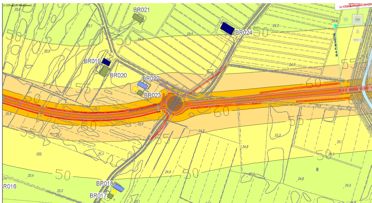
FIGURA 6.5-2 – PARTICOLARE DELLA MAPPATURA DELLE ISOFONICHE IN ADIACENZA AL RICETTORE BR022
