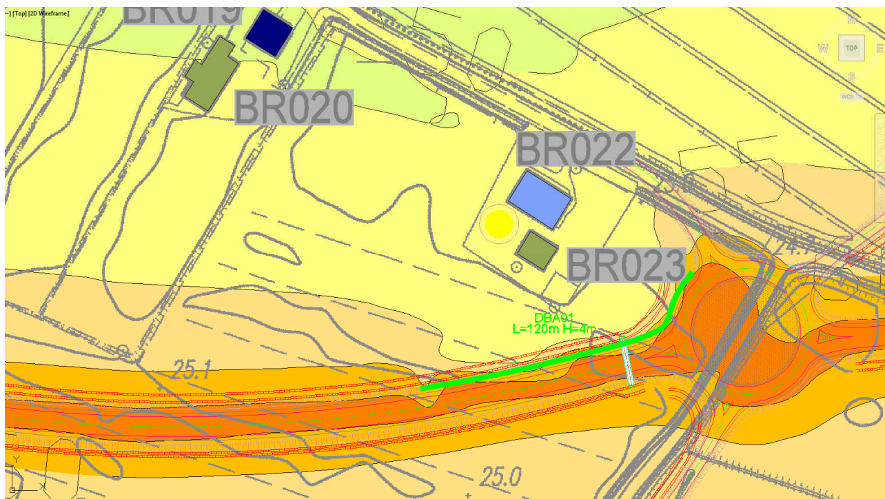
FIGURA 8.3-2 – DETTAGLIO DELLA MAPPATURA DELLE ISOFONICHE DIURNE CON OPERE DI MITIGAZIONE IN CORRISPONDENZA DEL RICEUTORE BR022
