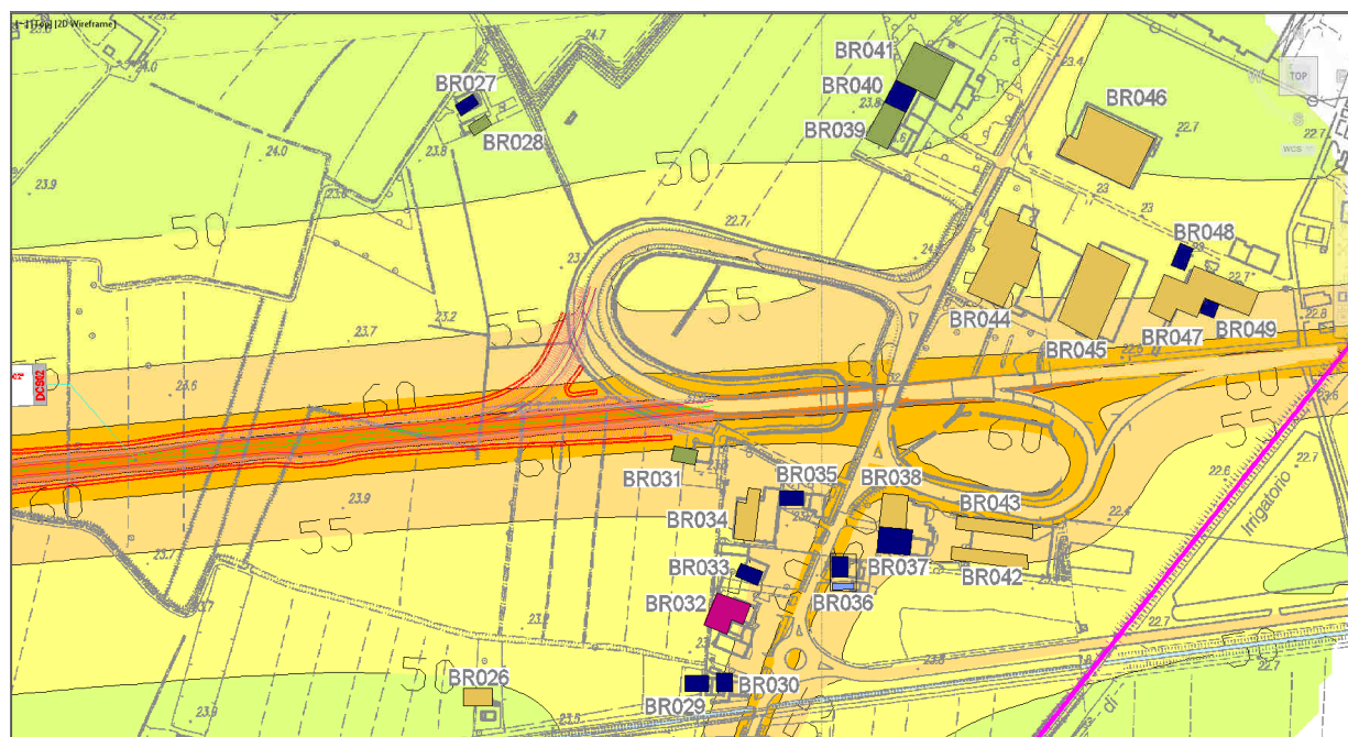
FIGURA 6.5-3 – PARTICOLARE DELLA MAPPATURA DELLE ISOFONICHE IN ADIACENZA AI RICETTORI BR035-BR037 E BR 049
