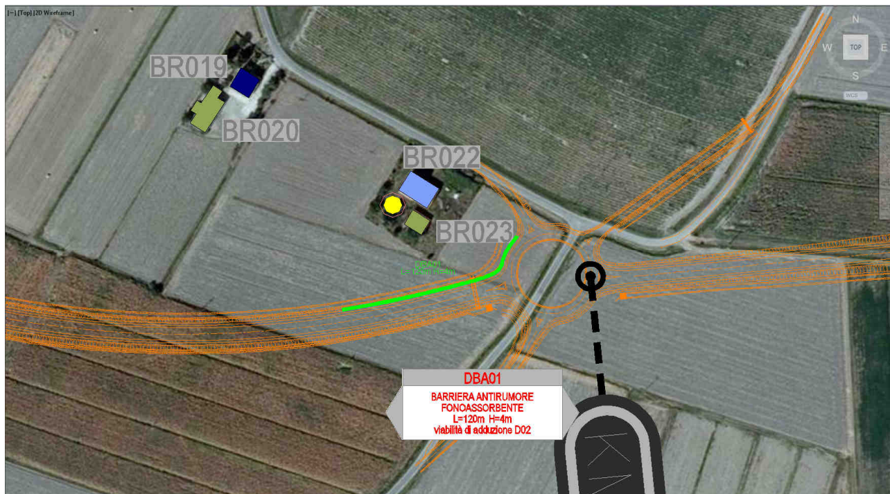
FIGURA 7.3-2 – LOCALIZZAZIONE ED ESTENSIONE DELLA BARRIERA ACUSTICA PREVISTA IN ADIACENZA AL RICETTORE BR022
