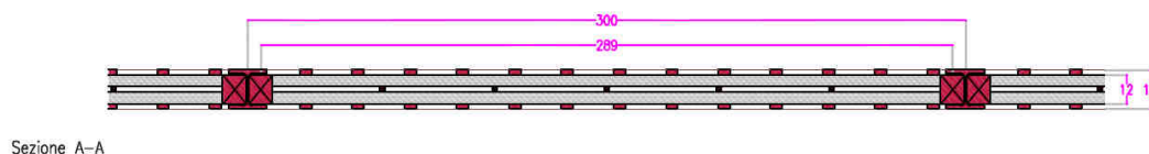
FIGURA 7.2-2 – SEZIONE ORIZZONTALE DELLA BARRIERA ACUSTICA IN LEGNO
