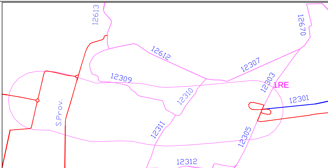
FIGURA 5.3-1 – GRAFO STRADALE STATO DI FATTO – ZONA VIABILITÀ DI ADDUZIONE “D02”
