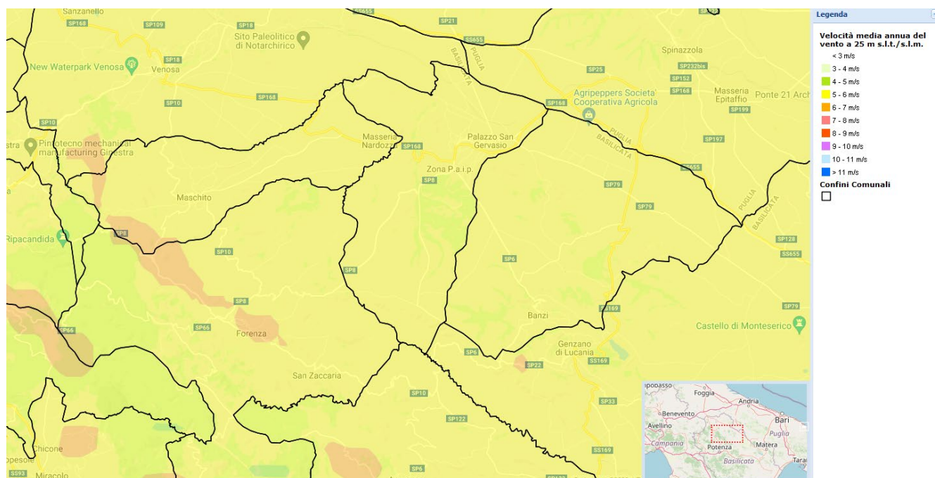
Figura 4 – Velocità media annua del vento a 25 metri.
