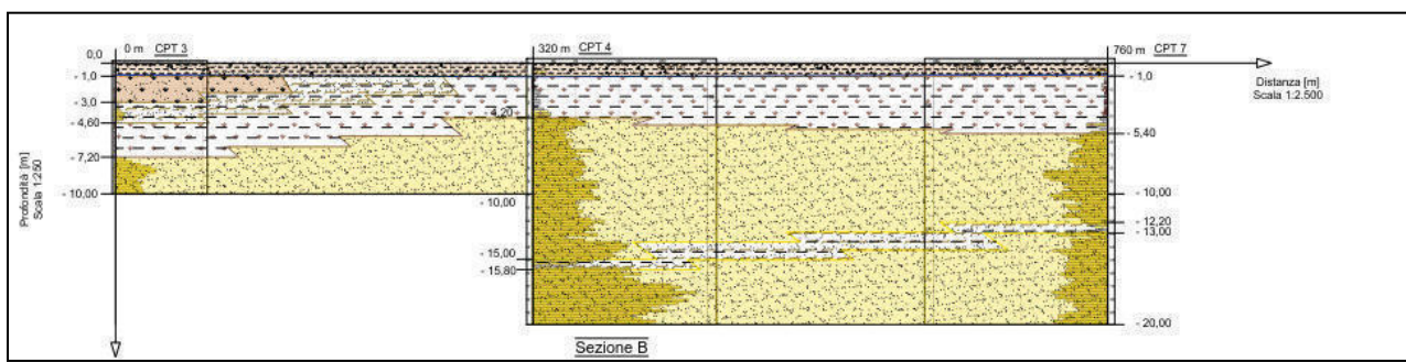
Fig.12: Sezione stratigrafica tra le CPT 3, CPT4 e CPT 7
