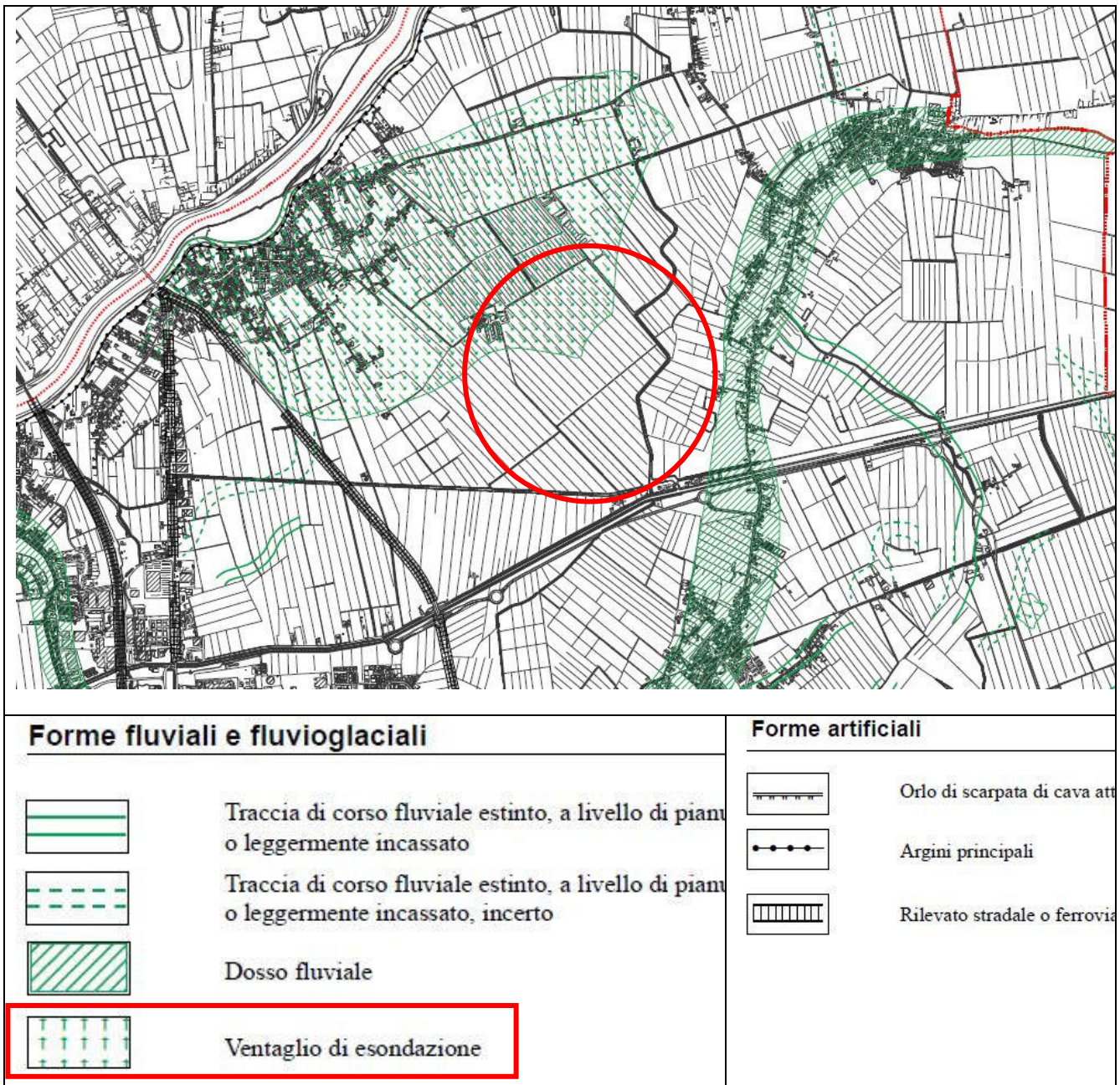
Figura 6: Estratto della Carta geomorfologica del PAT del Comune di Rovigo
