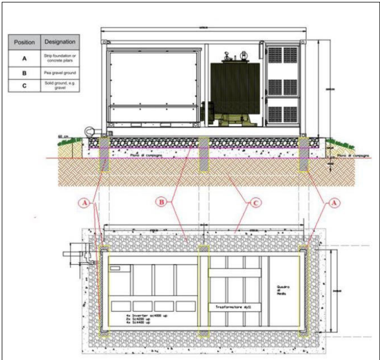
Figura 24: Particolare cabina/piano di campagna e particolare dei supporti della cabina.
