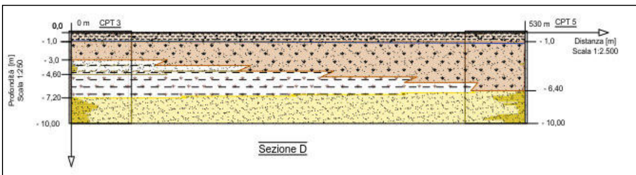
Fig.13: Sezione stratigrafica tra le CPT 3, CPT 5
