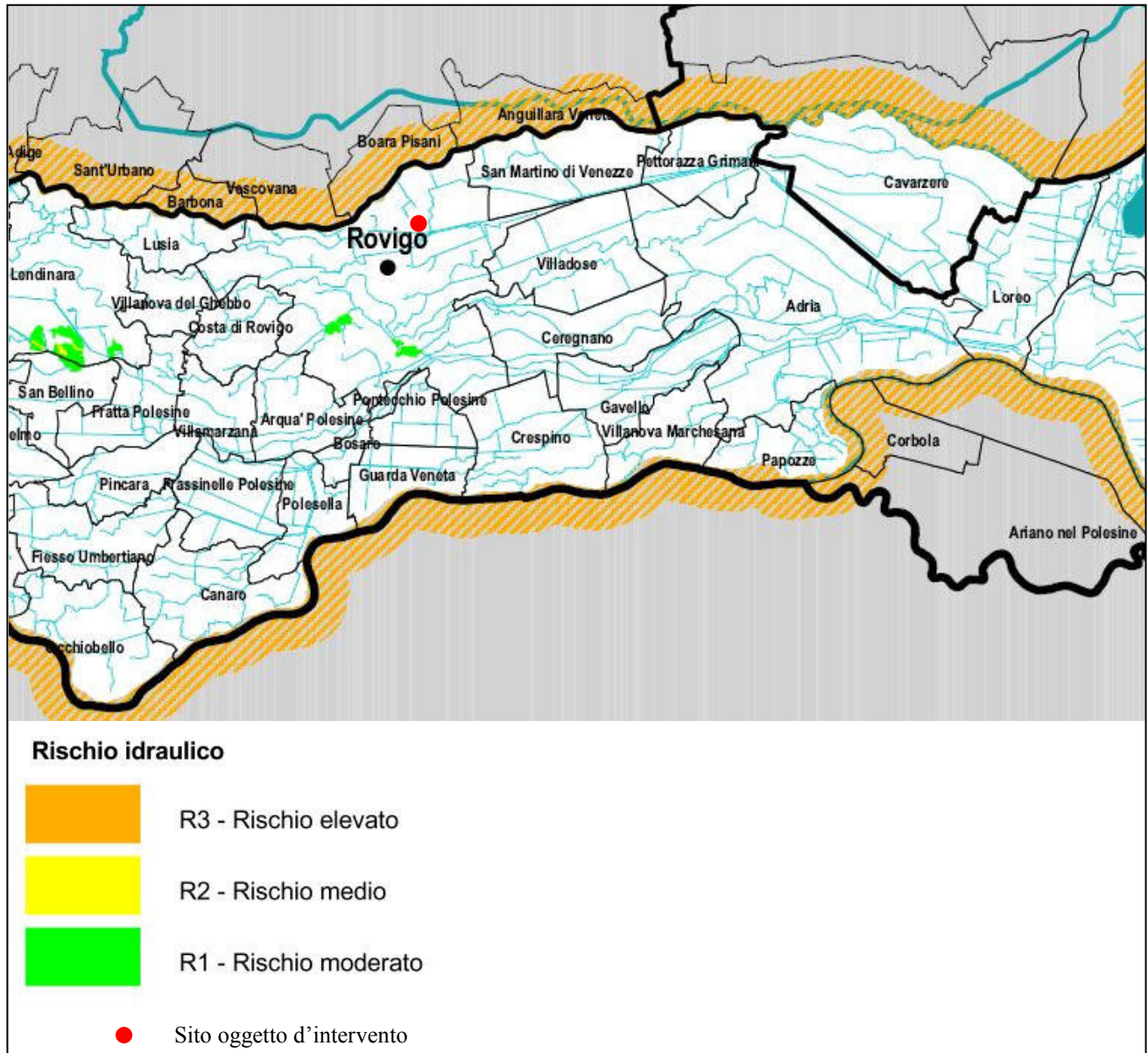
Figura 18: Estratto della Carta di Rischio Idraulico dell' Autorità di Bacino dei Fiumi Fissero-Tartaro-Canalbianco
