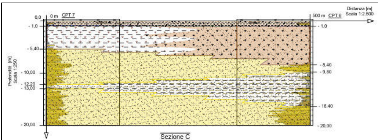
Fig.12: Sezione stratigrafica tra le CPT 7, CPT6
