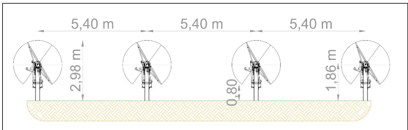
Figura 22: Interasse moduli FVT
