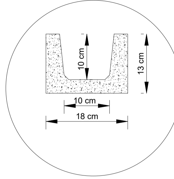
DETTAGLIO CANALETTA PASSA - CAVI SCALA 1:10
