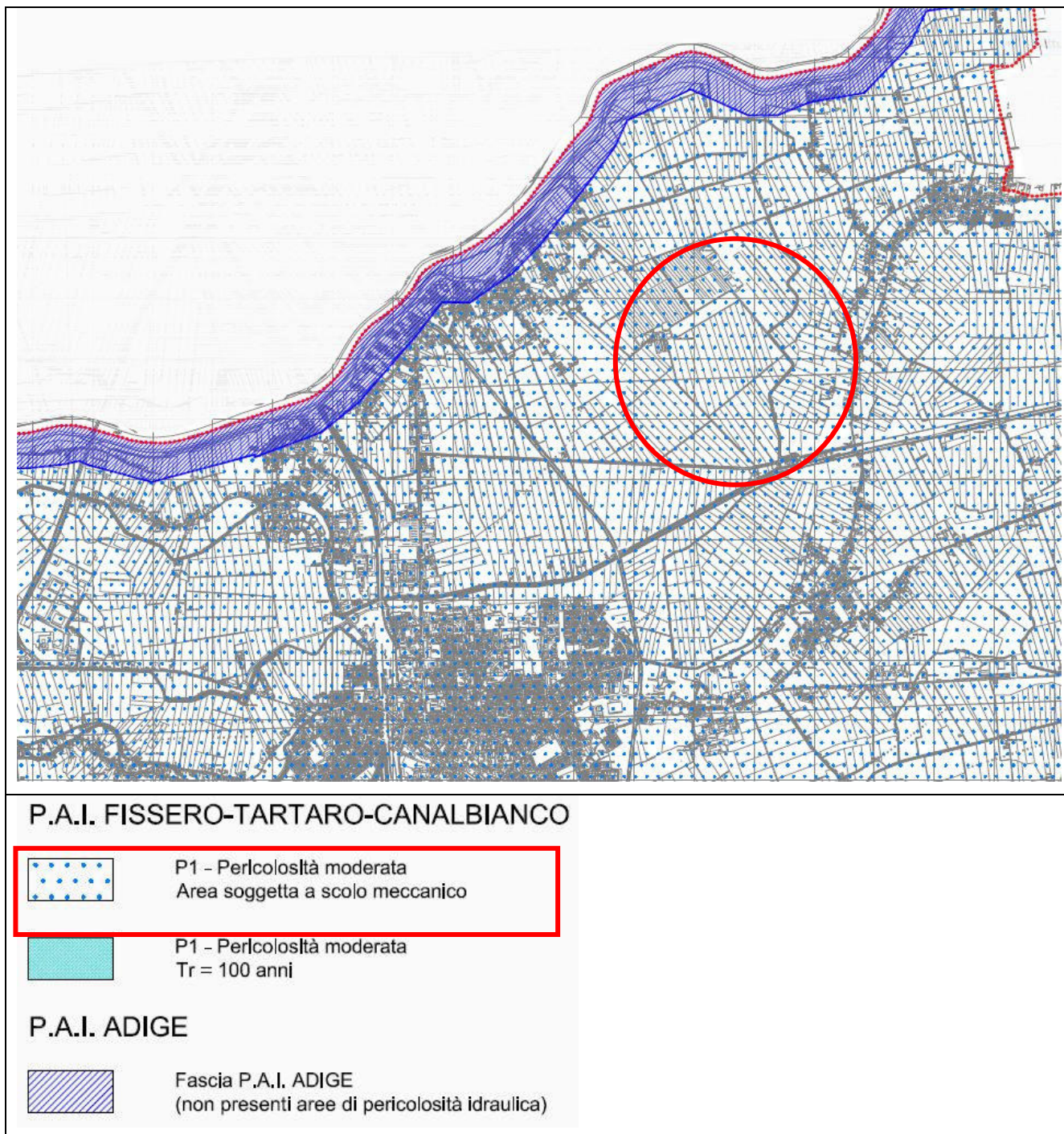
Figura 17: Estratto della Carta di Pericolosità Idraulica dell'Autorità di Bacino dei Fiumi Fissero-Tartaro-Canalbianco
