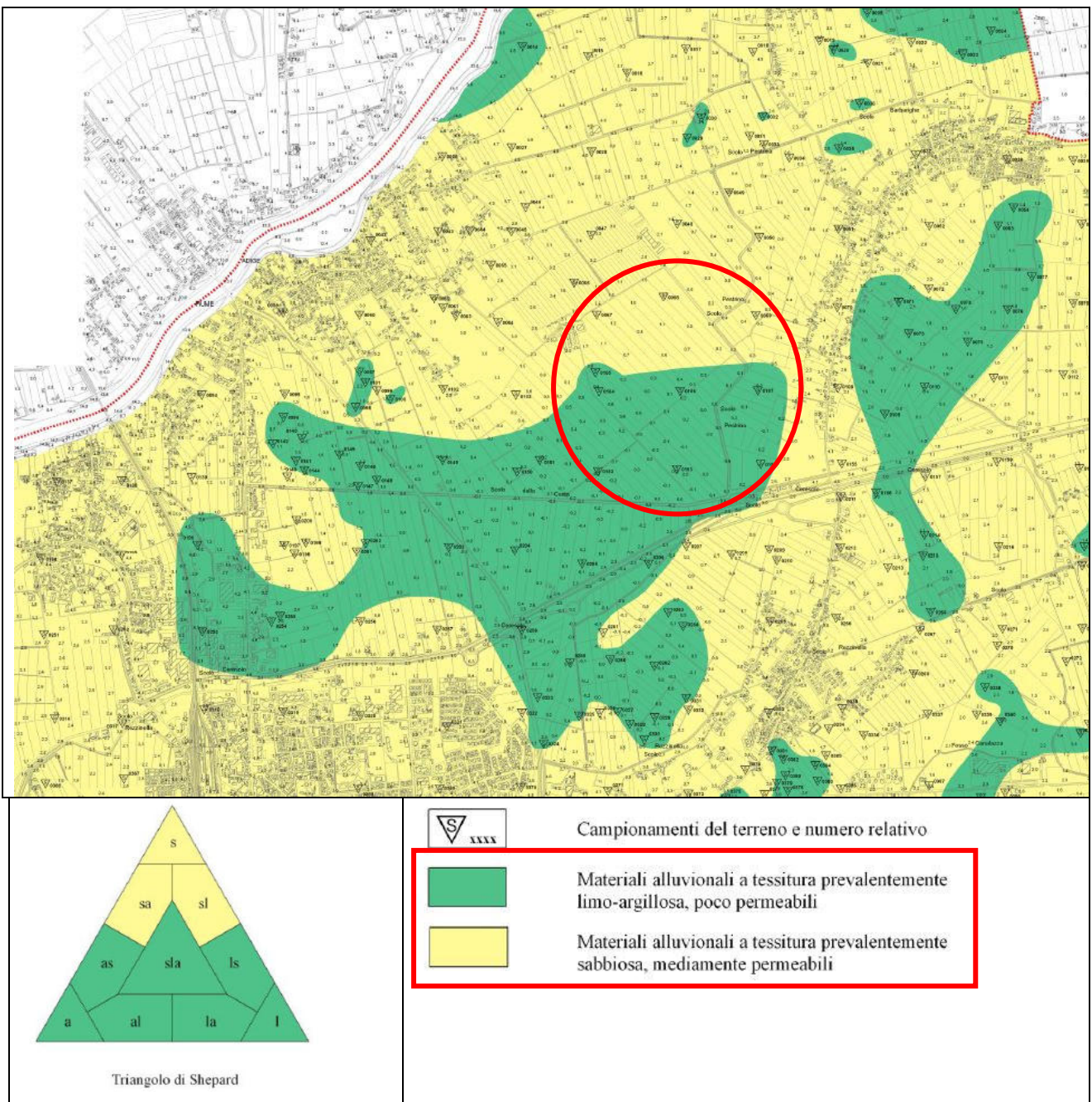
Figura 7: Estratto della Carta Litologica del PAT del Comune di Rovigo
