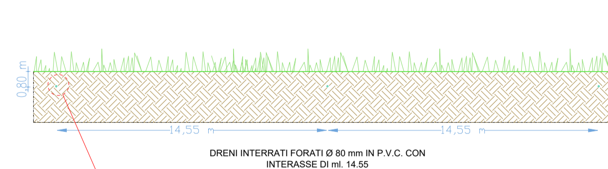
DETTAGLIO DRENO SCALA 1:50
