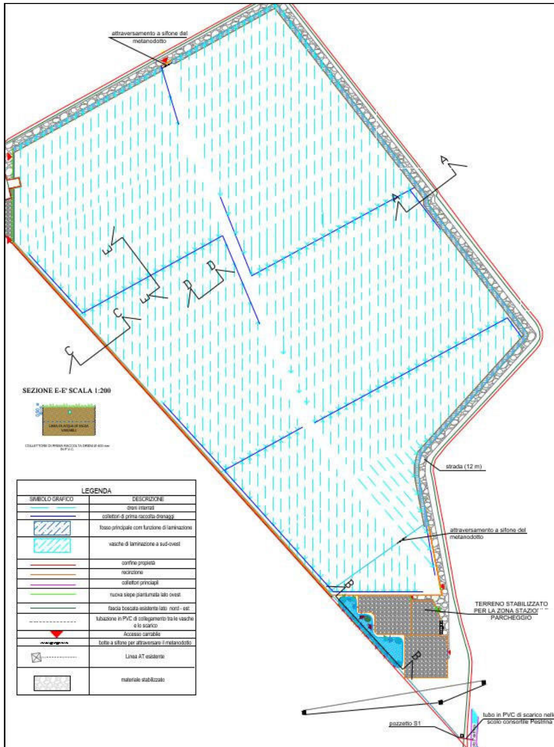
Figura 21: Planimetria di progetto dell'impianto FTV ( estratto da Tav. n.14 "schema rete di deflusso e drenaggio acque meteoriche-stato di progetto" in allegato)
