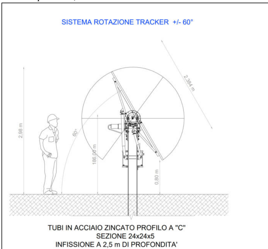
Figura 23: Modulo monoassiale impianto FTV
