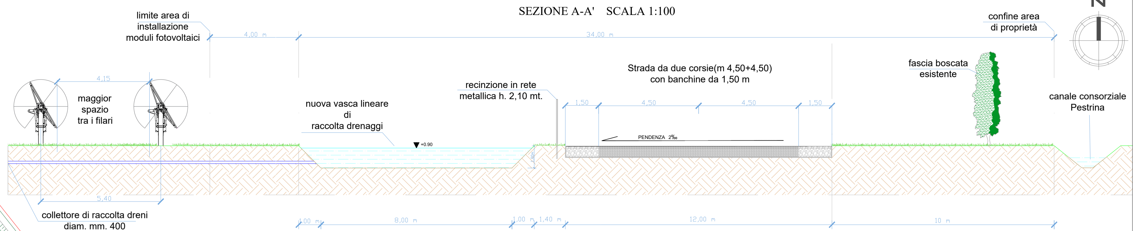
SEZIONE A-A' SCALA 1:100
