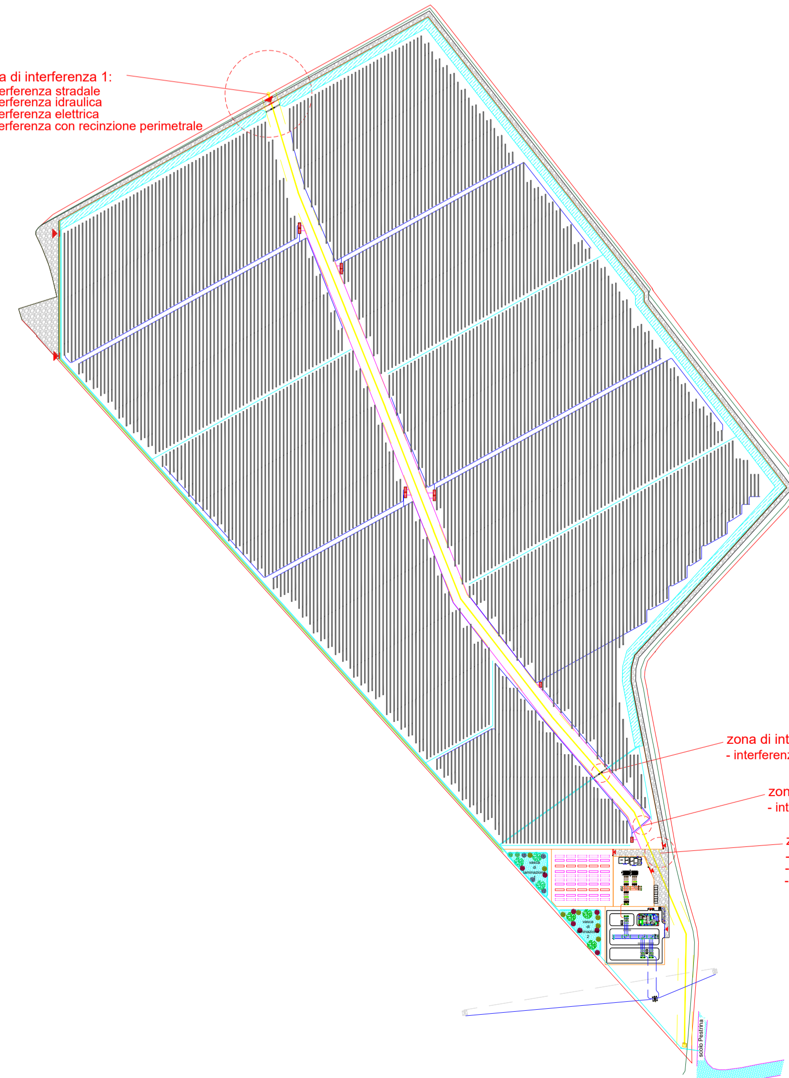
PLANIMETRIA DELL'IMPIANTO - SCALA 1:5.000
