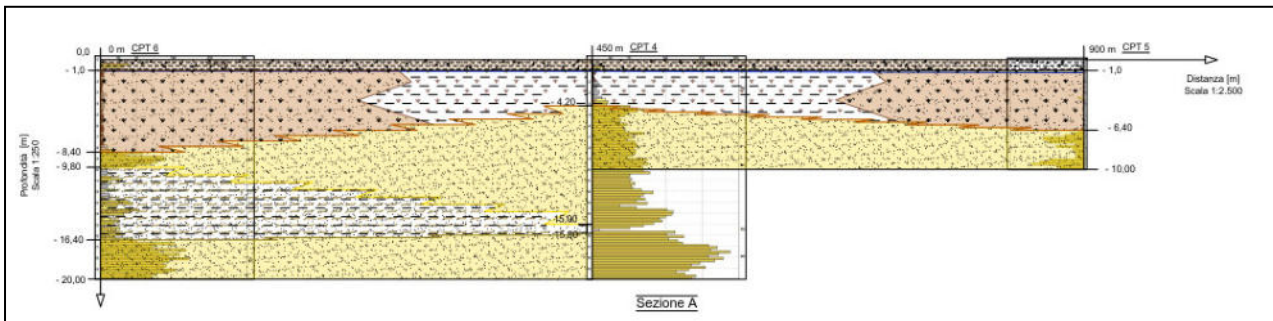
Fig.10: Sezione stratigrafica tra le CPT 6, CPT4 e CPT 5
