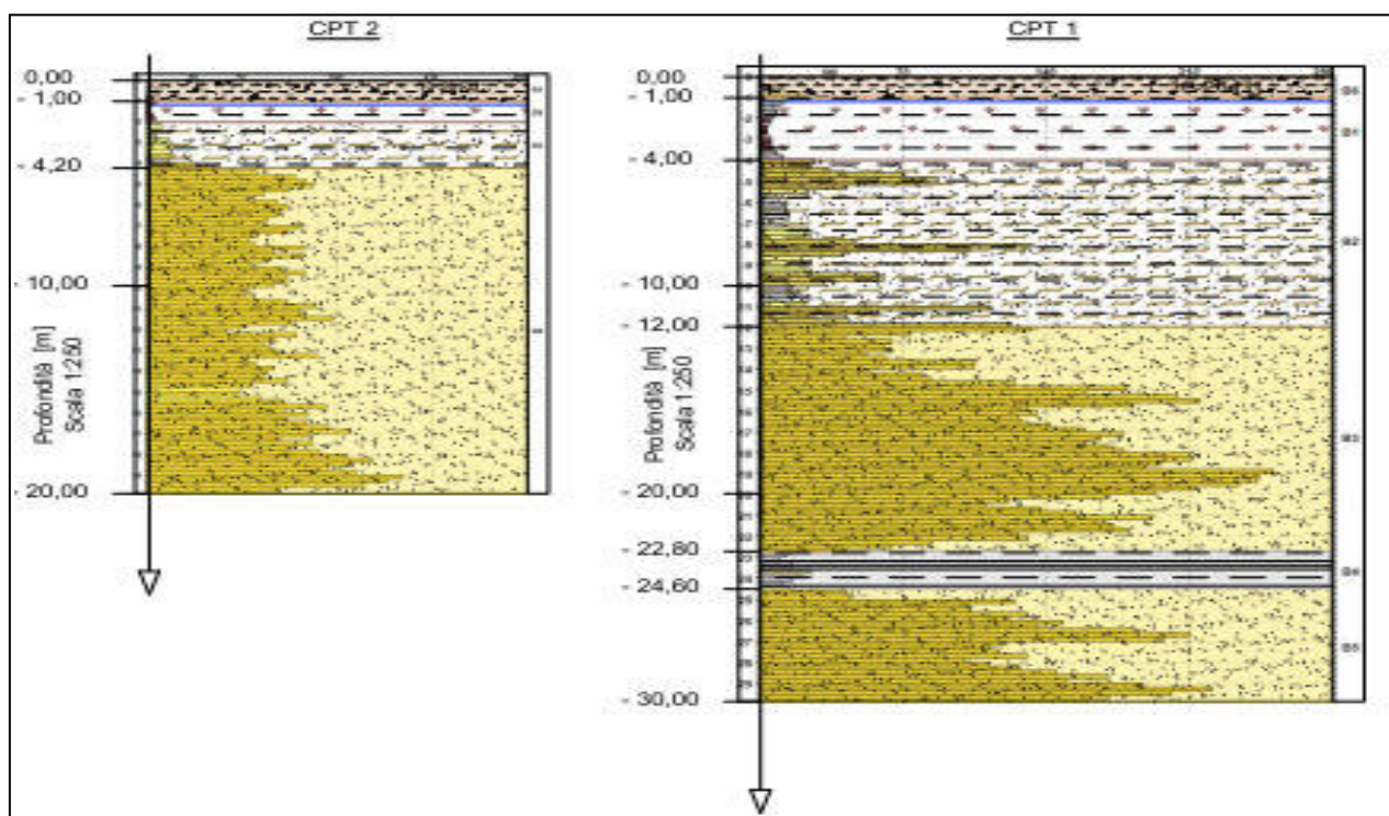
Fig.14: Sezione stratigrafica CPT 2, CPT1
