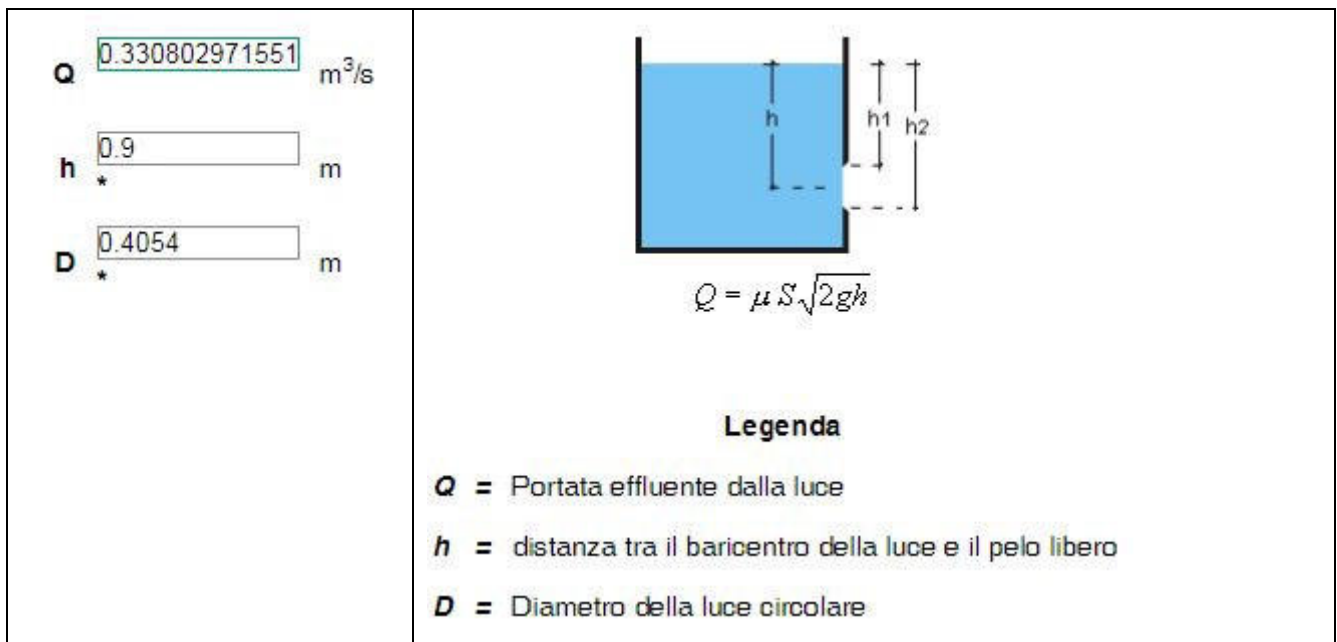
Figura 25 – Calcolo diametro tubo e schema pozzetto di scarico
