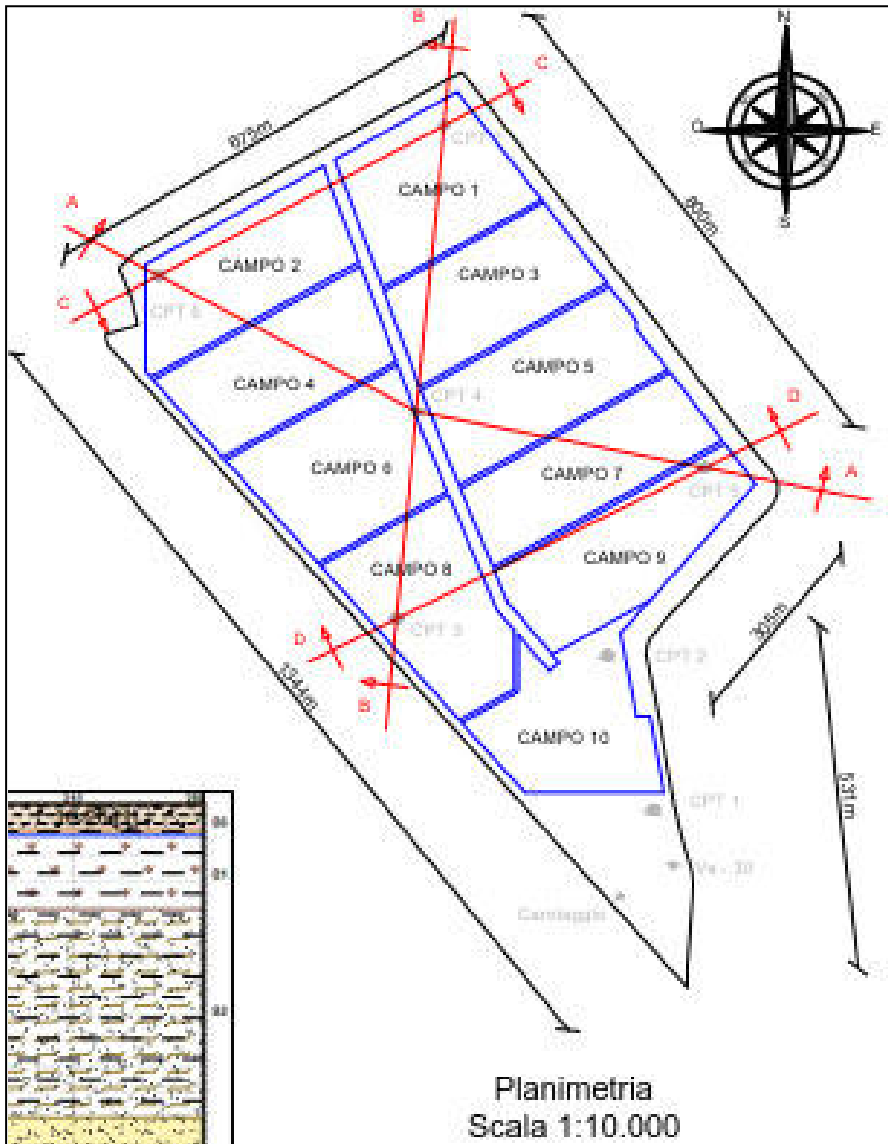
Fig.9: Estratto planimetrico con tracciate le sezioni stratigrafiche
