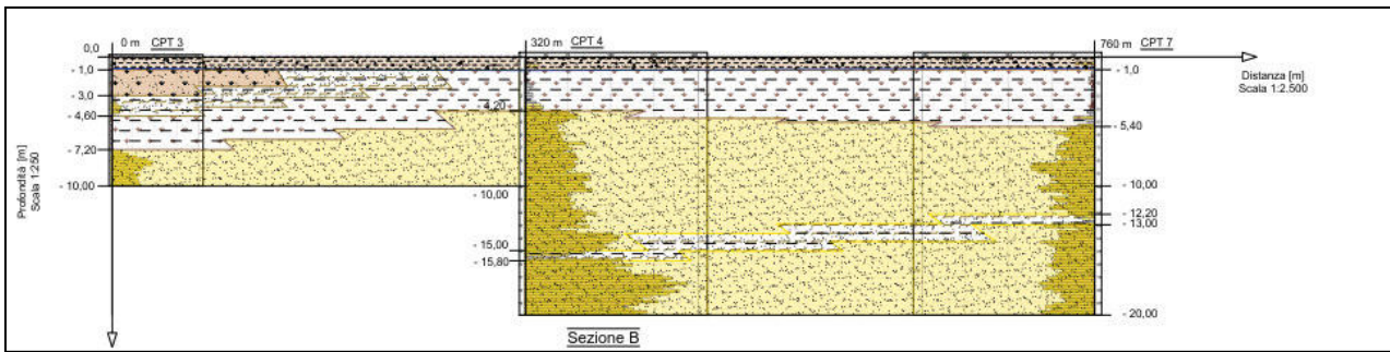
Fig.11: Sezione stratigrafica tra le CPT 3, CPT4 e CPT 7
