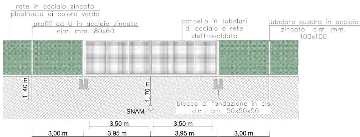
Figura 12: attraversamento della fascia di rispetto con la recinzione e cancello di accesso nella zona 1.
