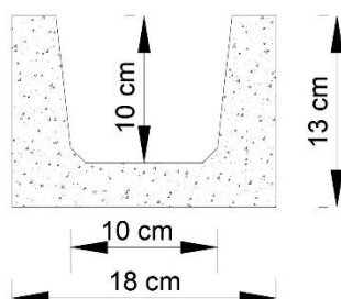
Figura 10: dettaglio canaletta passa - cavi.
