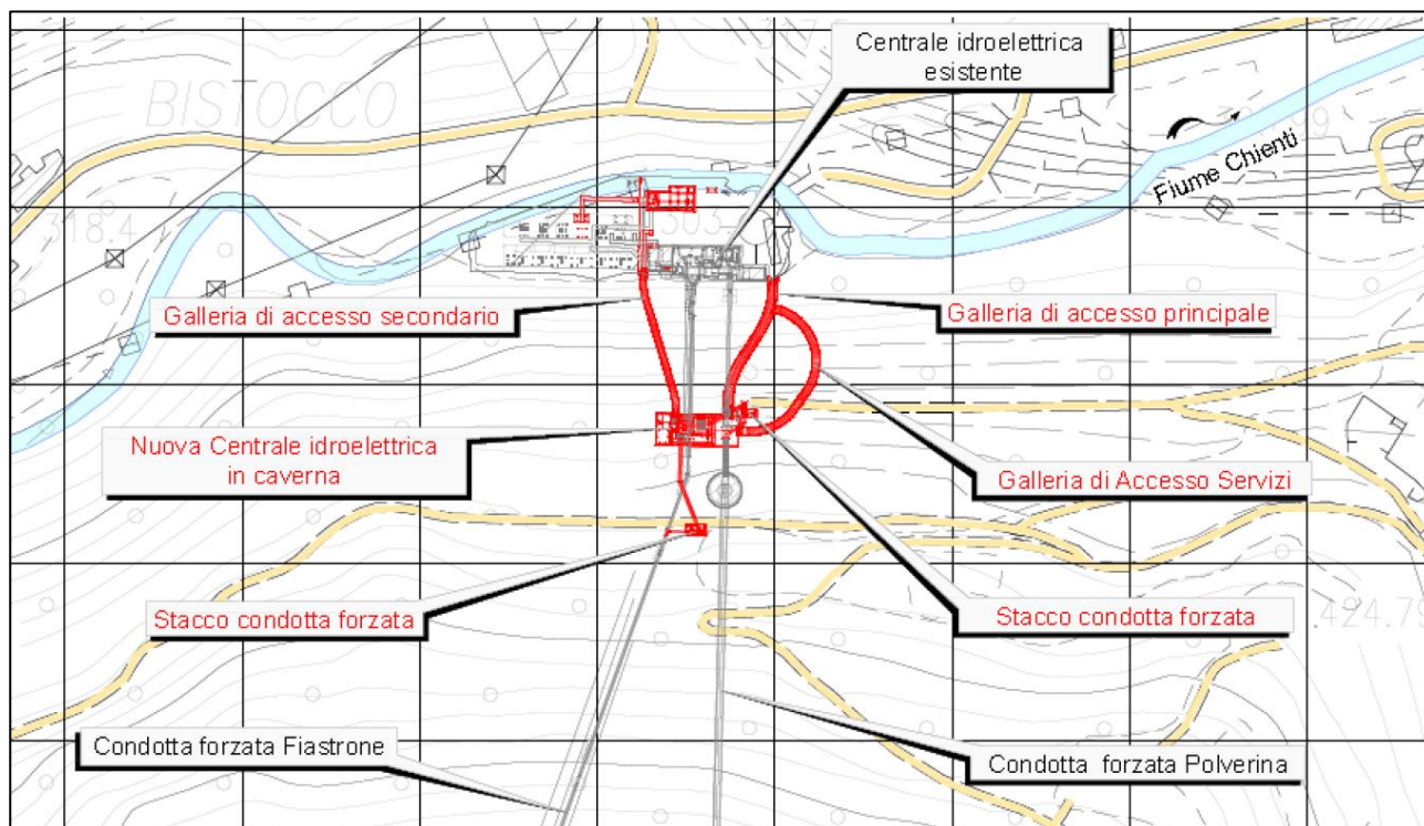
Figura 2: area di intervento centrale esistente
