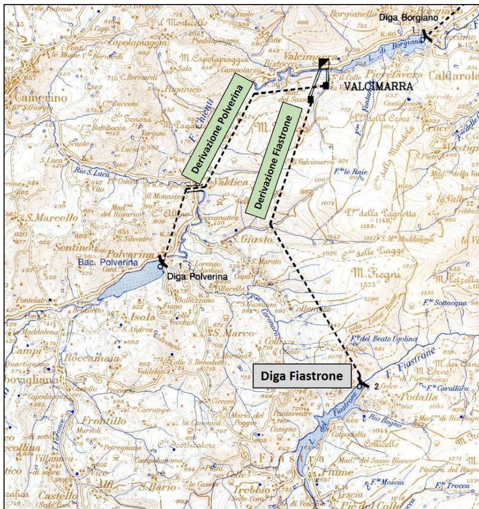
Figura 9: impianto di Valcimarra Chienti - Schema idraulico
