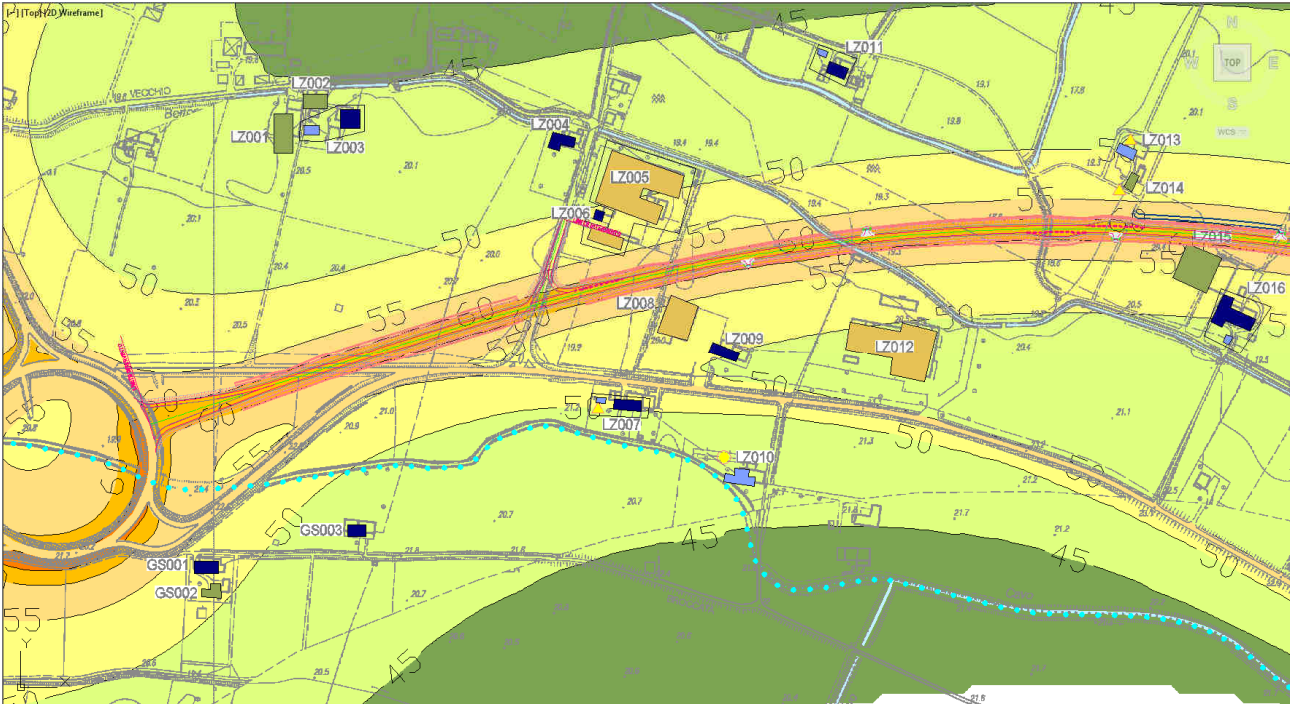
FIGURA 8.3-1 – DETTAGLIO DELLA MAPPATURA DELLE ISOFONICHE IN CORRISPONDENZA DEI RICETTORI LZ006 E LZ016
