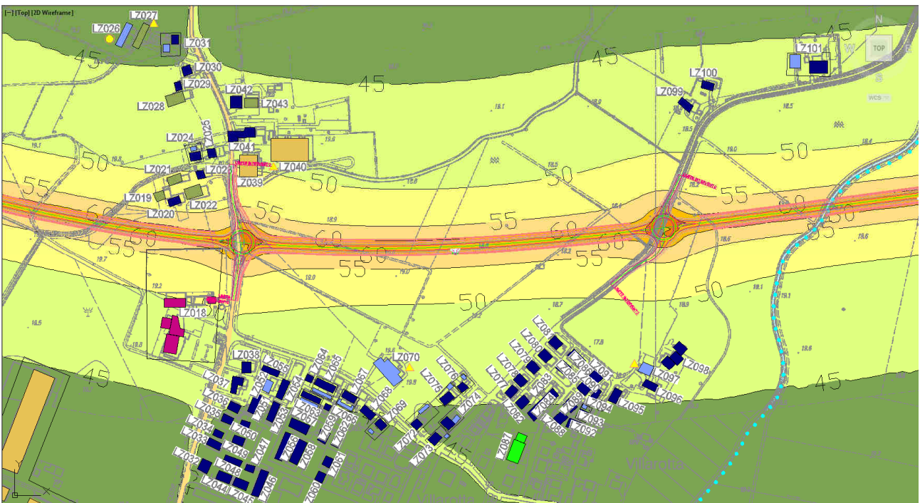
FIGURA 8.3-2 – DETTAGLIO DELLA MAPPATURA DELLE ISOFONICHE IN CORRISPONDENZA DEL RICETTORE LZ020
