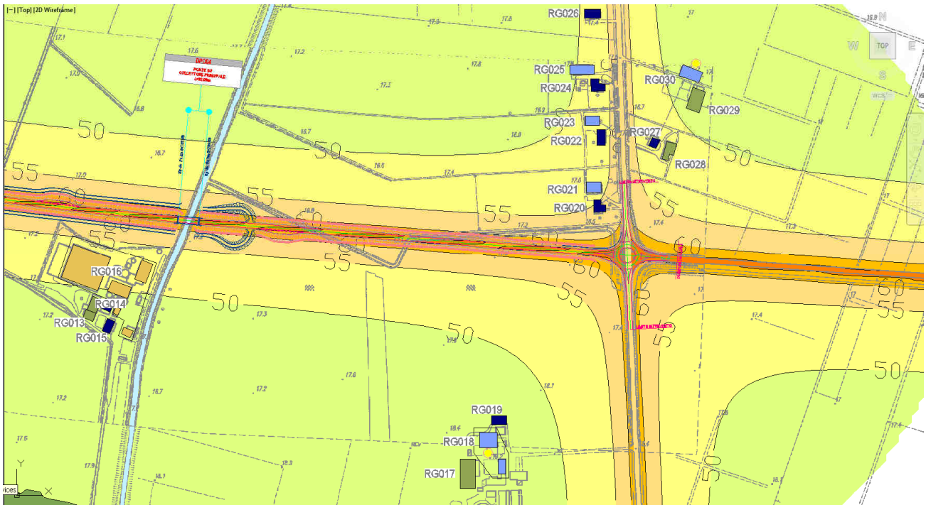
FIGURA 6.5-3 – PARTICOLARE DELLA MAPPATURA DELLE ISOFONICHE NEL TRATTO FINALE DELL'OPERA DI ADDUZIONE D03
