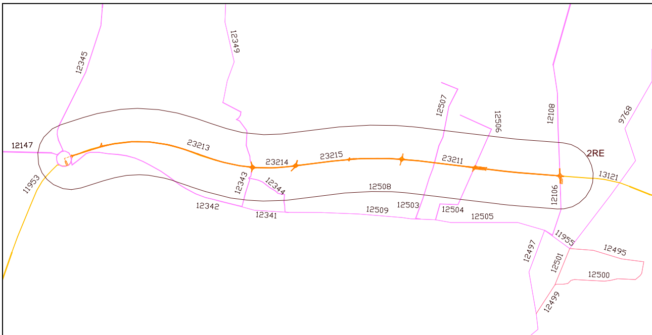
FIGURA 6.3-1 – GRAFO STRADALE – ZONA VIABILITÀ DI ADDUZIONE D03
