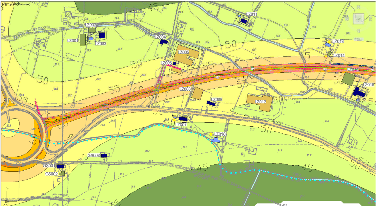
FIGURA 6.5-1 – PARTICOLARE DELLA MAPPATURA DELLE ISOFONICHE NEL TRATTO INIZIALE DELL'OPERA DI ADDUZIONE D03
