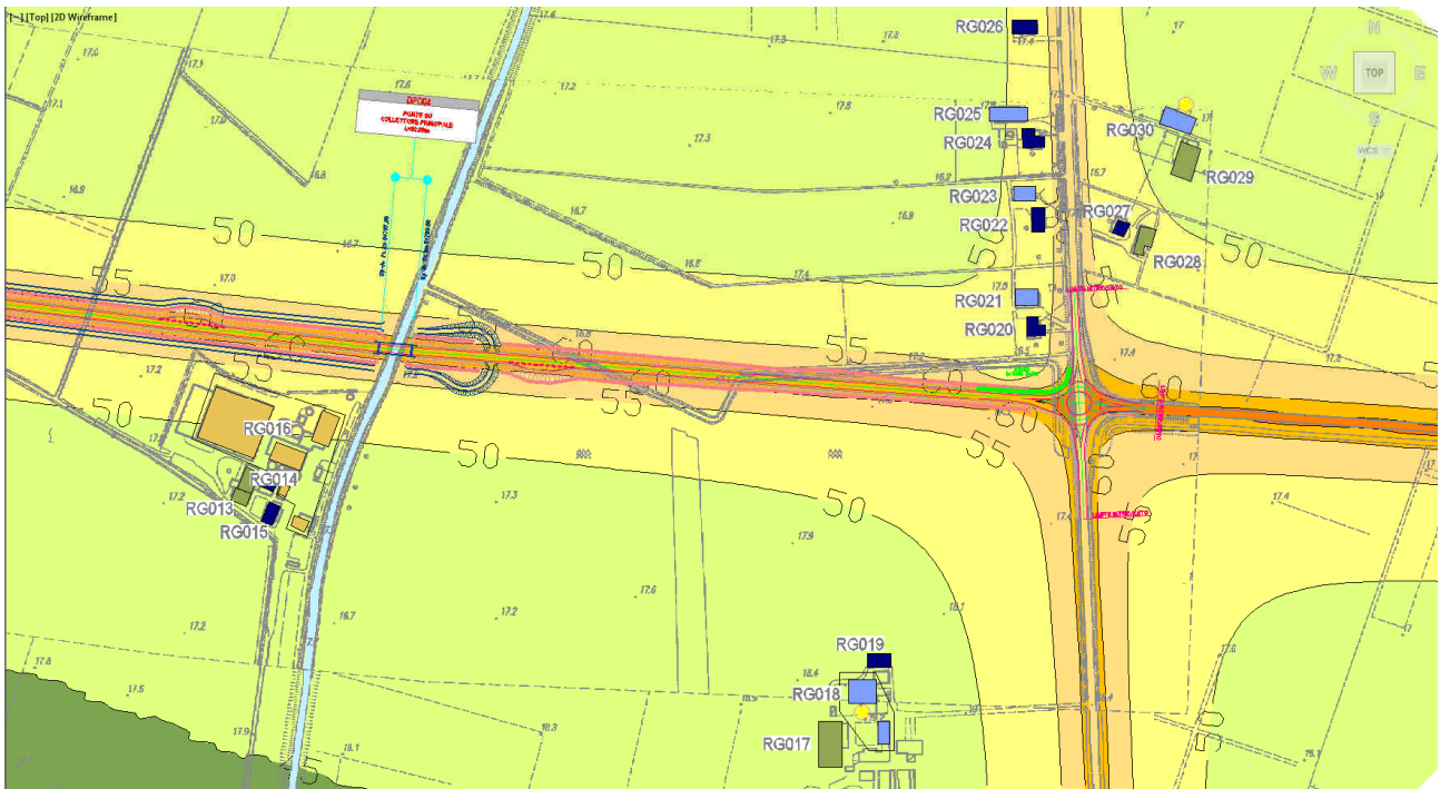
FIGURA 8.3-3 – DETTAGLIO DELLA MAPPATURA DELLE ISOFONICHE IN CORRISPONDENZA DEL RICETTORE RG020
