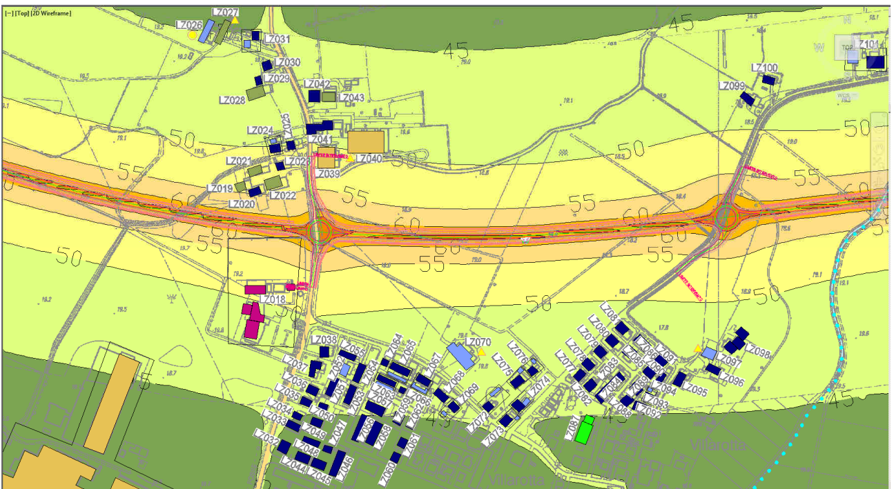
FIGURA 6.5-2 – PARTICOLARE DELLA MAPPATURA DELLE ISOFONICHE NEL TRATTO CENTRALE DELL'OPERA DI ADDUZIONE D03
