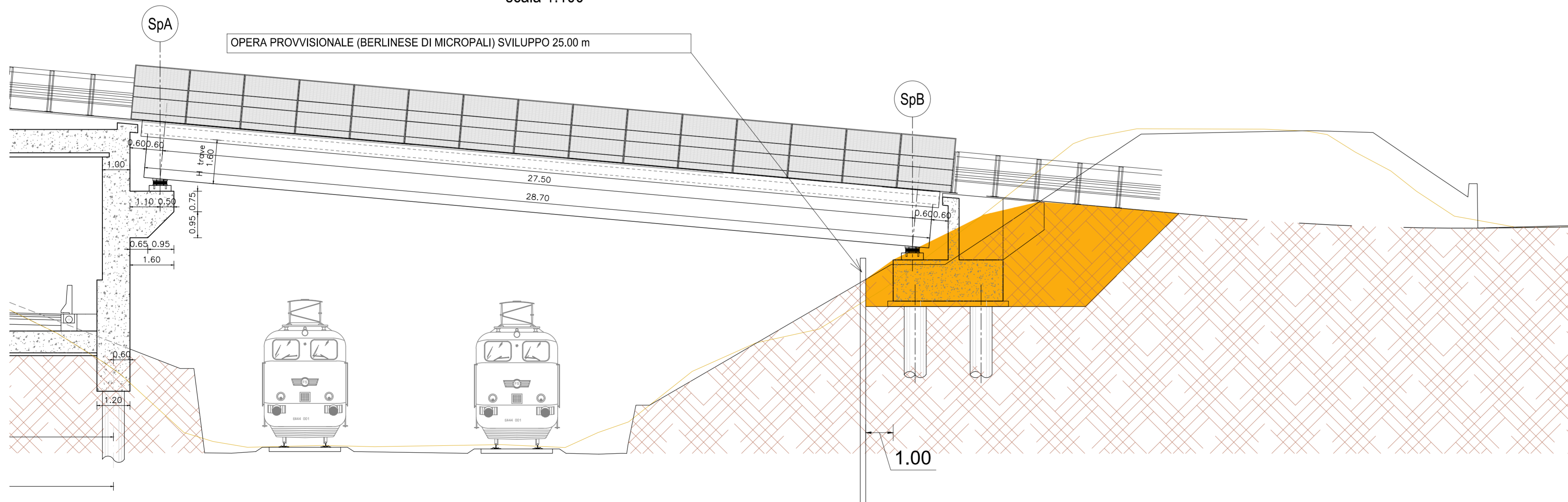
PROSPETTO VISTA LONGITUDINALE VIABILITÀ SEC 01 scala 1:100
