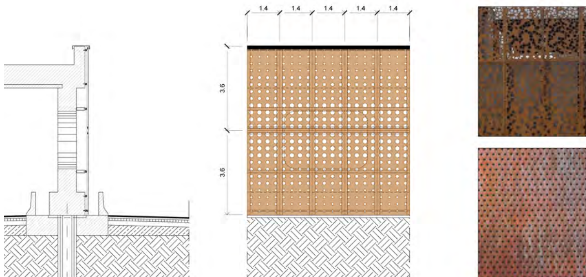
Figura 9.10 Galleria Ripa di Olmo, dettaglio del rivestimento in acciaio corten, a forometria variabile – tratto singola fornice.
