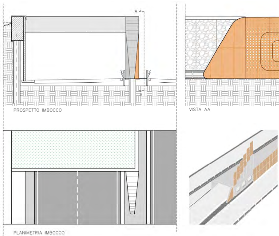
Figura 9.12 Galleria Ripa di Olmo – Imbocco con elementi rastremati, rivestiti in acciaio corten sulla faccia esterna.
