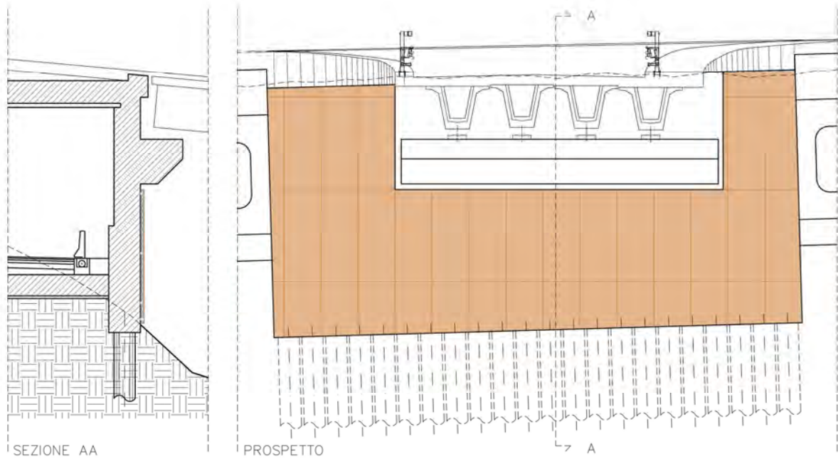
Figura 9.11 Galleria Ripa di Olmo – Rivestimento in acciaio corten pieno – tratto a doppia fornice (sotto al cavalcavia CV01).
