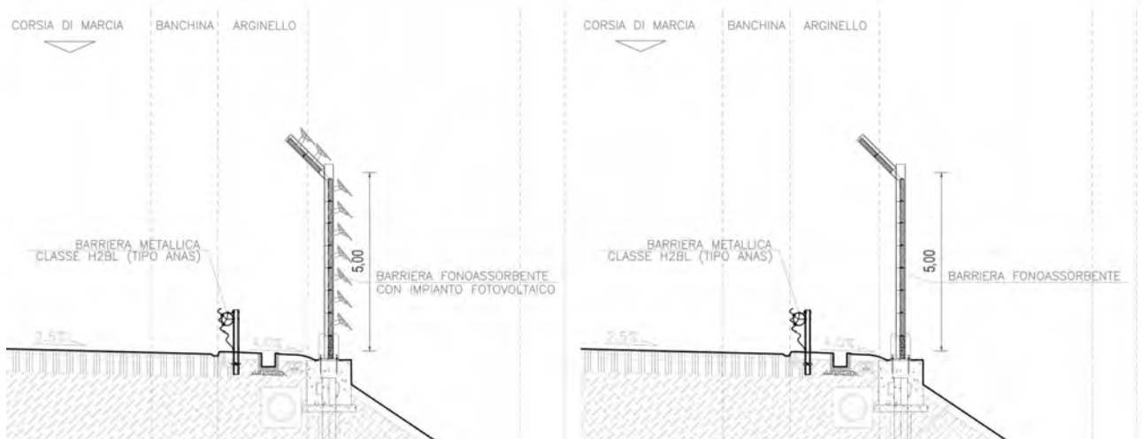
Figura 7.18 Tipologico barriere acustiche in acciaio corten con e senza pannelli fotovoltaici.
