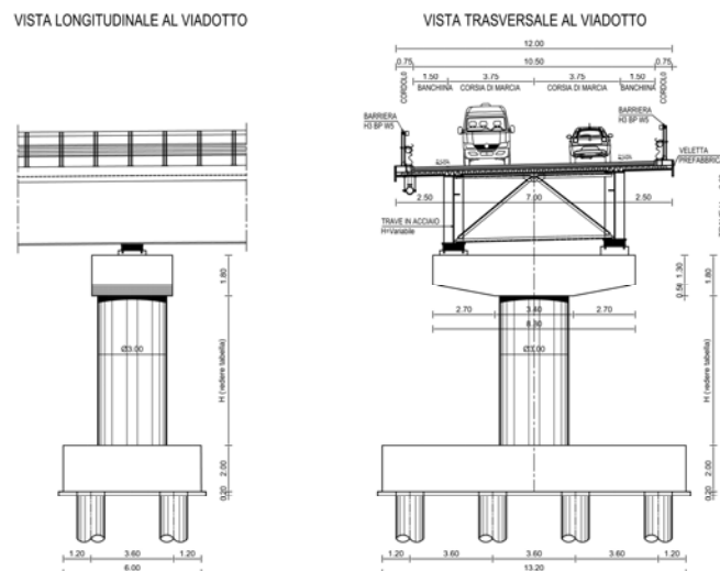
Figura 9.6 Sezione trasversale e longitudinale del cavalcavia San Giuliano.
