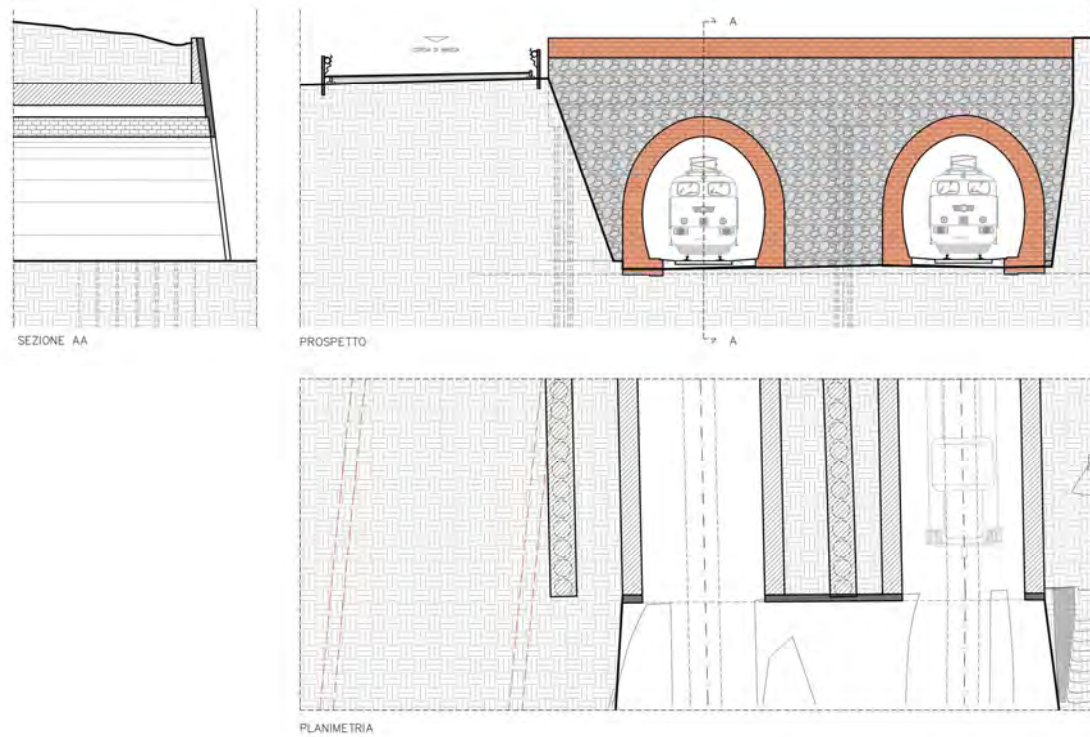
Figura 9.14 Imbocco ovest della galleria ferroviaria su modello di quello esistente.
