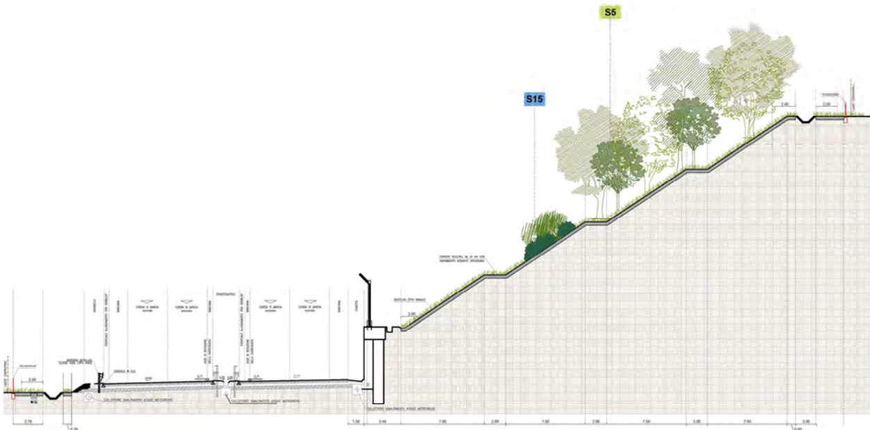
Figura 2.5 Sezione del passaggio del nuovo asse stradale in prossimità delle pendici del Bosco di Sargiano con utilizzo distanziato di siepi termofile e alberi per ricucitura boschiva non resinosi (si vedano i sestii di impianto riportati S5 e S15).
