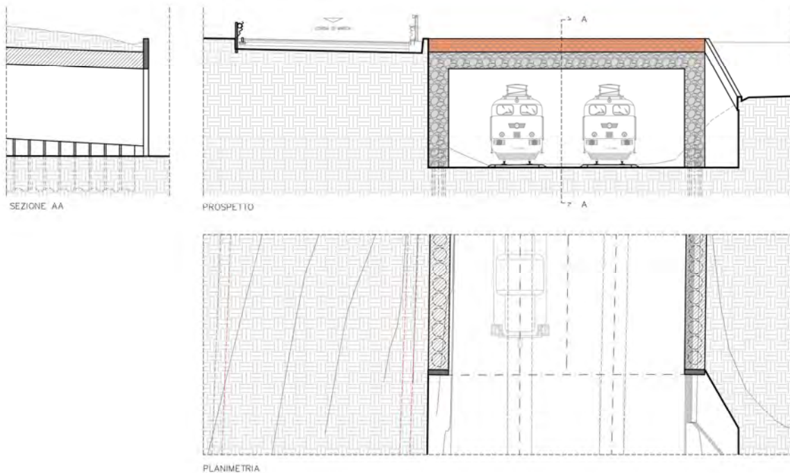
Figura 9.15 Imbocco est del prolungamento della galleria ferroviaria esistente.
