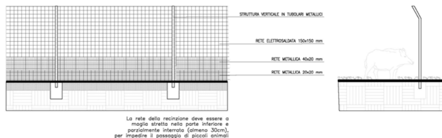
Figura 9.1 Assonometria schematica, prospetto e sezione della recinzione e delle rampe di fuga.
