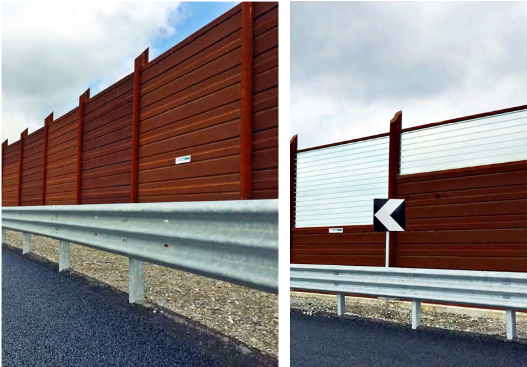
Figura 9.19 Immagine di riferimento per barriere antirumore in acciaio corten – Senza inserto trasparente e con inserto in vetro con rigatura orizzontale.
