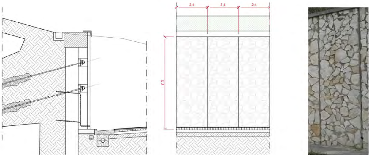
Figura 9.17 Rivestimenti muri e paratie in C.A. - dettaglio dei rivestimenti in pietra naturale.
