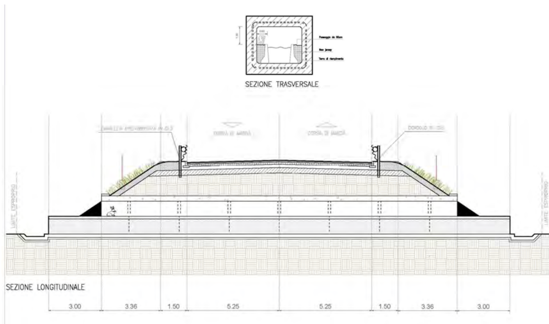
Figura 9.2 Sezione tipologica.
