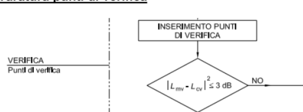
Figura 3-3 schema a blocchi taratura secondo UNI 11143-1 2005.
