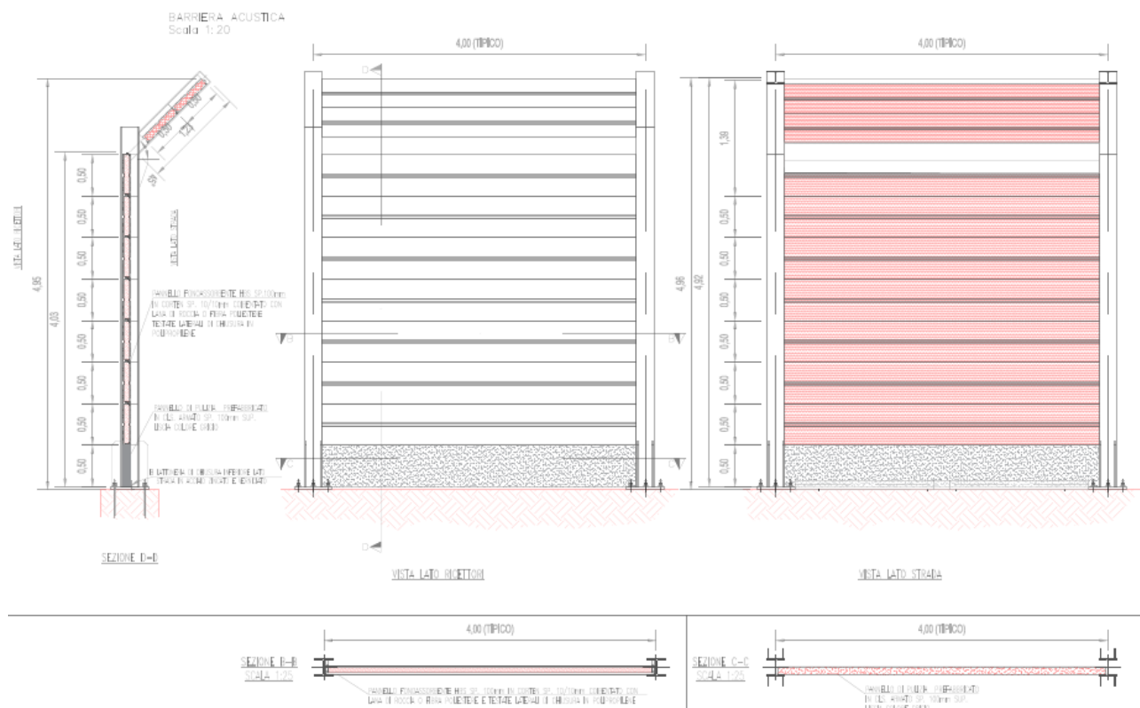
Figura 3-5 Particolare di una barriera.
