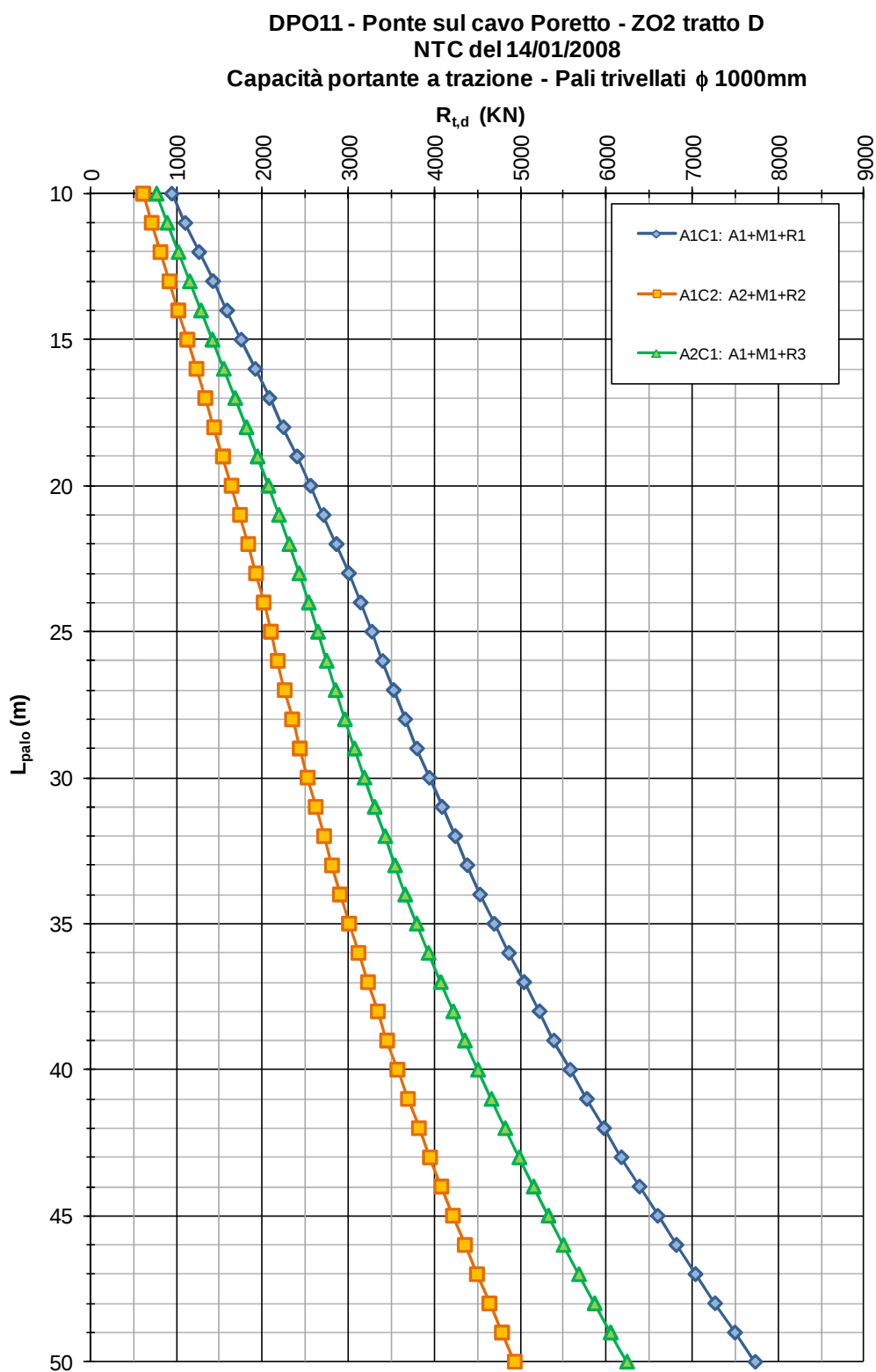
FIGURA 4-2: CAPACITÀ PORTANTE A TRAZIONE – PALI TRIVELLATI \phi 1000
