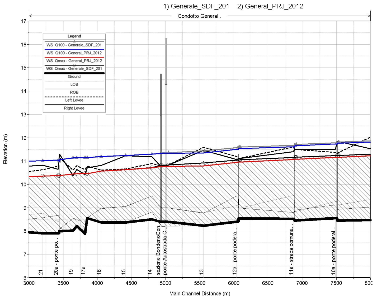
FIGURA 7-4: CONDOTTO GENERALE, DETTAGLIO DEL CONFRONTO TRA I PROFILI DI RIGURGITO PER LE PORTATE Q_{MAX} E Q_{100} NELLO STATO DI FATTO E DI PROGETTO
