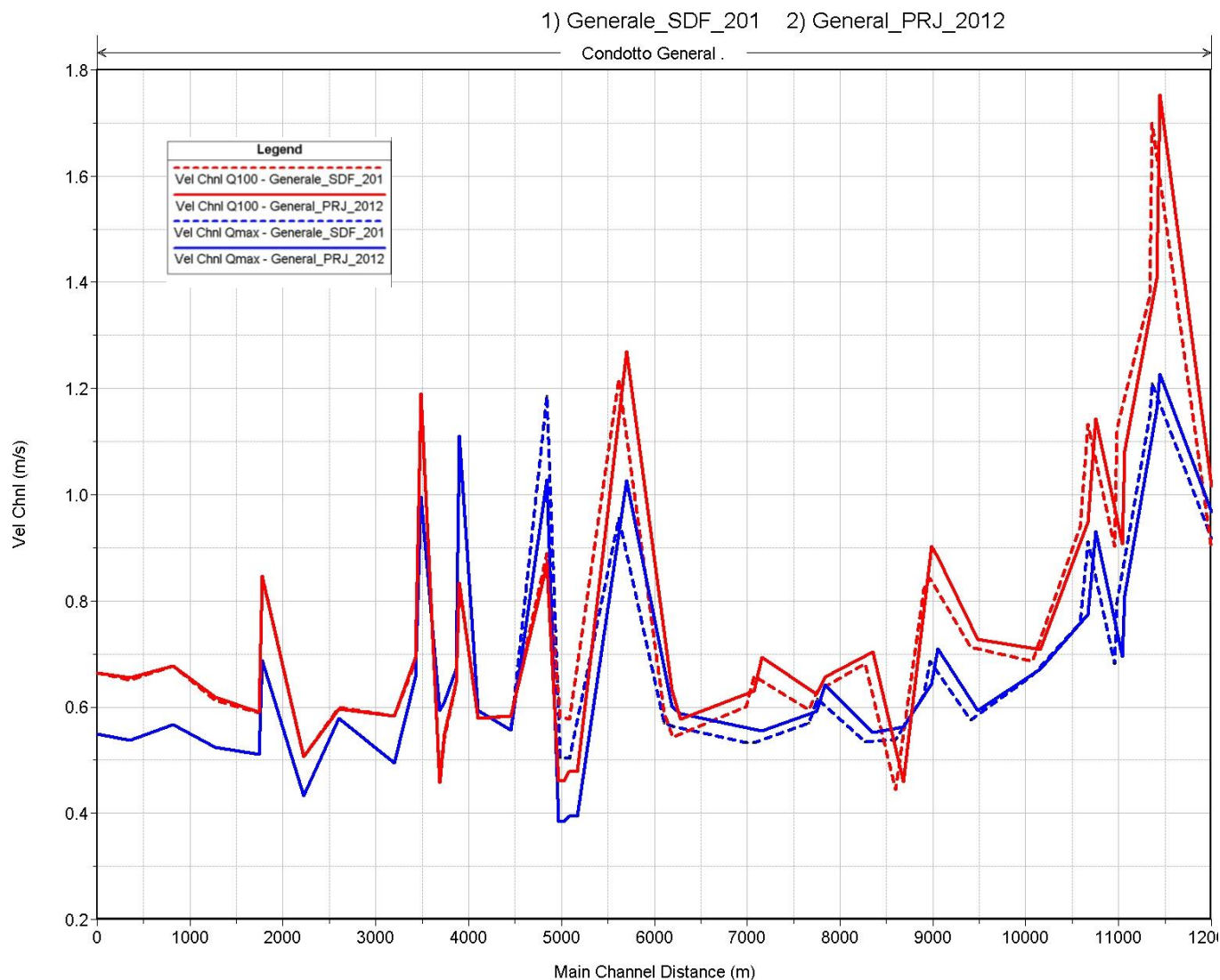
FIGURA 7-5: CONDOTTO GENERALE, ANDAMENTO DELLA VELOCITÀ MEDIE DELLA CORRENTE PER LE PORTATE NELLO STATO DI FATTO E DI PROGETTO.
