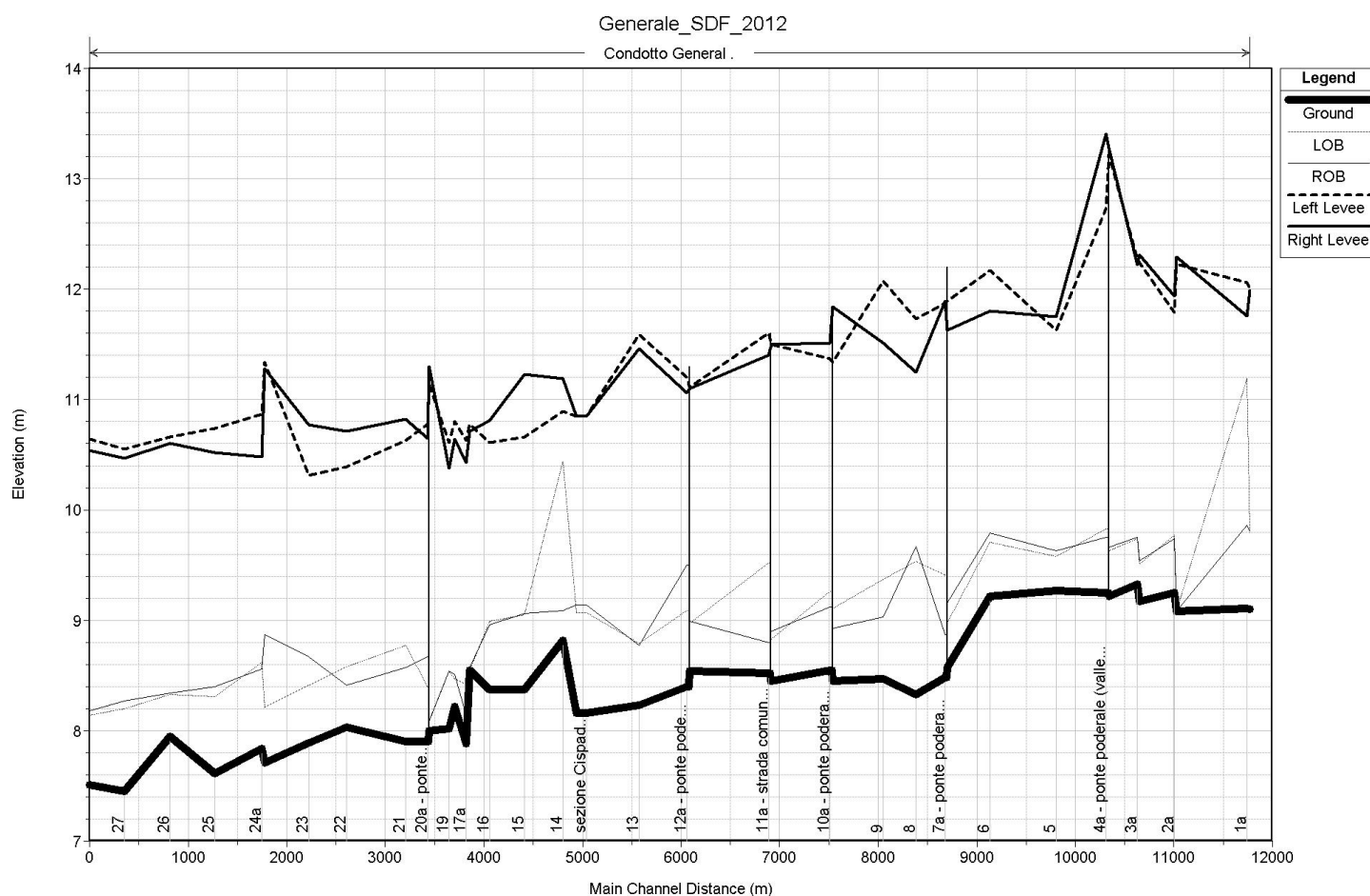
FIGURA 5-1: ANDAMENTO LONGITUDINALE DEL THALWEG E DELLE SPONDE NEL TRATTO DI CANALE ANALIZZATO
