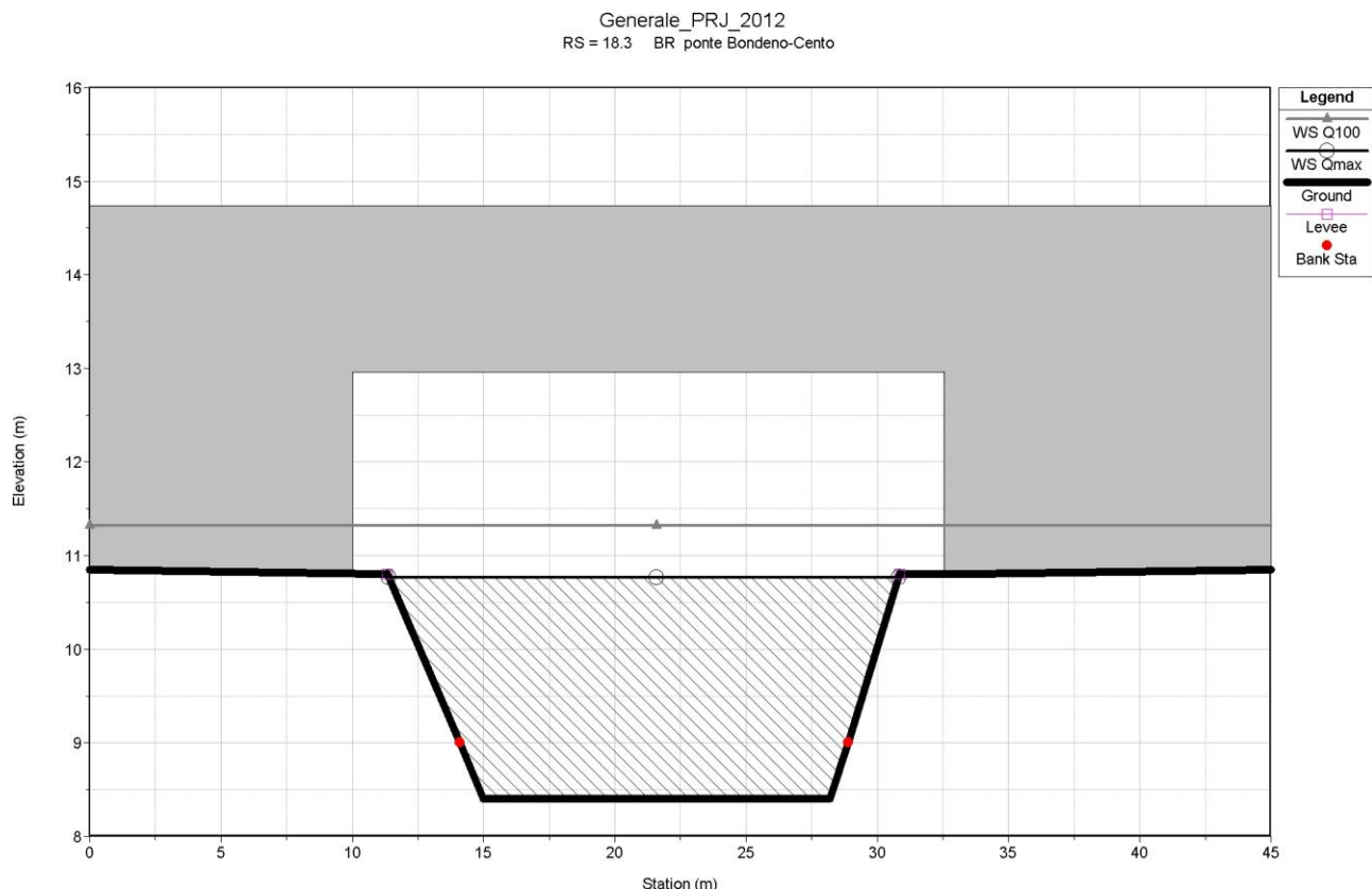
FIGURA 7-2: LIVELLO IDROMETRICO RAGGIUNTO PER Q_{MAX} E Q_{100} ALLA SEZIONE TRASVERSALE IN CORRISPONDENZA DELL'ASSE STRADALE NELLO STATO DI PROGETTO
