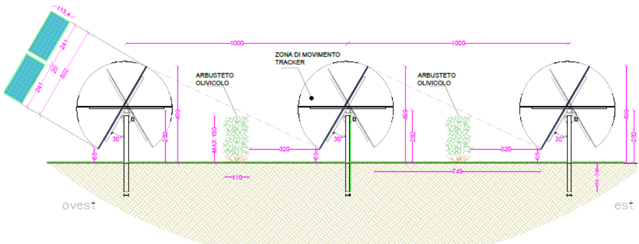
Figura 4 - Sezione tipo impianto con installazione su sistema ad inseguimento solare tipo tracker
