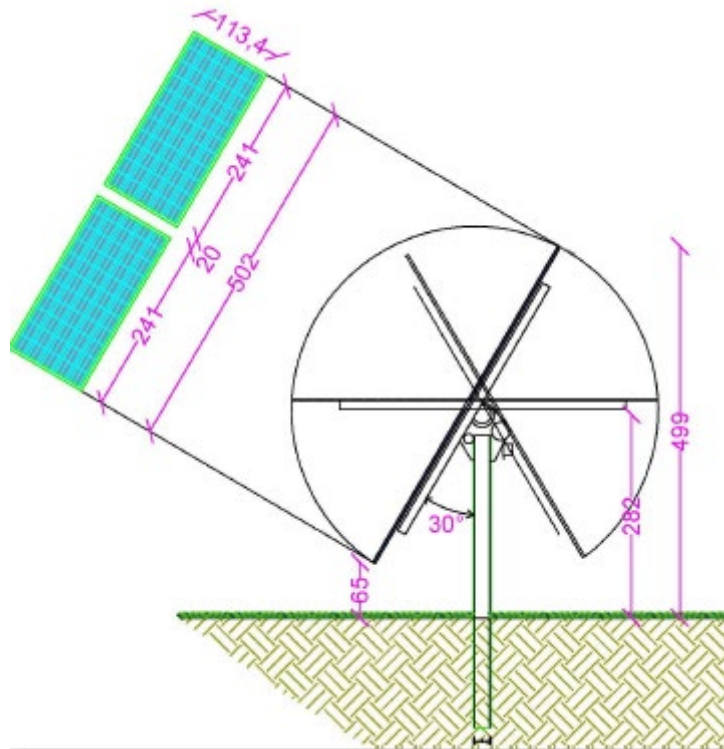
Figura 3 - Estratto elaborato MBFAF96_Elaborato_Grafico_R.5.c (Particolari costruttivi)
