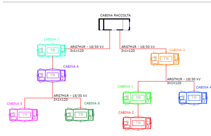
Schema a blocchi anello MT di collegamento cabine di trasformazione MT/BT
