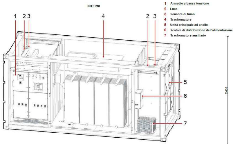
Configurazione di massima degli skid "Huawei"
