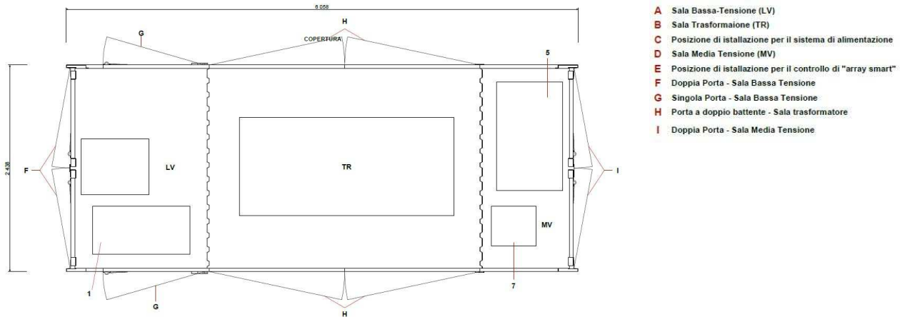
Layout di uno skid "Huawei"
