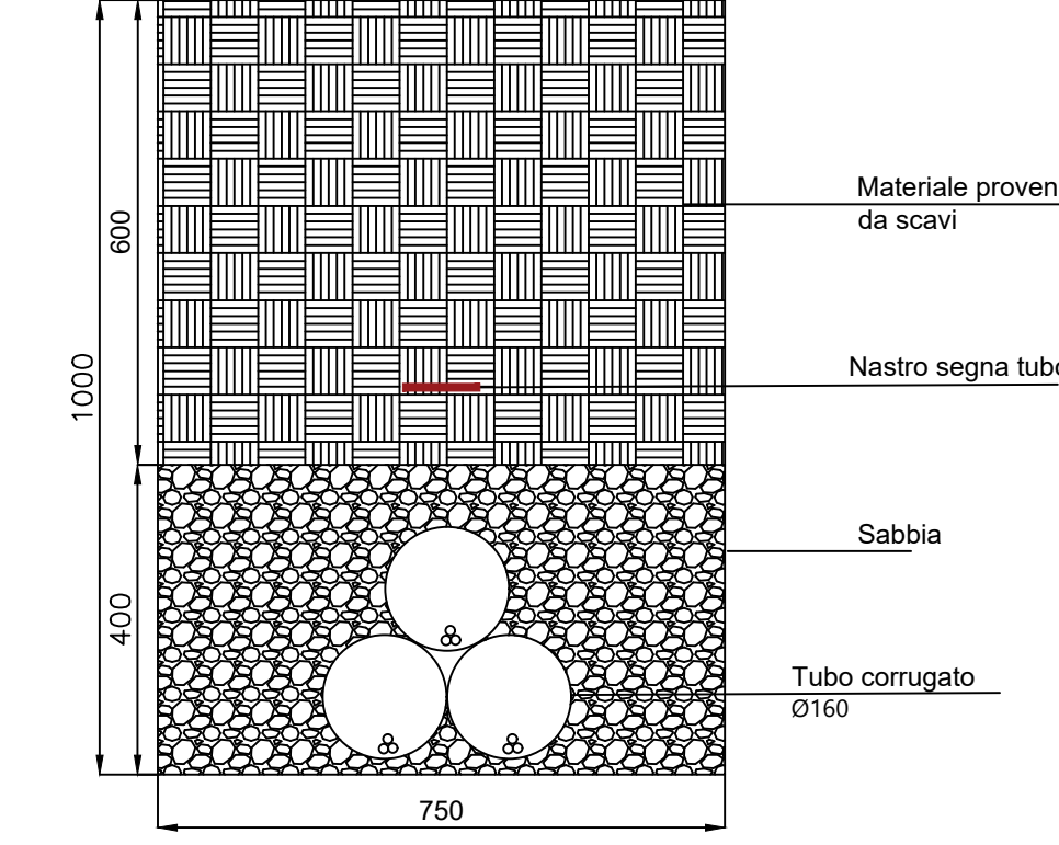
SEZIONE TIPO CAVIDOTTO SU TERRA
