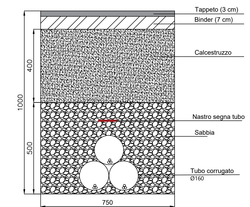
SEZIONE TIPO CAVIDOTTO SU STRADA PROVINCIALE
