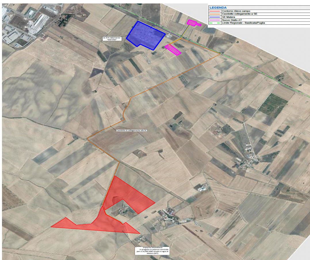
Tavola n. 5: ubicazione area impianto e sottostazione di AT esistente.
