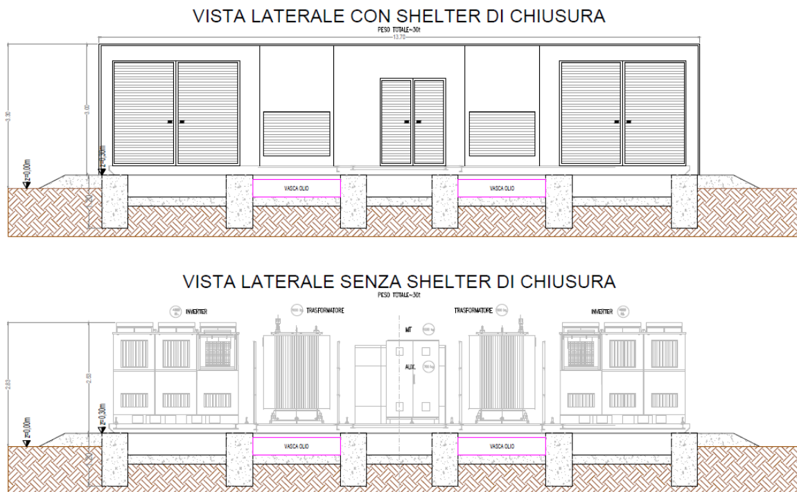
Figura 6 - Layout preliminare cabina di trasformazione BT/MT (cfg doppia) con/senza shelter di chiusura
