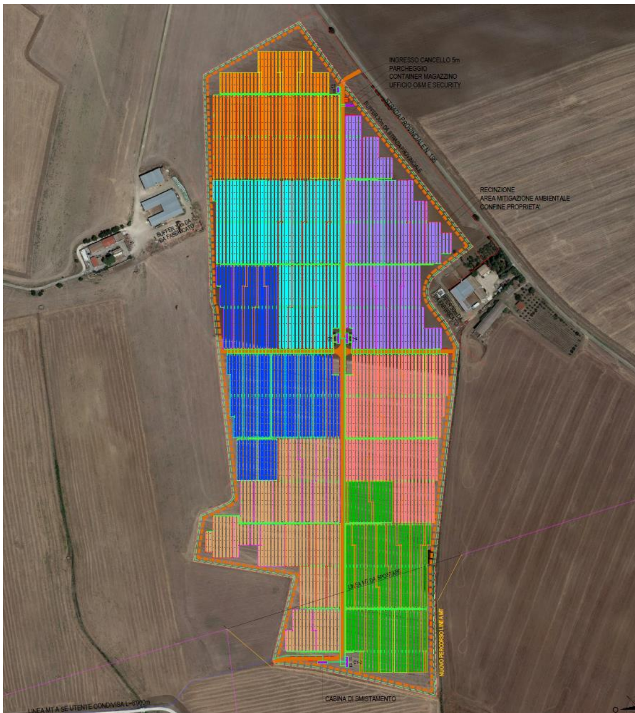
Figura 2 - Layout d'impianto su ortofoto
