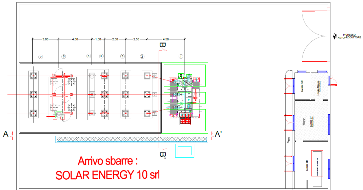
Figura 12 - Layout della sottostazione utente
