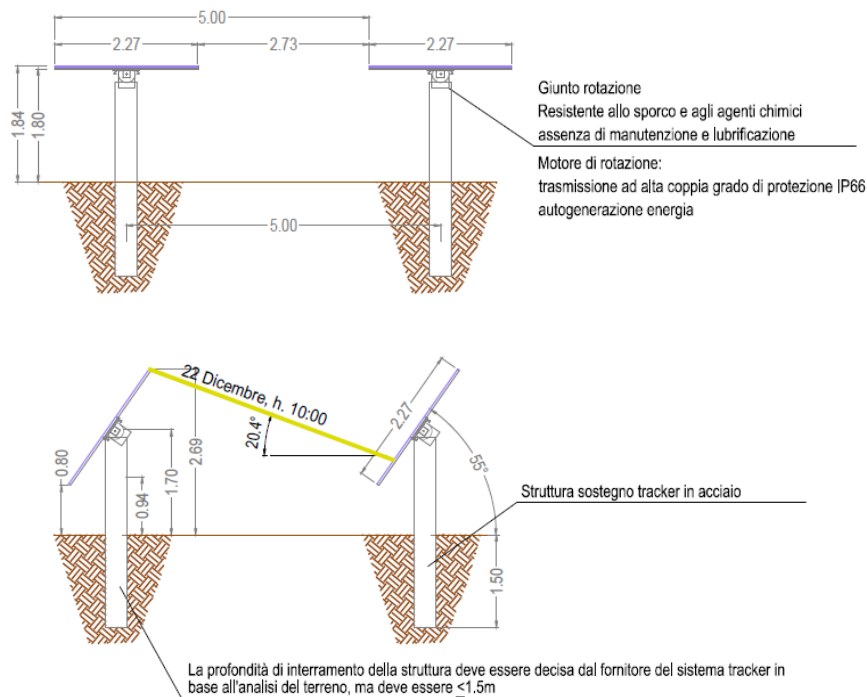
Figura 4 - Inseguitori mono-assiali: modalità di installazione e principali quotature
