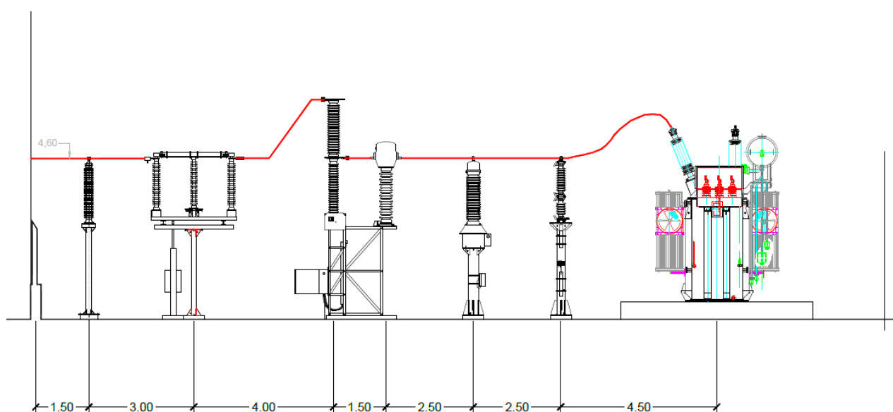
Figura 13 - Vista laterale delle apparecchiature elettromeccaniche in AT
