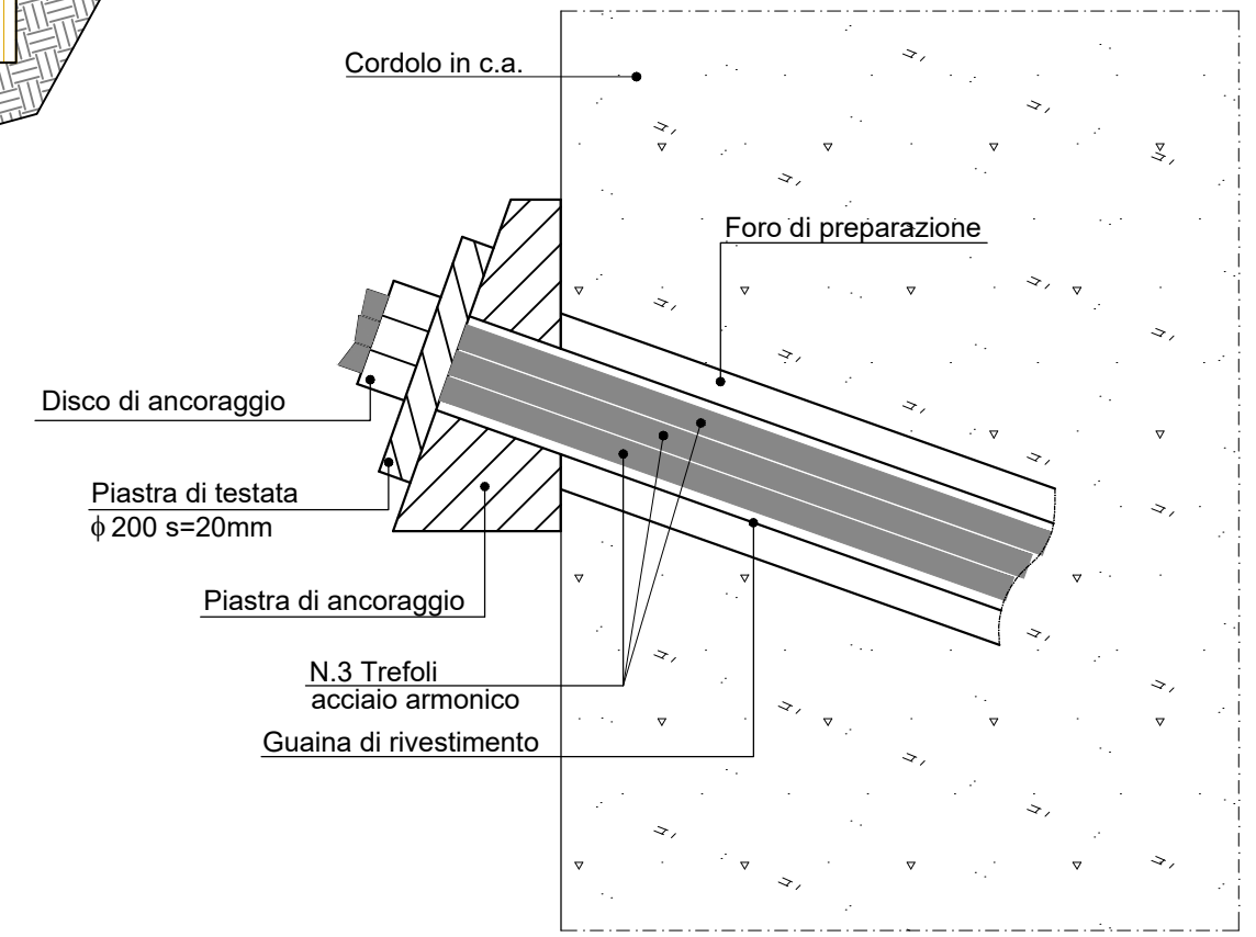
PARTICOLARE TIRANTE SCALA FS
