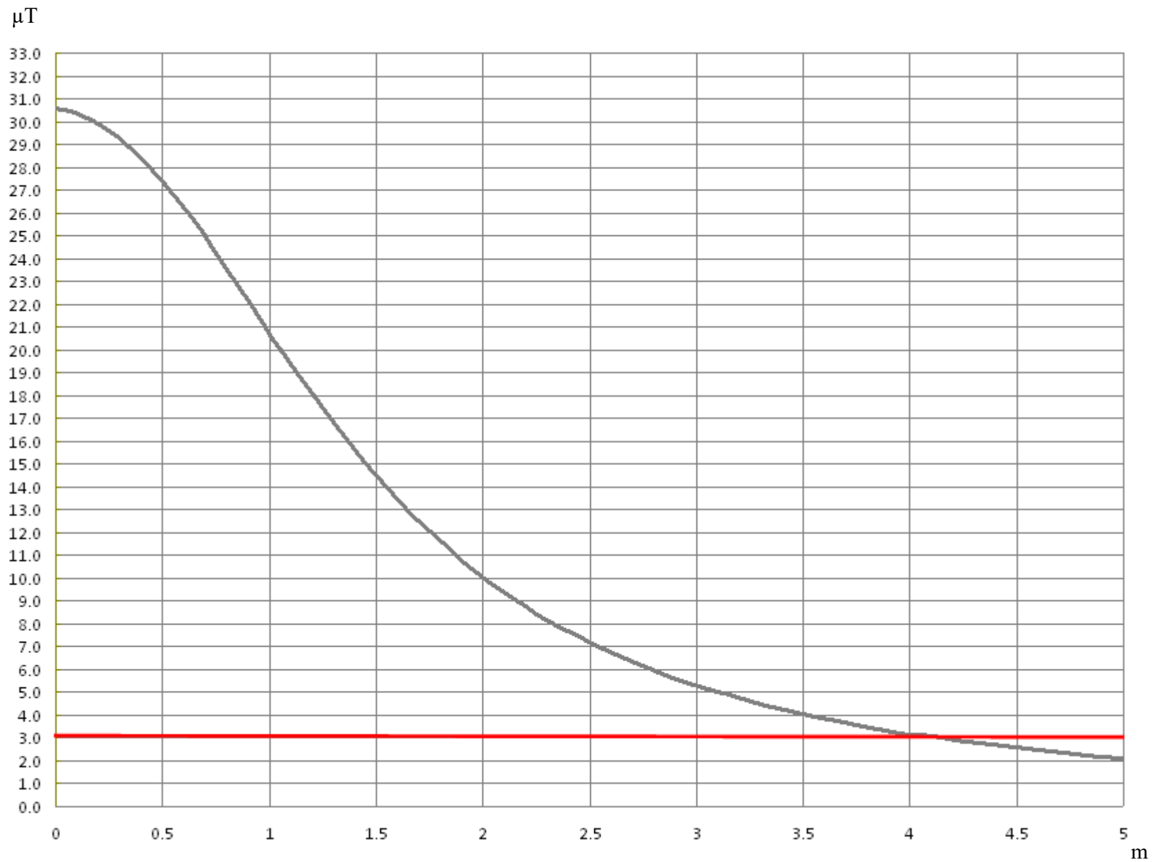
Valore dell'induzione magnetica al suolo del cavidotto MT nel tratto composto da 5 terne da 630 mm 2
