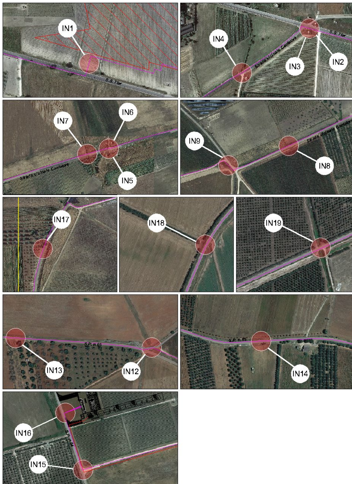
Figura 5 - Interferenze del cavo M.T. con sottoservizi esistenti
