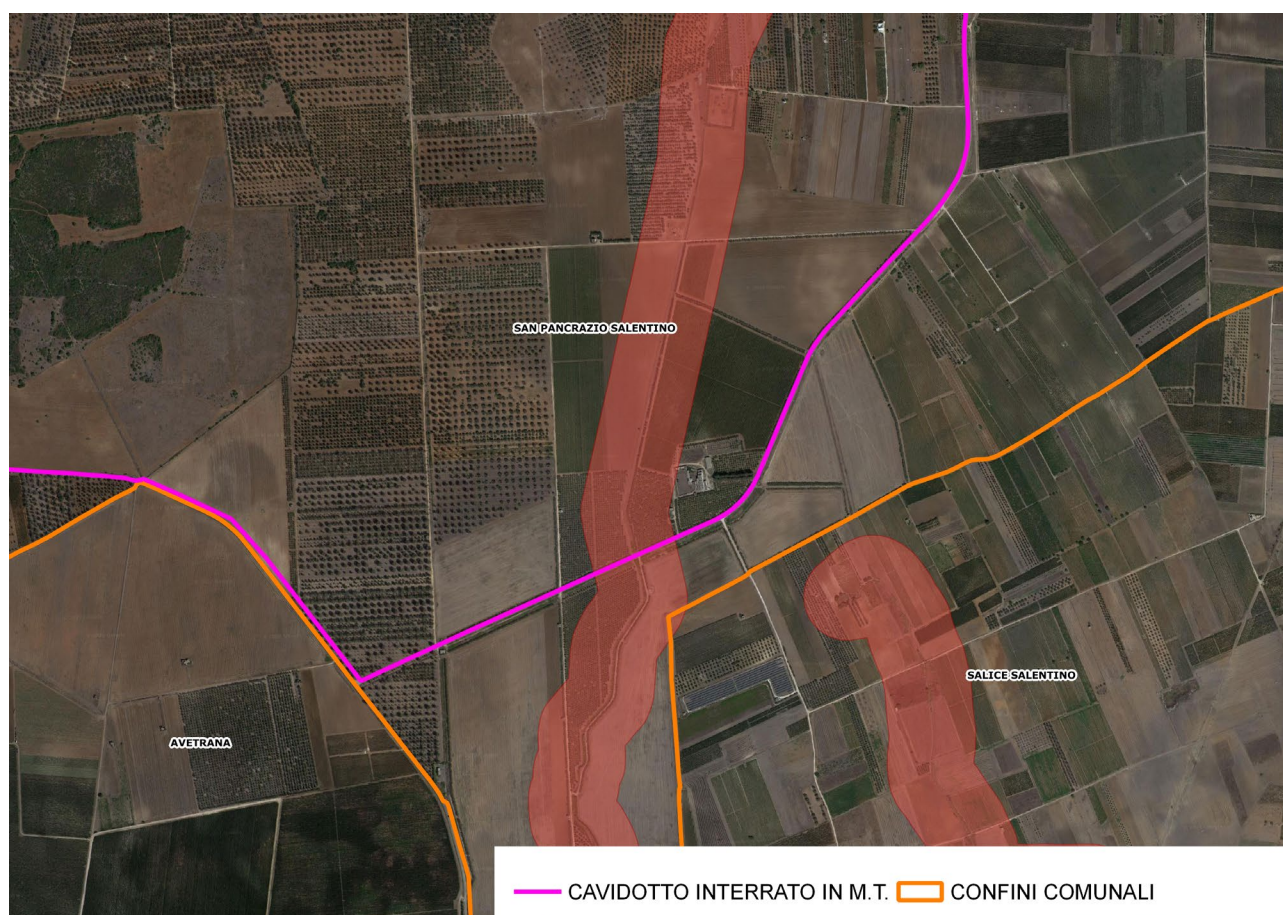
Figura 12: stralcio del PPRT, interferenza con "Canale presso Mass.a Campone", UCP Reticolo idrografico di connessione della R.E.R. nel tratto in posa interrata al di sotto della SP65. E' prevista la risoluzione dell'interferenza mediante il ricorso alla posa con tecnica no-dig (senza scavo) con passaggio al di sotto del canale.
