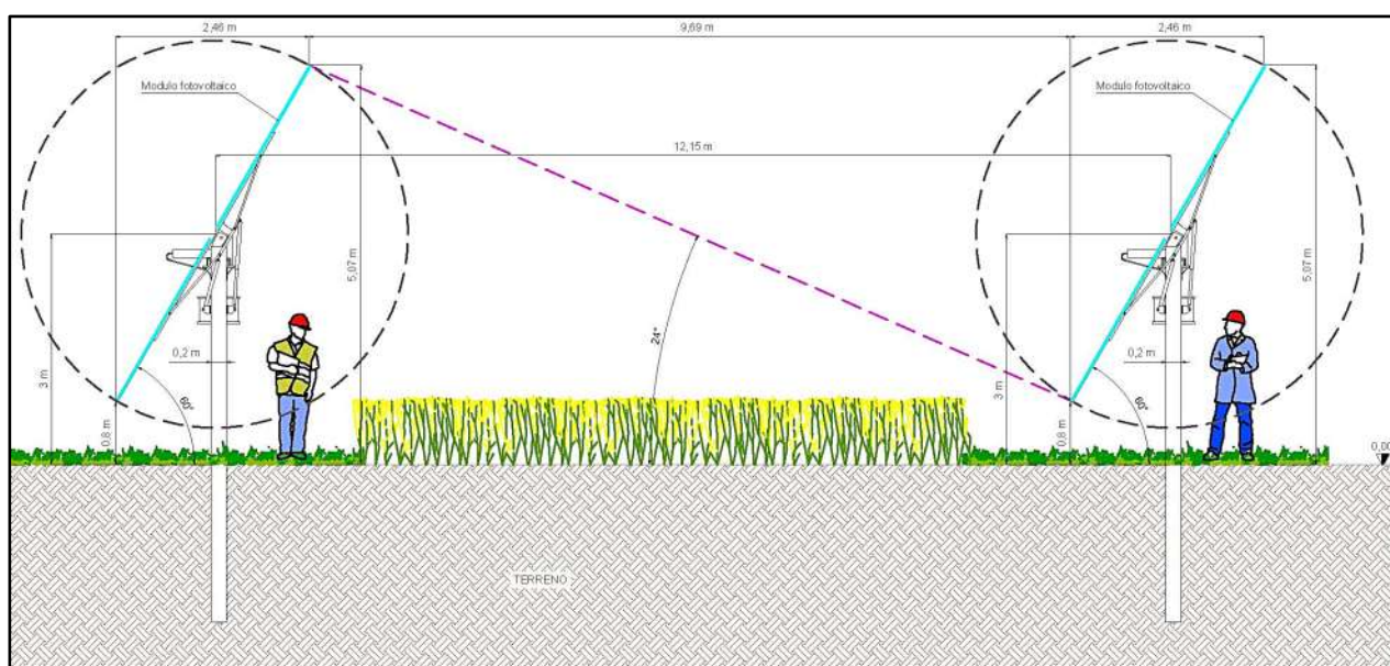
mpianto fotovoltaico con inseguitori monoassiali
