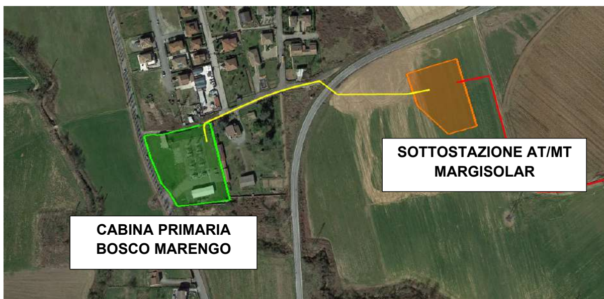
Dettaglio del tracciato del cavidotto AT
