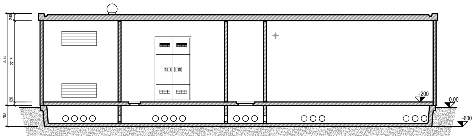
SEZIONE A-A'
