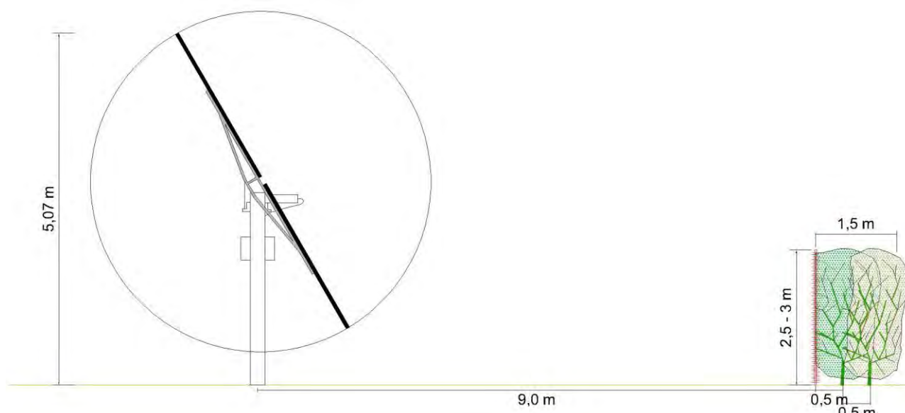
Figura 4: Schema di siepe – Sezione trasversale
