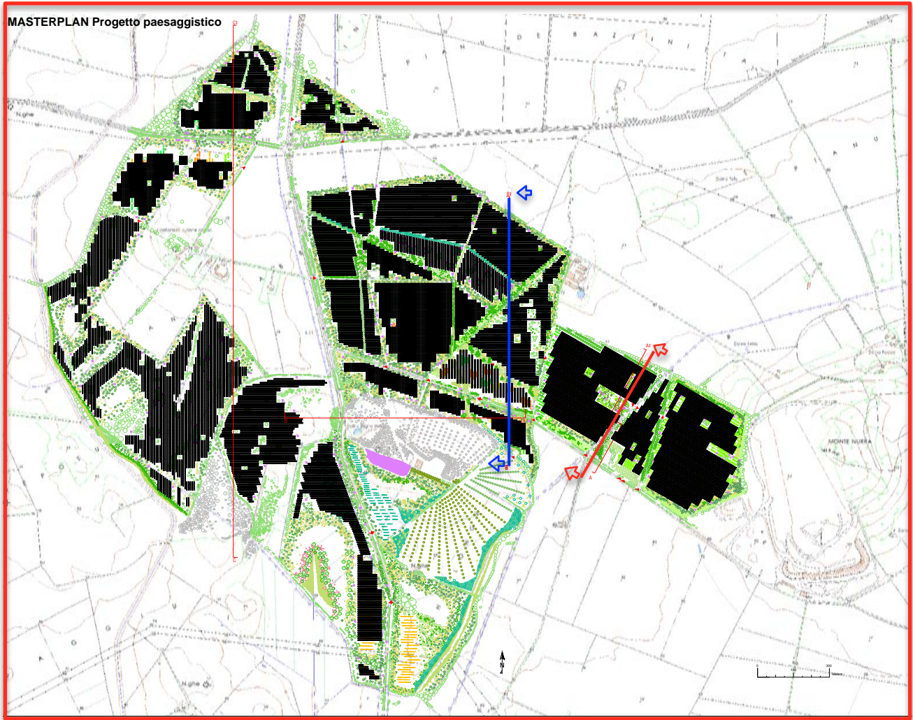
PROGETTO PAESAGGISTICO / PLANIMETRIA E SEZIONI A/A' - B/B' - C/C'
