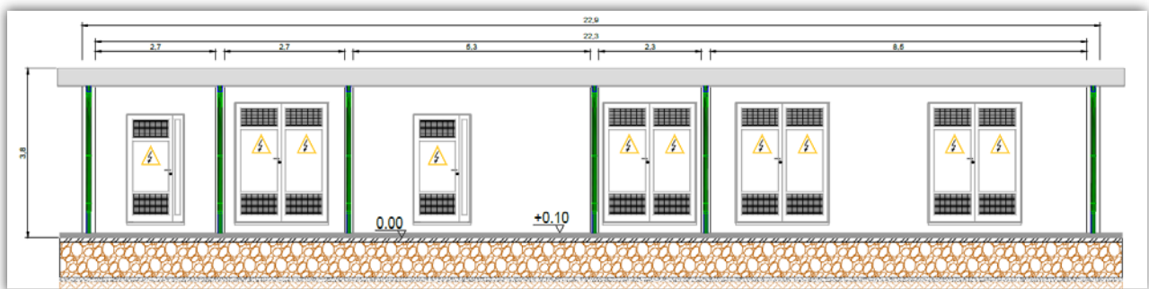
Fig. 44. Prospetto principale dei locali tecnici della SSE.
