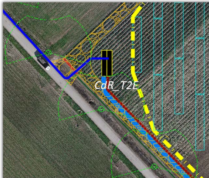
Fig. 27. Dettaglio della CdR EST: in rosso scuro, la linea proveniente dalle varie cabine di conversione e trasformazione; in blu la dorsale proveniente dalla CdR_T2C; in celeste le linee dorsali in partenza verso la Sottostazione Produttore
