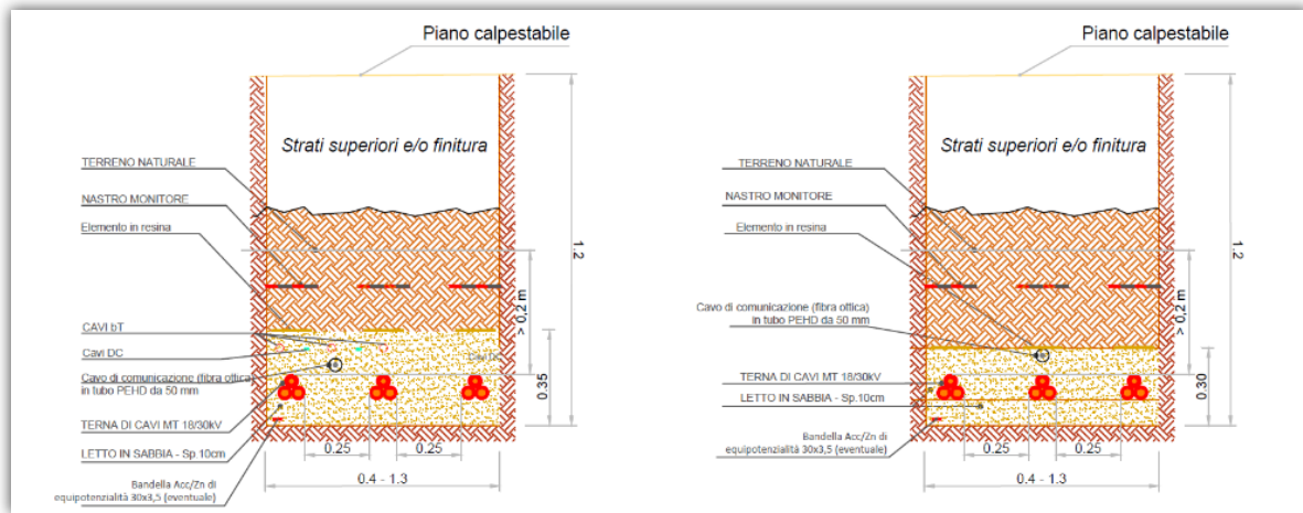
Fig. 34. – Particolare: tipico scavo MT per 1-4 terne MT; a sinistra, con presenza di cavi bT.
