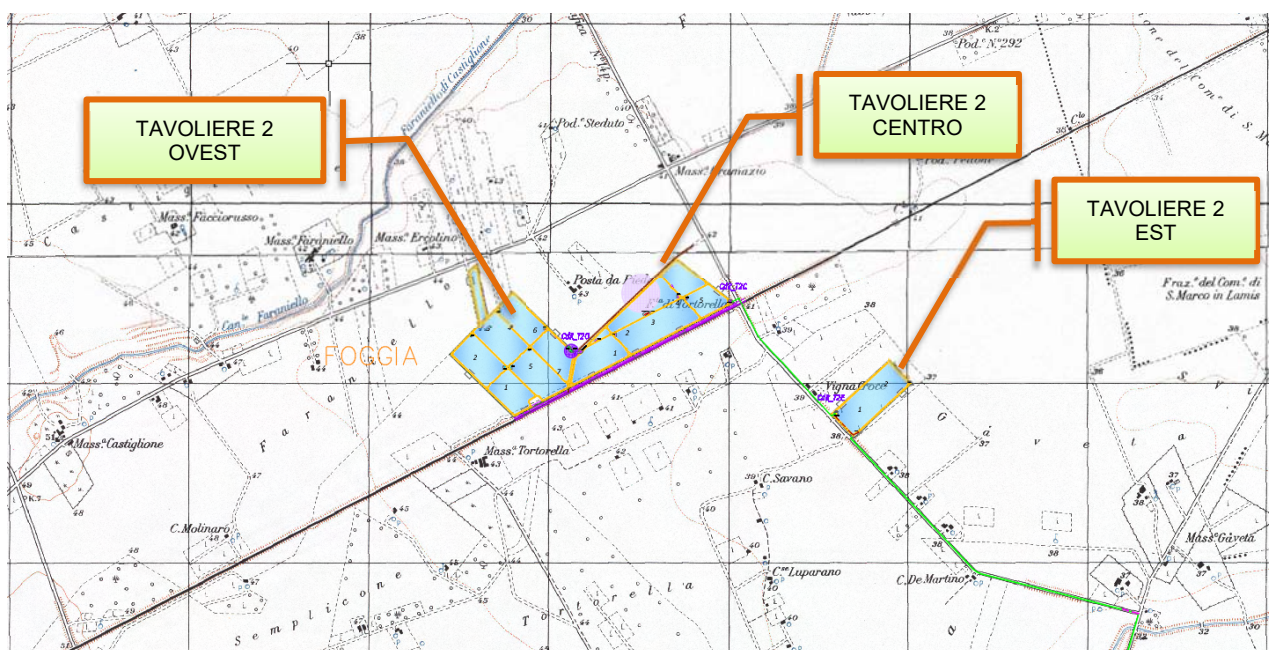
Fig. 9. Layout impianto con identificazione dei Sottoimpianti OVEST, CENTRO e EST, e tratto iniziale dell'elettrodoto dorsale (in VERDE) su I.G.M.
