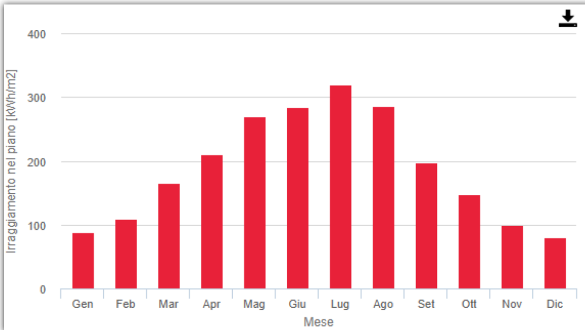
Fig. 7. Grado di irraggiamento complessivo sul piano dei moduli mensile in località Borgo Tavernola (fonte PVGIS)
