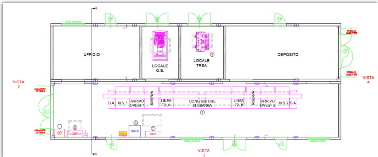
Fig. 28. Tipico PIANTA delle Cabine di Raccolta: in alto il locale bT, con i gruppi di continuità ed il TRSA, oltre ad un vano uso ufficio ed un vano deposito; in basso il locale destinato a soli Quadri MT (dimensioni complessive 15,00 x 6,20 x 4,50h).
