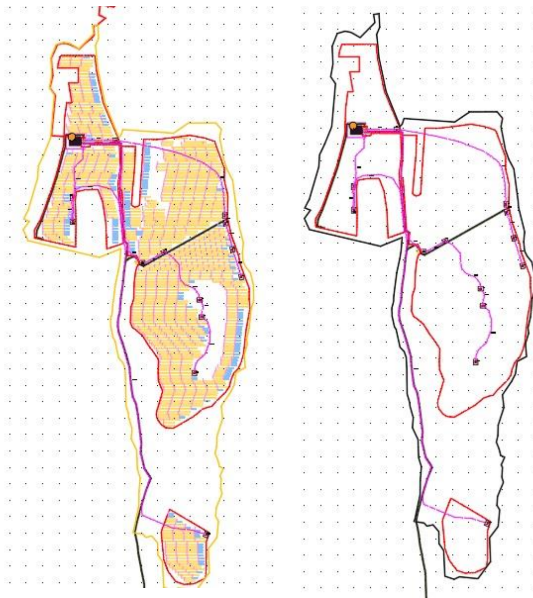
Figura 3.1: Stato di progetto dell'area di impianto
