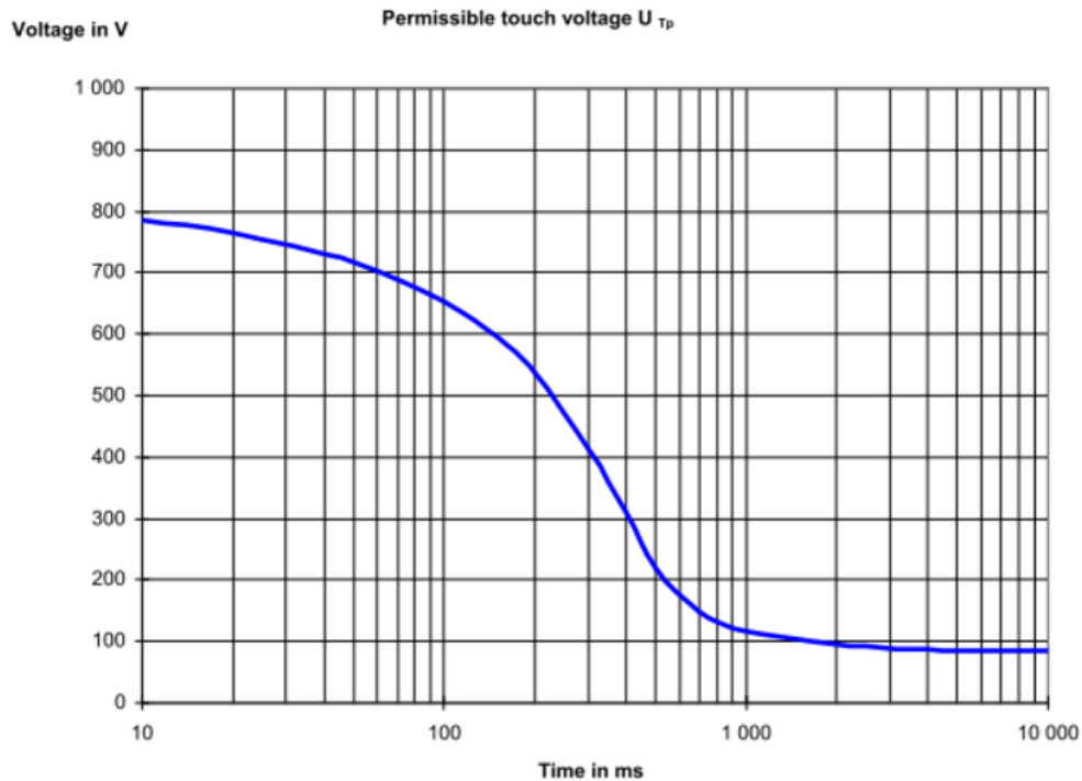
Figura .1: Massima tensione ammissibile (CEI EN 50522, Fig.4
