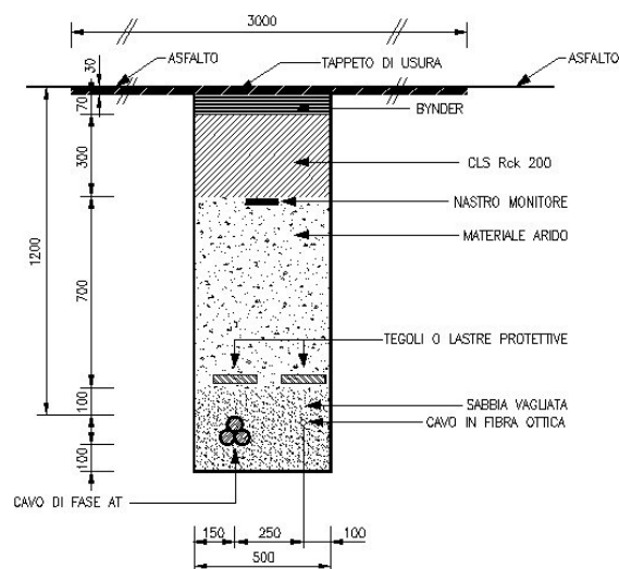
Figura 4: Tipici di posa cavi AT su strade asfaltate
