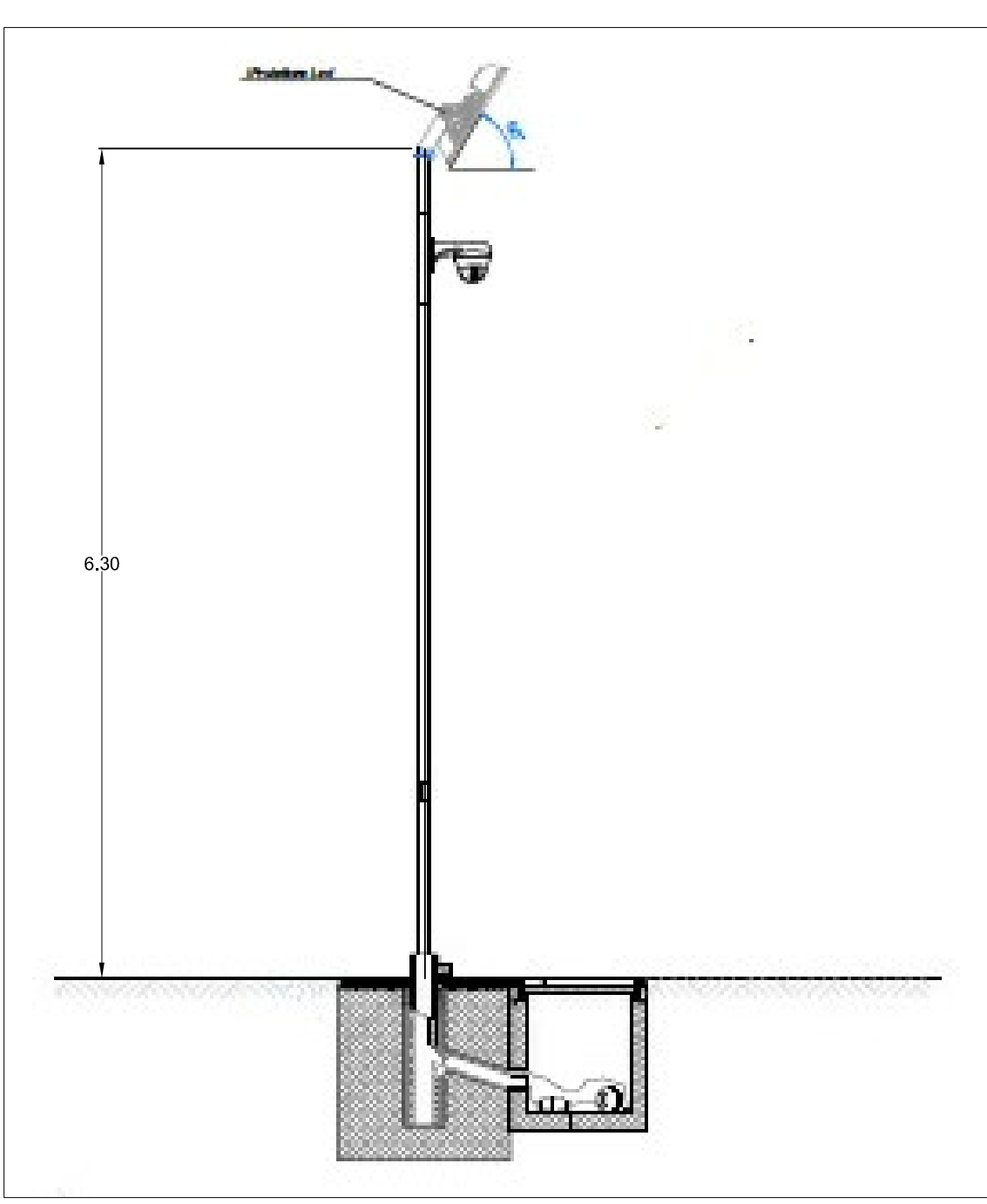
Particolare Sostegno videosorveglianza ed illuminazione perimetrale scala 1:50
