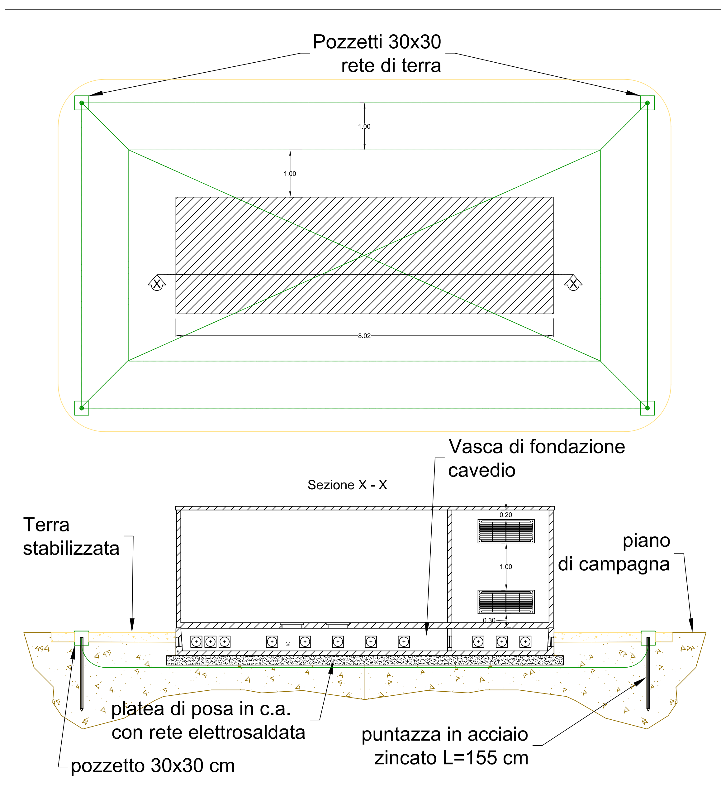
Particolare Posa Cabina di Consegna Scala 1: 50
