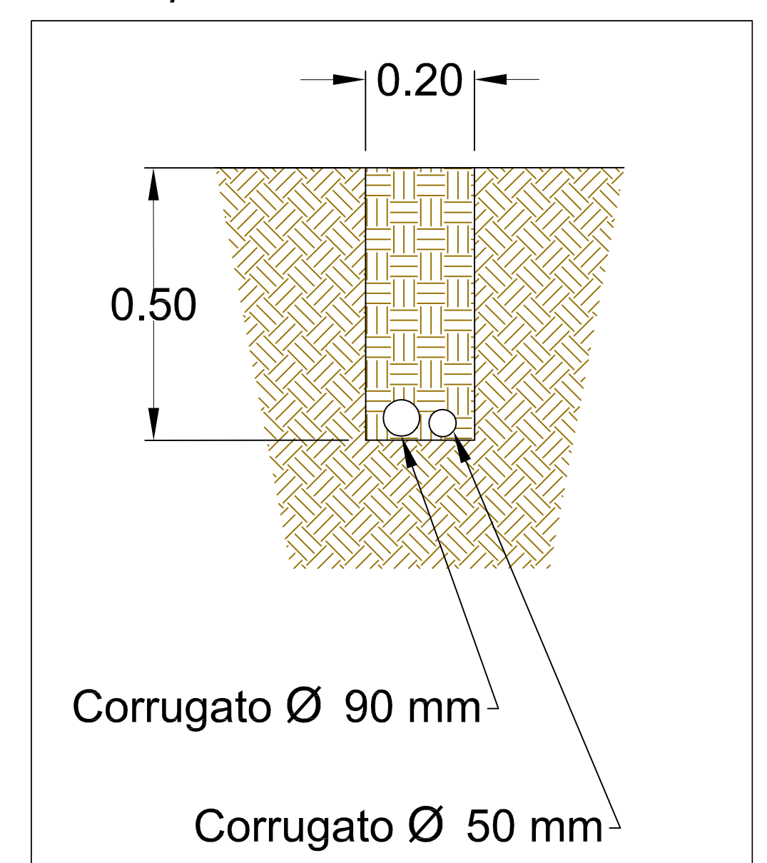
Particolare cavidotto perimetrale scala 1:25
