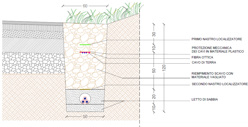
Figura 39: Sezione tipo del cavidotto in fregio alla viabilità esistente
