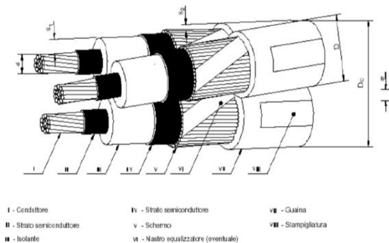
Figura 38: Cavo tipo MT
