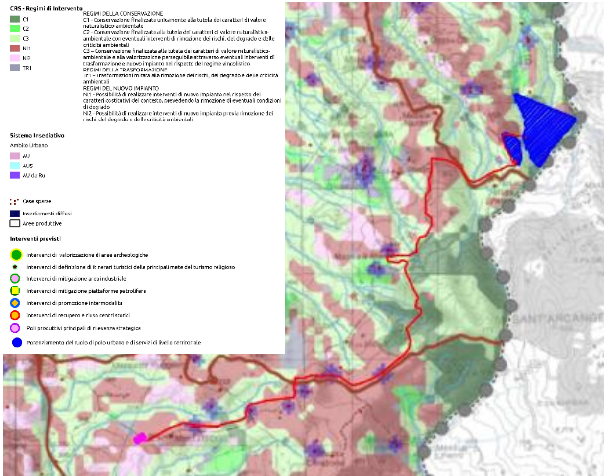
Figura 14: PSP - Carta con indicazione dei regimi di intervento e strategie programmate
