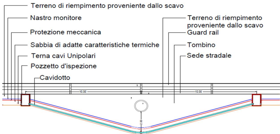
Figura 46: Risoluzione interferenze mediante TOC
