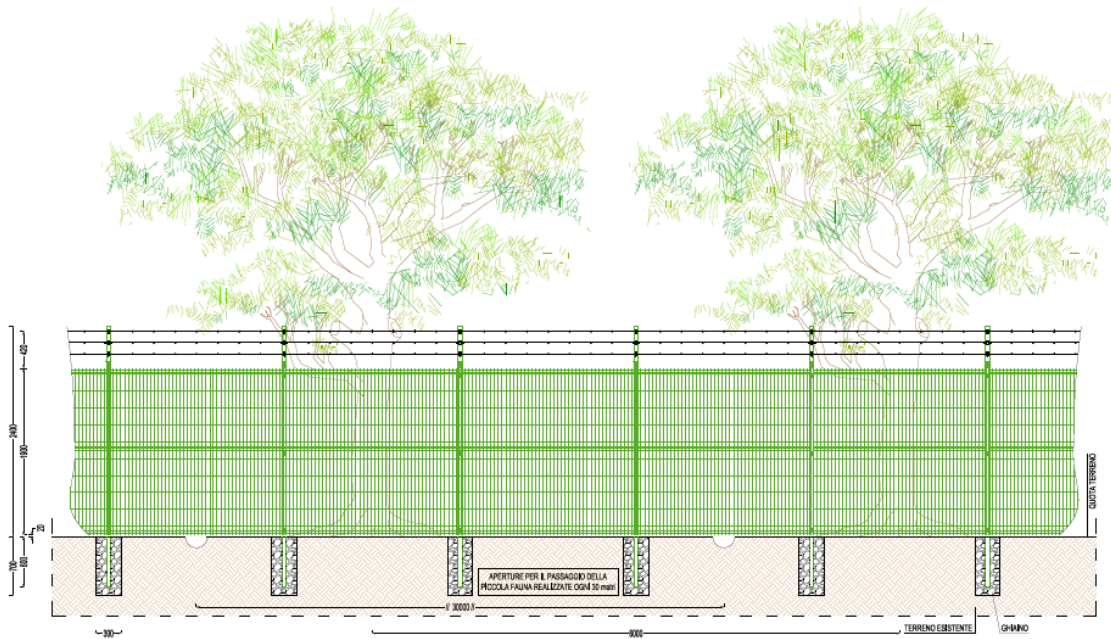
Figura 37: Prospetto recinzione con fascia di mitigazione
