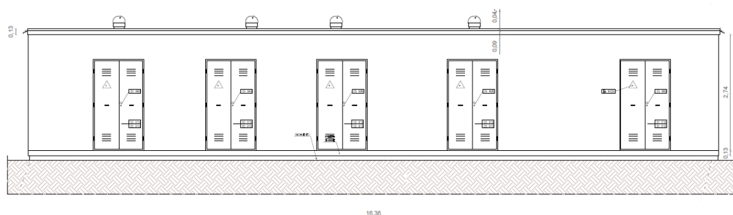
Figura 33: Cabina di raccolta
