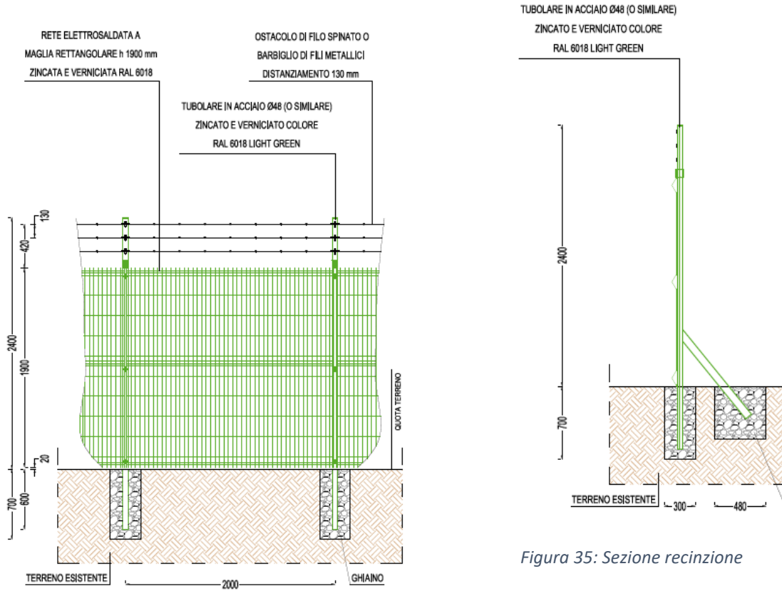
Figura 34: Prospetto recinzione
