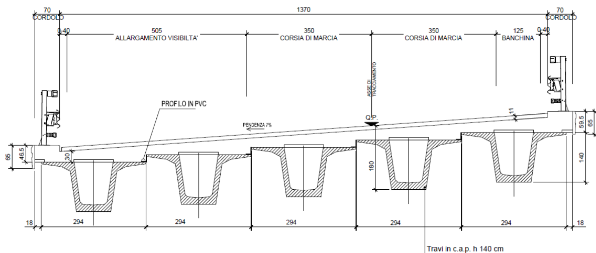
FIGURA 1-1 SEZIONE TRASVERSALE TIPICA
