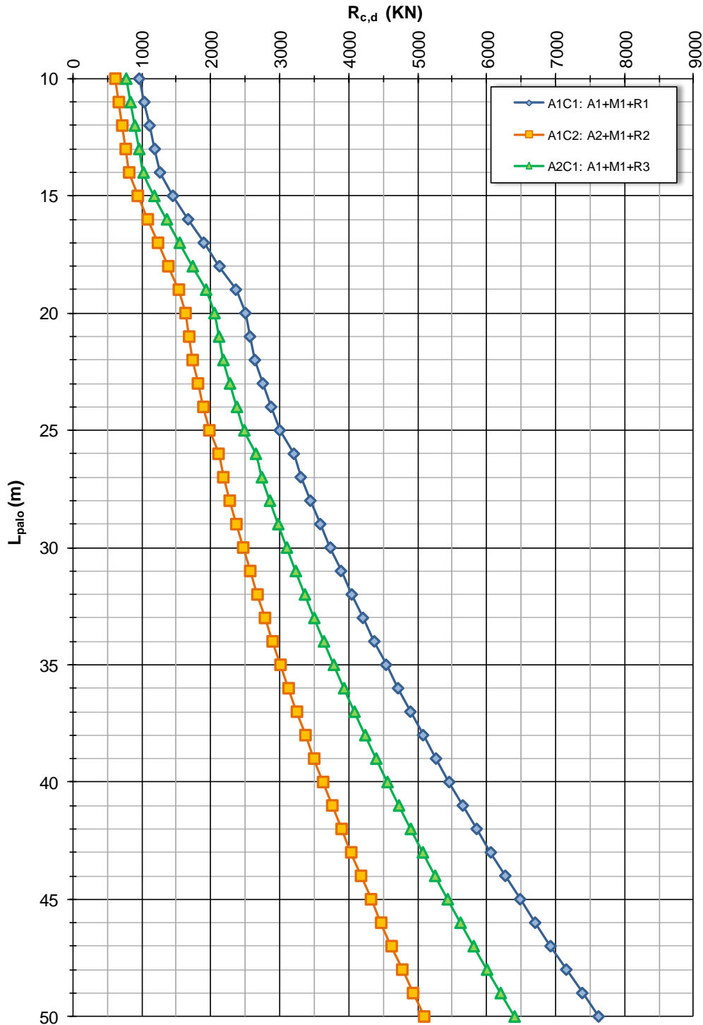
FIGURA 5.1.11-2 CAPACITA' PORTANTE PALO
