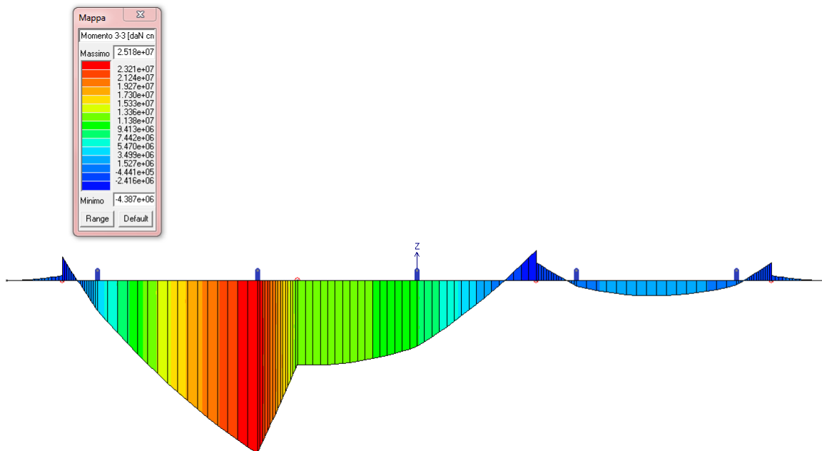
FIGURA 10-14 COMBINAZIONE SLE FREQUENTE 1 : MOMENTO FLETTENTE
