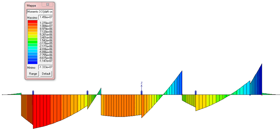
FIGURA 10-10 COMBINAZIONE SLV 2 : MOMENTO FLETTENTE
