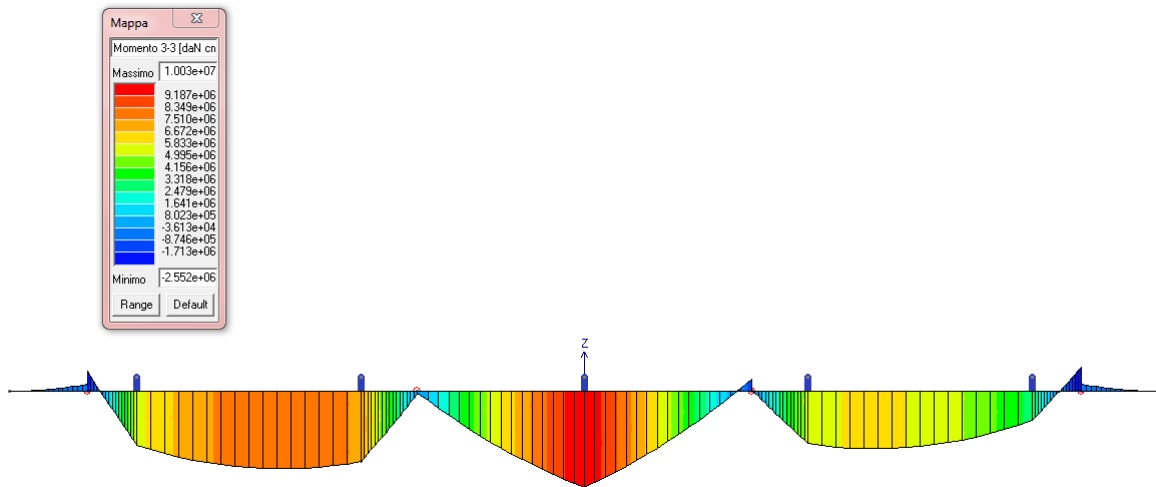
FIGURA 10-12 COMBINAZIONE SLE RARA 1 : MOMENTO FLETTENTE
