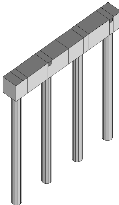
FIGURA 10-1 MODELLAZIONE UTILIZZATA VISTA 3D
