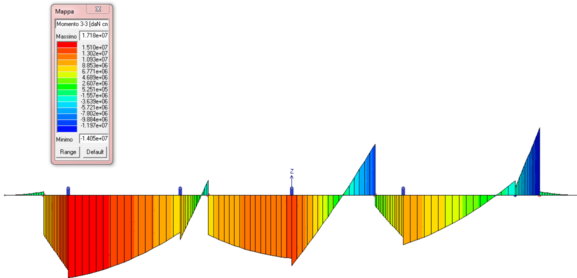
FIGURA 10-8 COMBINAZIONE SLV 1 : MOMENTO FLETTENTE
