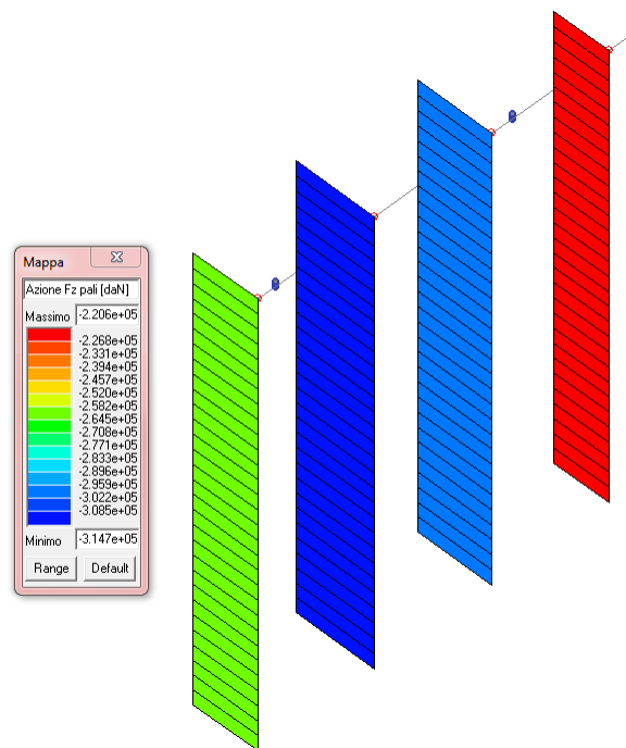
FIGURA 5.1.11-1 CARICO SU PALO
