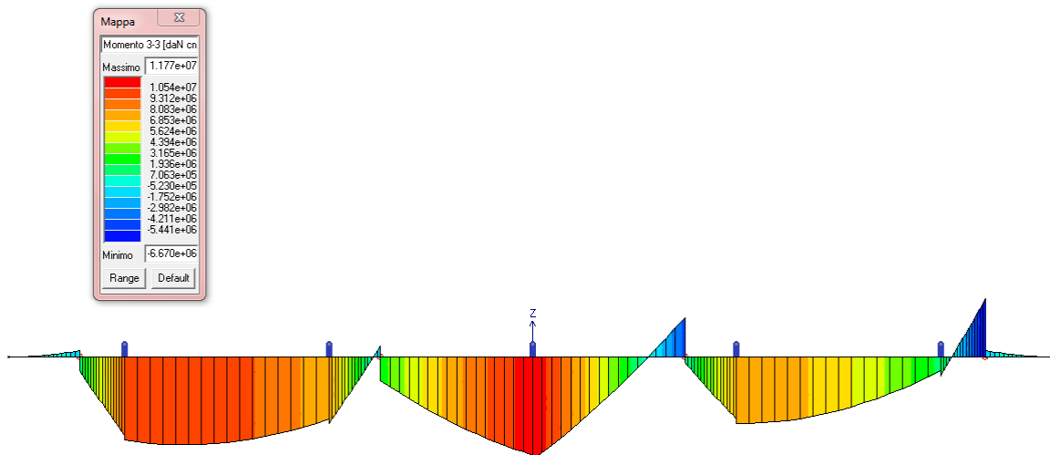
FIGURA 10-18 COMBINAZIONE SLD 1 : MOMENTO FLETTENTE
