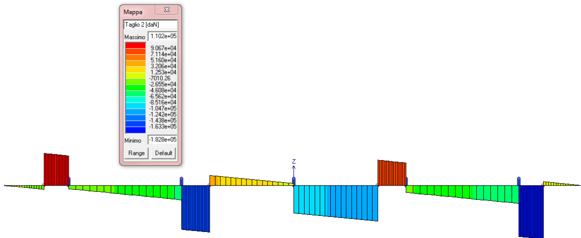
FIGURA 10-9 COMBINAZIONE SLV 1 : TAGLIO
