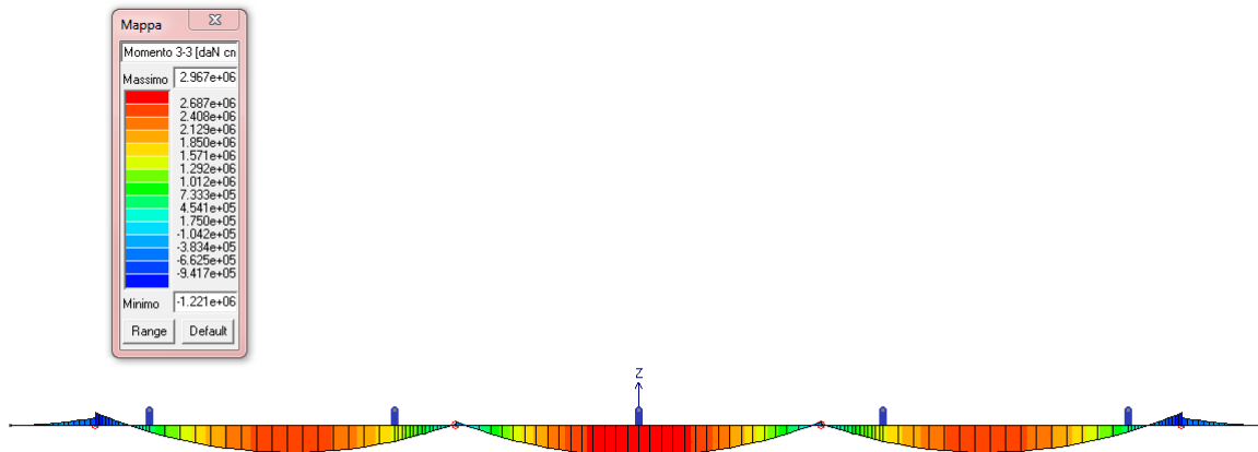
FIGURA 10-16 COMBINAZIONE SLE QUASI PERMANENTE 1 : MOMENTO FLETTENTE
