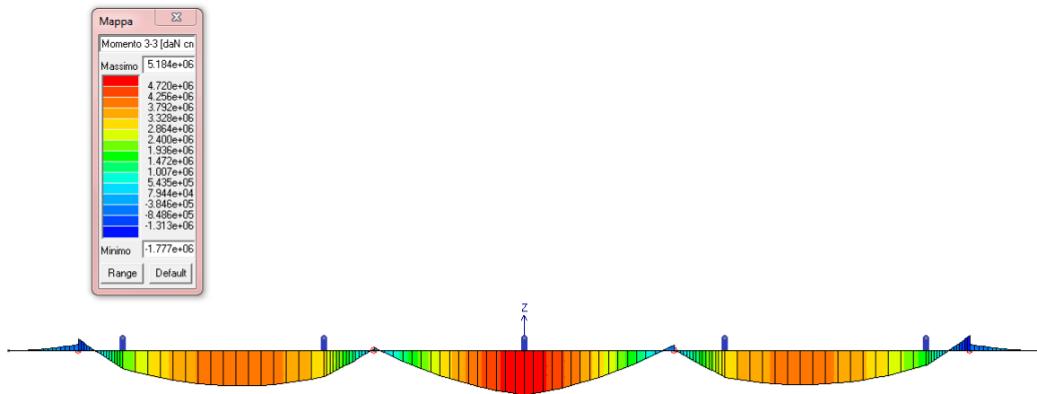
FIGURA 10-12 COMBINAZIONE SLE RARA 1 : MOMENTO FLETTENTE
