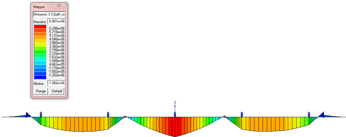
FIGURA 10-14 COMBINAZIONE SLE FREQUENTE 1 : MOMENTO FLETTENTE
