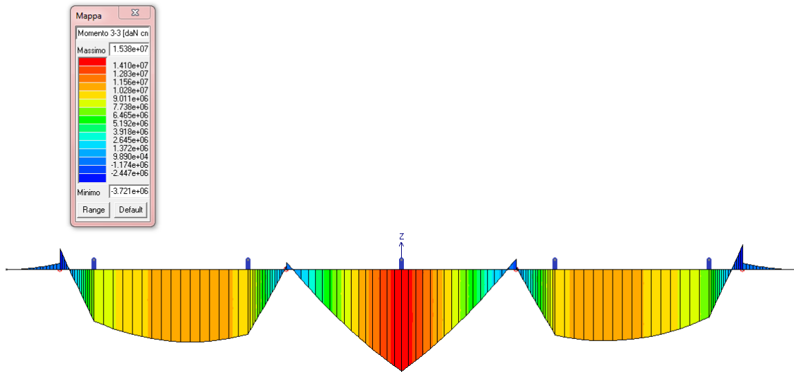
FIGURA 10-6 COMBINAZIONE SLU 2 : MOMENTO FLETTENTE
