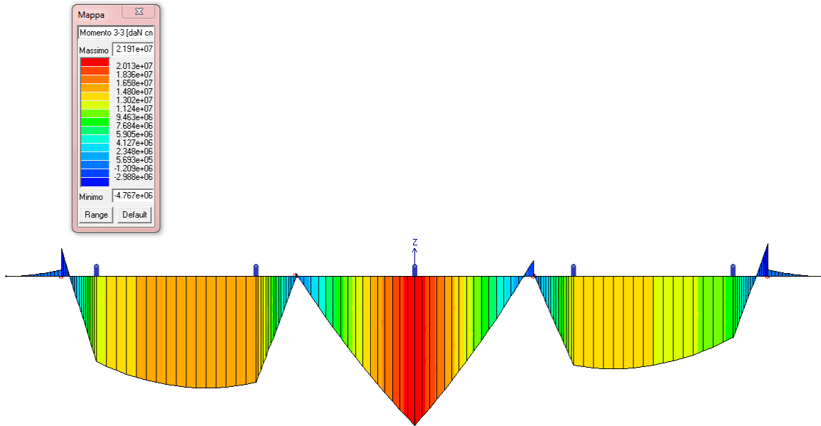
FIGURA 10-4 COMBINAZIONE SLU 1 : MOMENTO FLETTENTE
