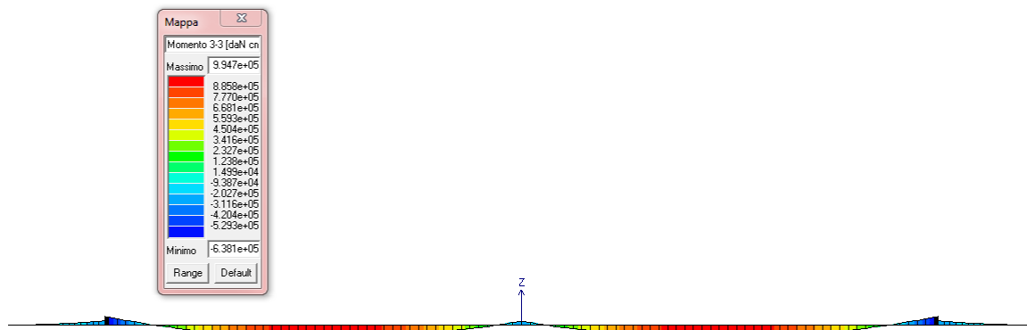
FIGURA 10-16 COMBINAZIONE SLE QUASI PERMANENTE 1 : MOMENTO FLETTENTE
