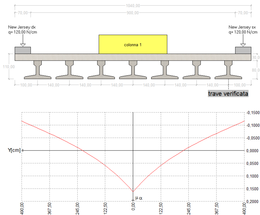
Diagramma coeff. \mu di influenza del traverso, configurazione del carico per M max
