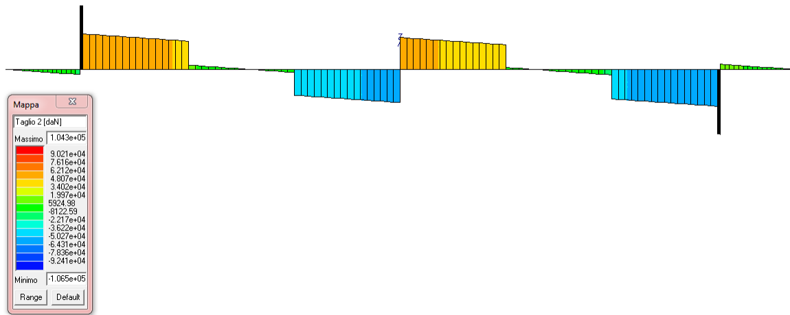
FIGURA 10-7 COMBINAZIONE SLU 2 : TAGLIO
