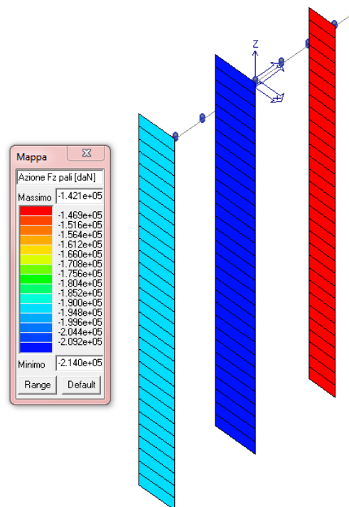
FIGURA 5.1.11-1 CARICO SU PALO
