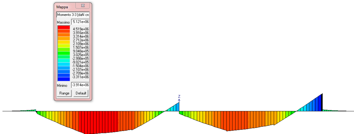
FIGURA 10-18 COMBINAZIONE SLD 1 : MOMENTO FLETTENTE
