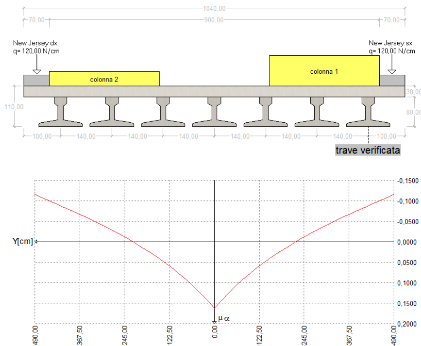
Diagramma coeff. \mu di influenza del traverso, configurazione del carico per M min
