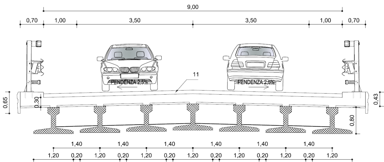
FIGURA 1-1 SEZIONE TRASVERSALE TIPICA
