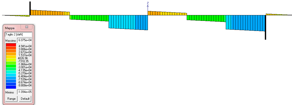
FIGURA 10-9 COMBINAZIONE SLV 1 : TAGLIO
