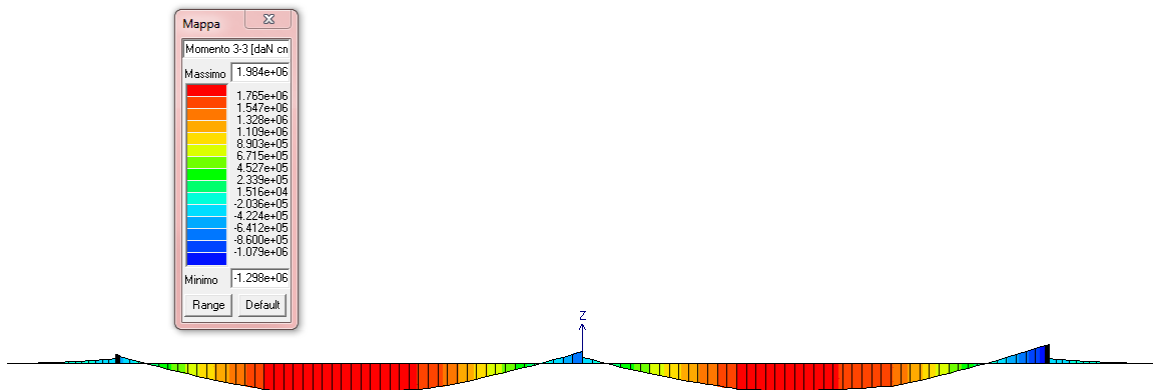
FIGURA 10-14 COMBINAZIONE SLE FREQUENTE 1 : MOMENTO FLETTENTE
