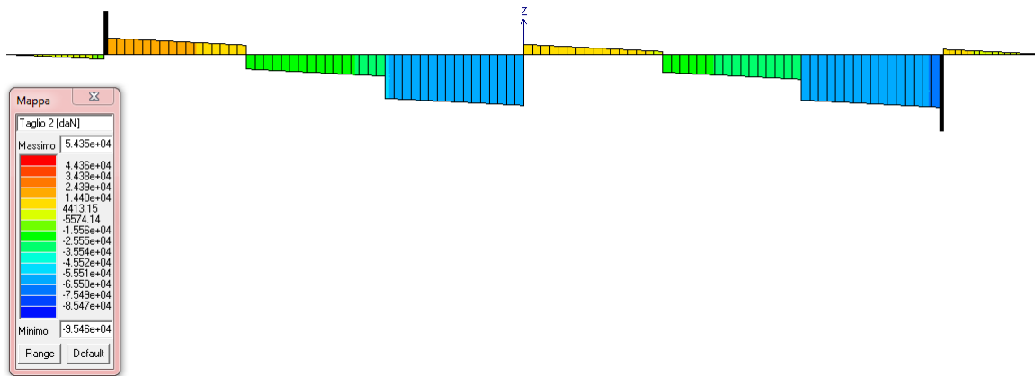
FIGURA 10-11 COMBINAZIONE SLV 2 : TAGLIO
