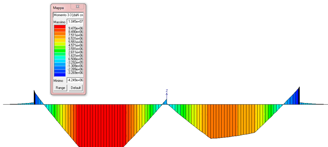
FIGURA 10-4 COMBINAZIONE SLU 1 : MOMENTO FLETTENTE
