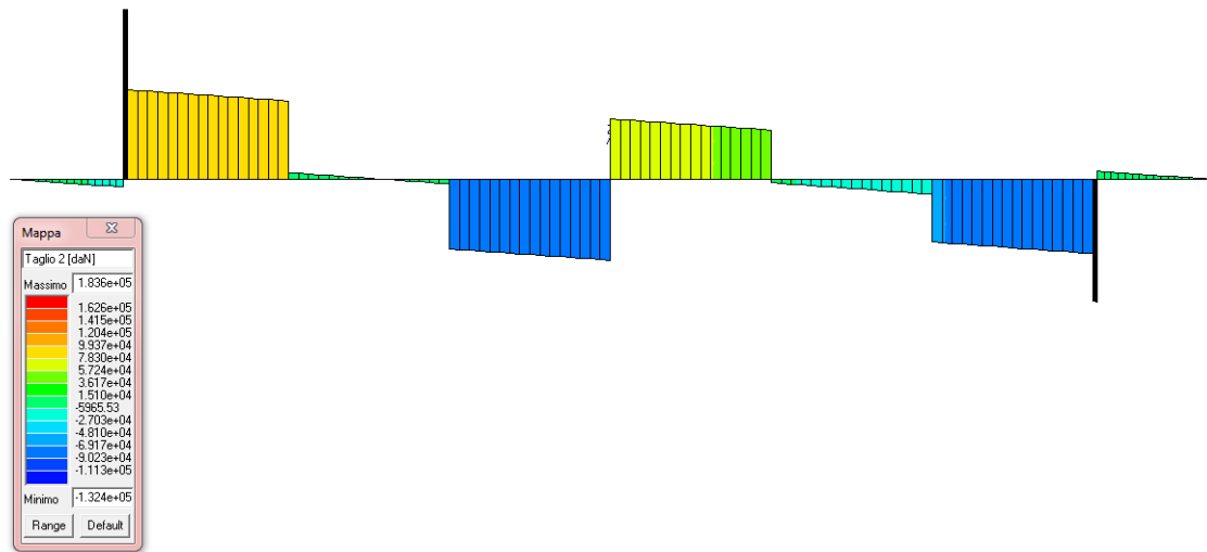
FIGURA 10-5 COMBINAZIONE SLU 1 : TAGLIO
