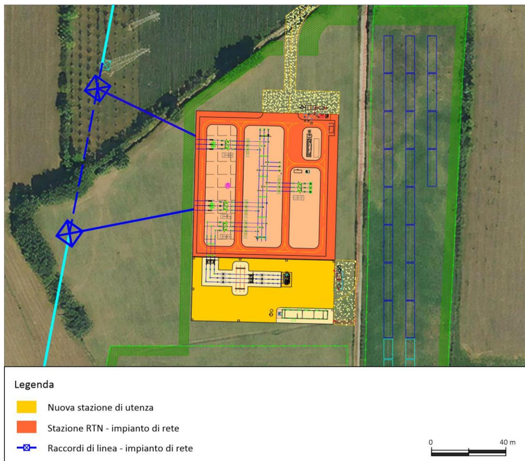
Figura.2- Lay out generale Impianto di Utenza e Impianto di Rete
