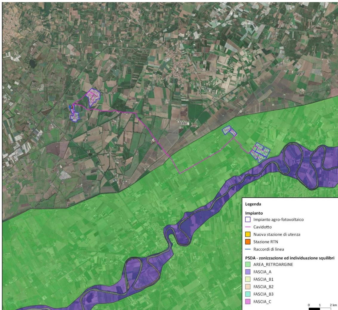
Figura.6- Estratto cartografia PSDA e PSDA - bav (Perimetrazione vigente)
