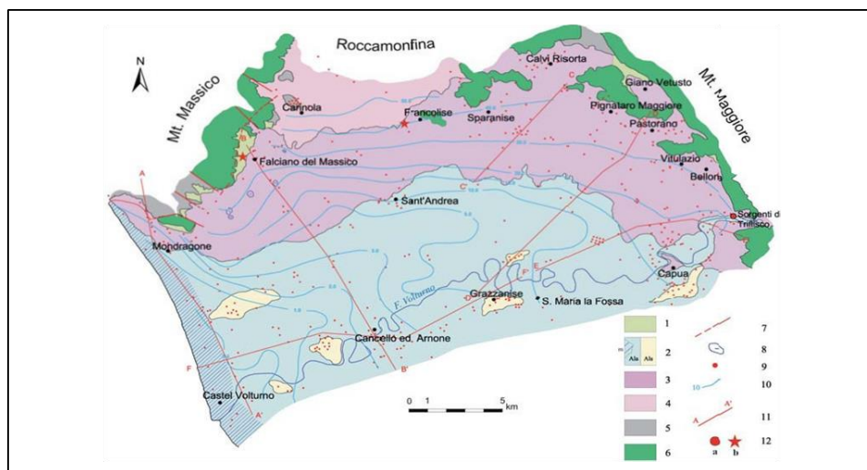
Figura.4- Schema idrogeologico ed assetto piezometrico.
