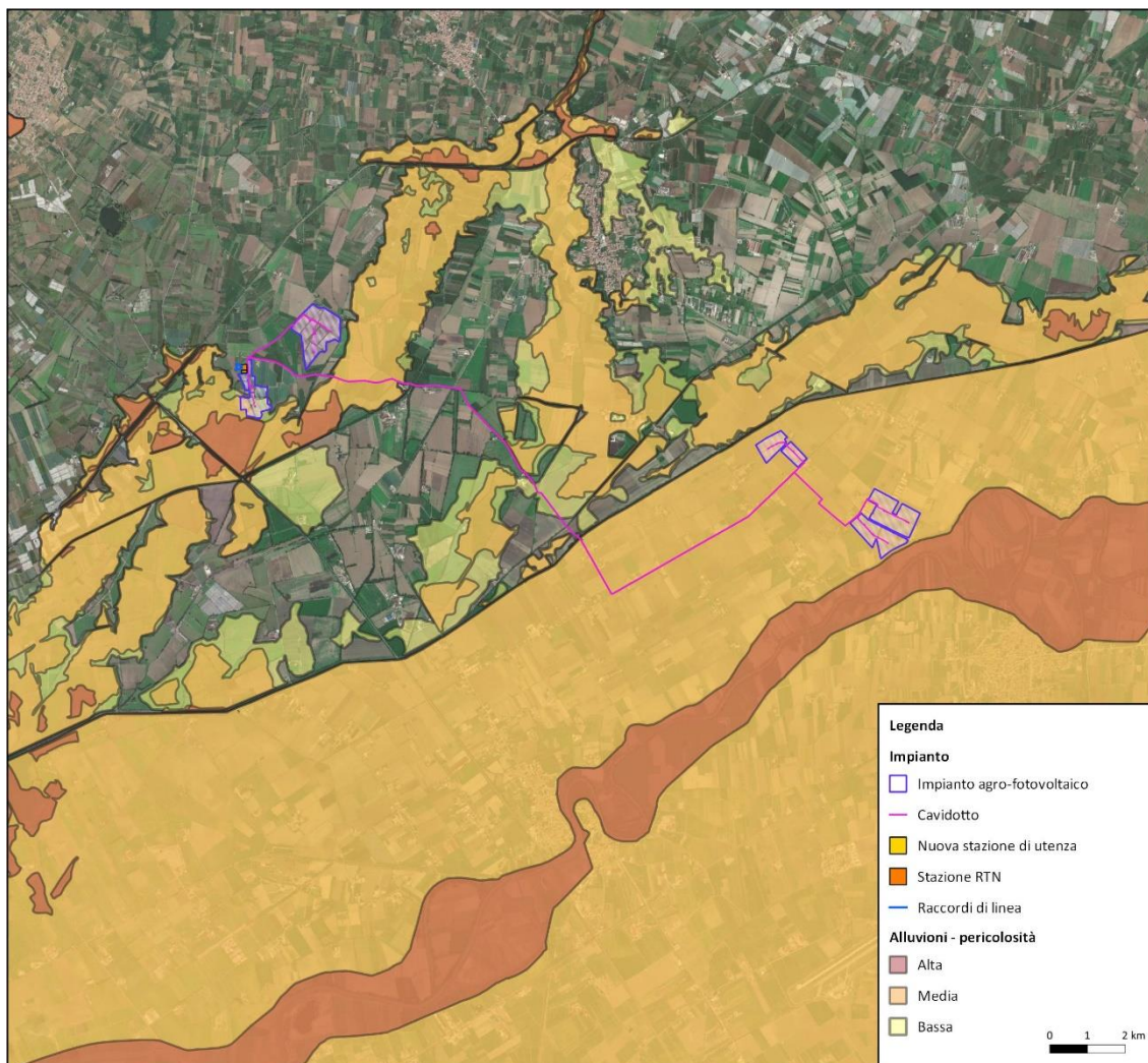
Figura.8- Estratto cartografia PGRA – Mappe Pericolosità alluvione
