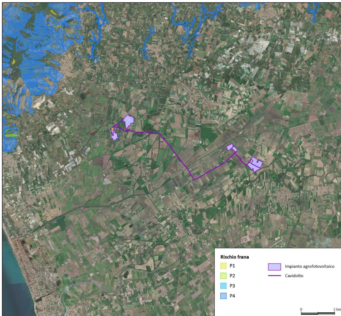
Figura.7- Mappa con ubicazione delle aree a rischio frana (Estratto cartografia PAI)
