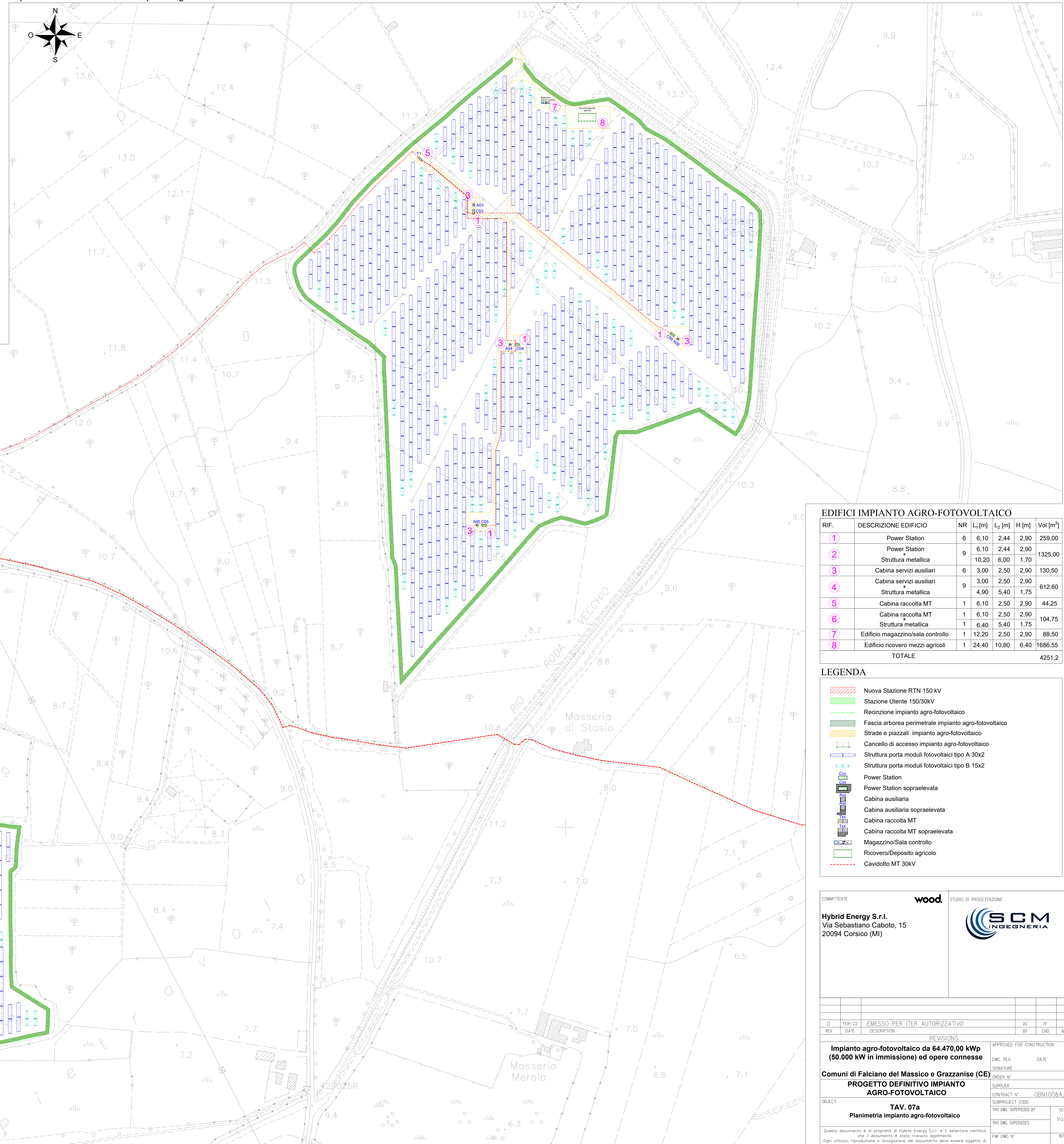
Inquadramento area 1 e area 2 impianto agro-fotovoltaico - Scala 1:2000
