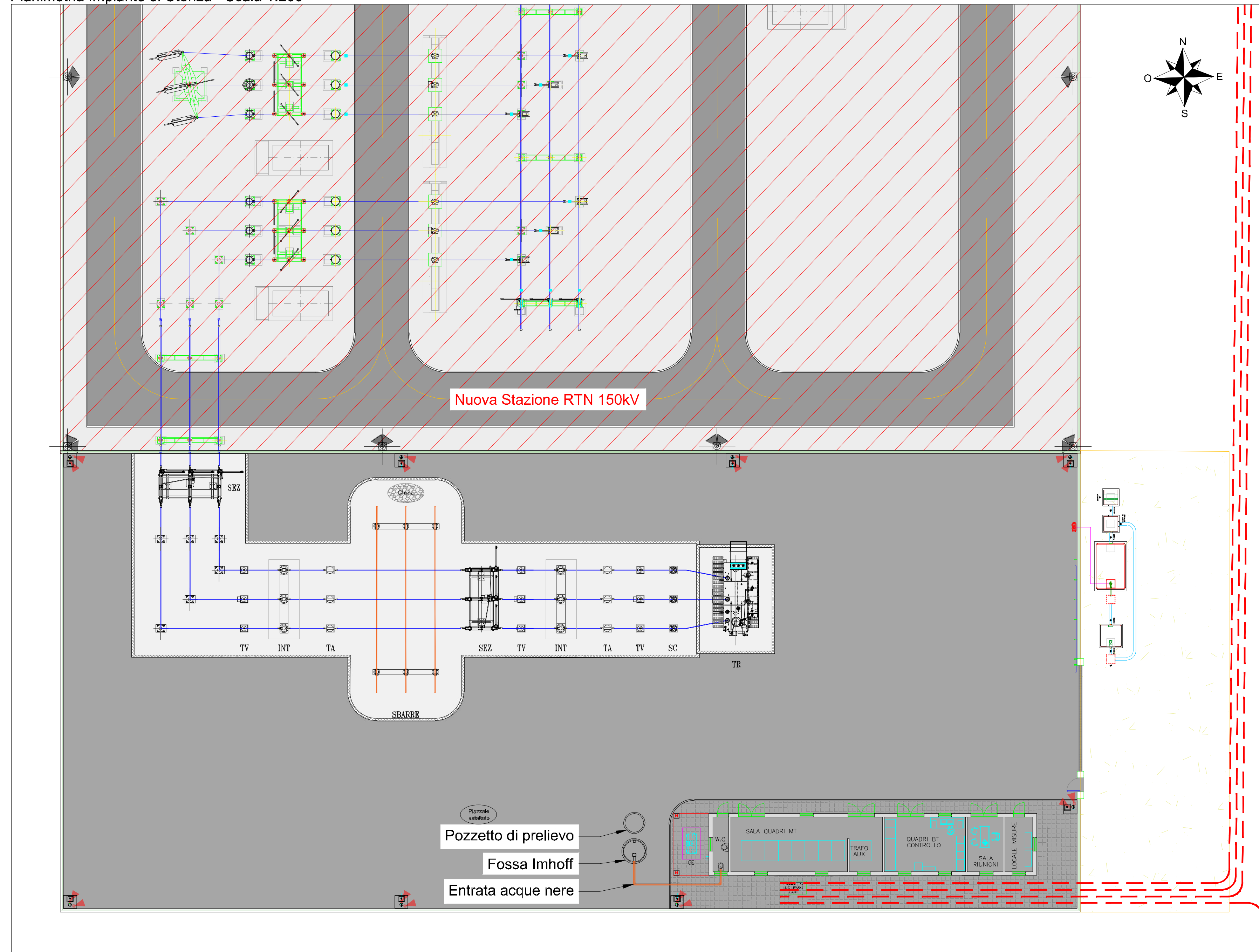
Planimetria Impianto di Utenza con dettaglio sistema di smaltimento acque nere - Scala 1:100
