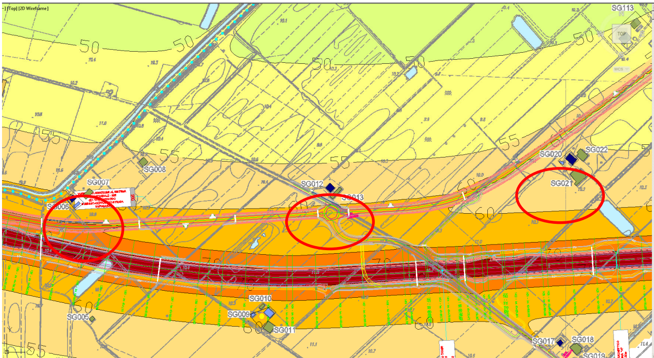
FIGURA 6.5-7 – DETTAGLIO DELLA MAPPATURA DELLE ISOFONICHE IN CORRISPONDENZA DEI RICETTORI SG006-SG012 E SG020
