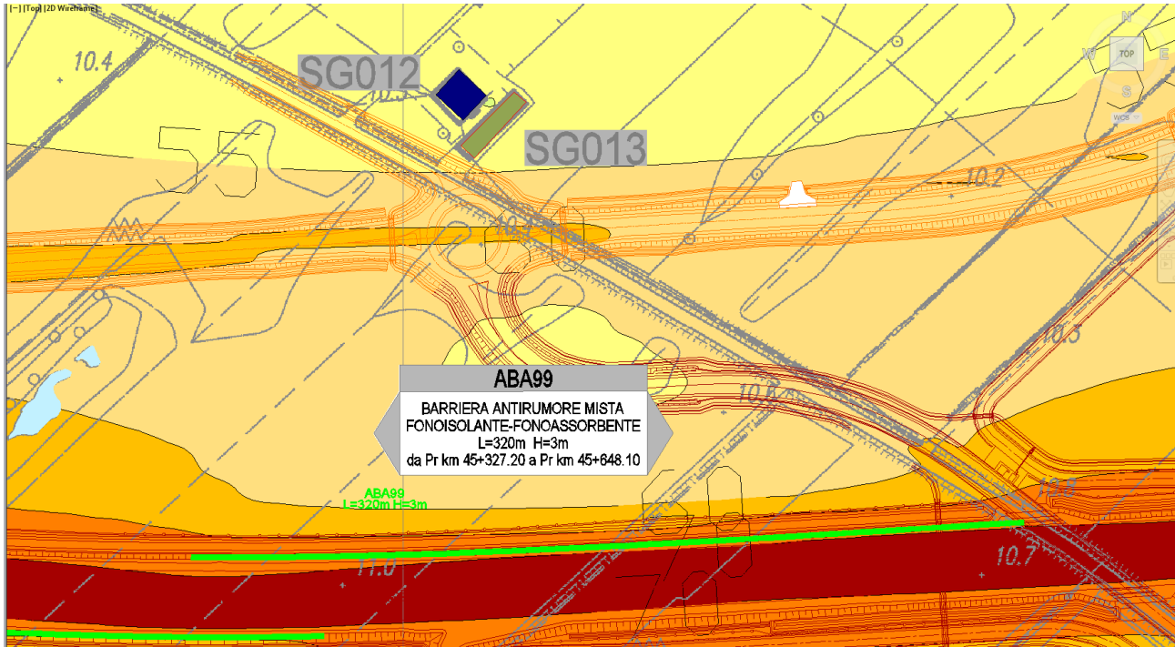
FIGURA 8.3-2 – DETTAGLIO DELLA MAPPATURA DELLE ISOFONICHE IN CORRISPONDENZA DEL RICETTORE SG012
