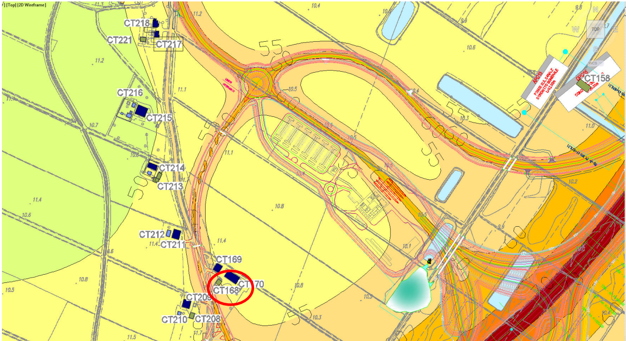
FIGURA 6.5-3 – DETTAGLIO DELLA MAPPATURA DELLE ISOFONICHE IN CORRISPONDENZA DEL RICETTORE CT168
