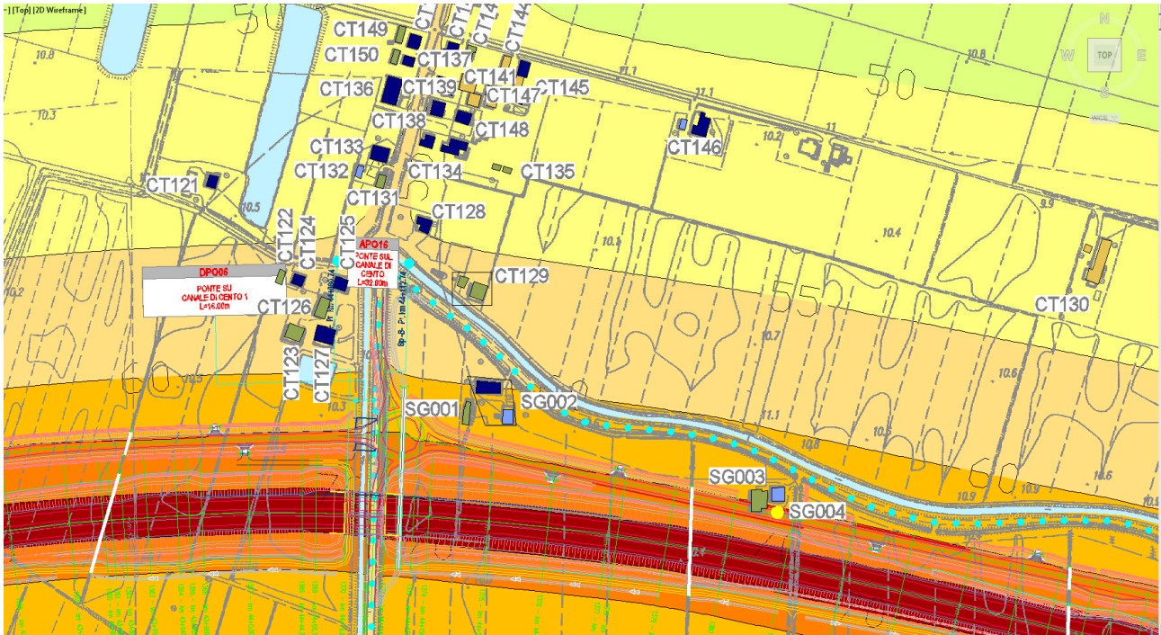
FIGURA 6.5-6 – DETTAGLIO DELLA MAPPATURA DELLE ISOFONICHE IN CORRISPONDENZA DEL RICEITTORE SG012
