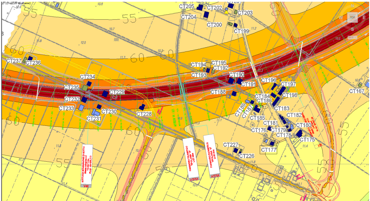
FIGURA 6.5-2 – DETTAGLIO DELLA MAPPATURA DELLE ISOFONICHE IN CORRISPONDENZA DEI RICETTORI CT184-CT232
