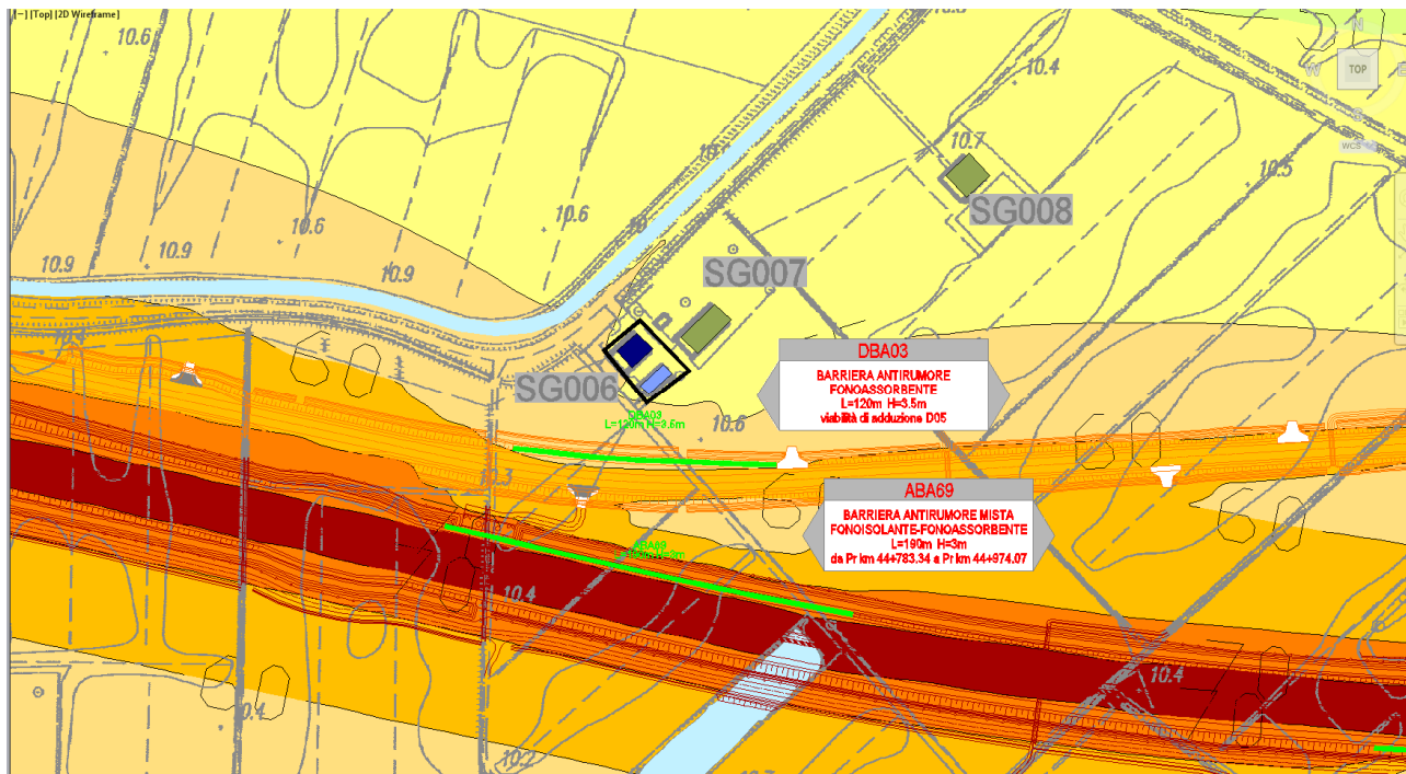
FIGURA 8.3-1 – DETTAGLIO DELLA MAPPATURA DELLE ISOFONICHE IN CORRISPONDENZA DEL RICETTORE SG006
