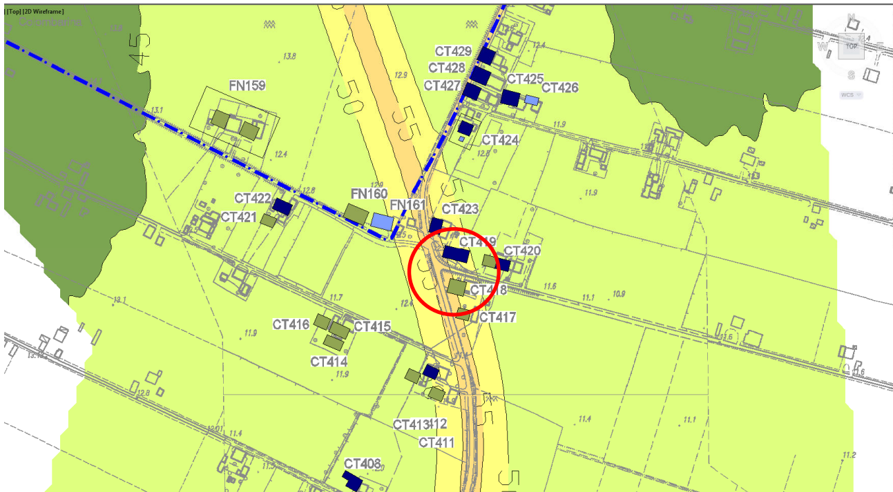
FIGURA 6.5-5 – DETTAGLIO DELLA MAPPATURA DELLE ISOFONICHE IN CORRISPONDENZA DEI RICETTORI CT419 E 423
