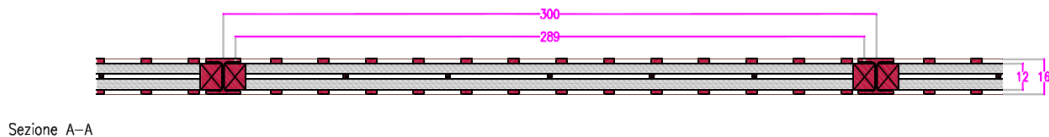
FIGURA 7.2-2 – SEZIONE ORIZZONTALE DELLA BARRIERA ACUSTICA IN LEGNOI
