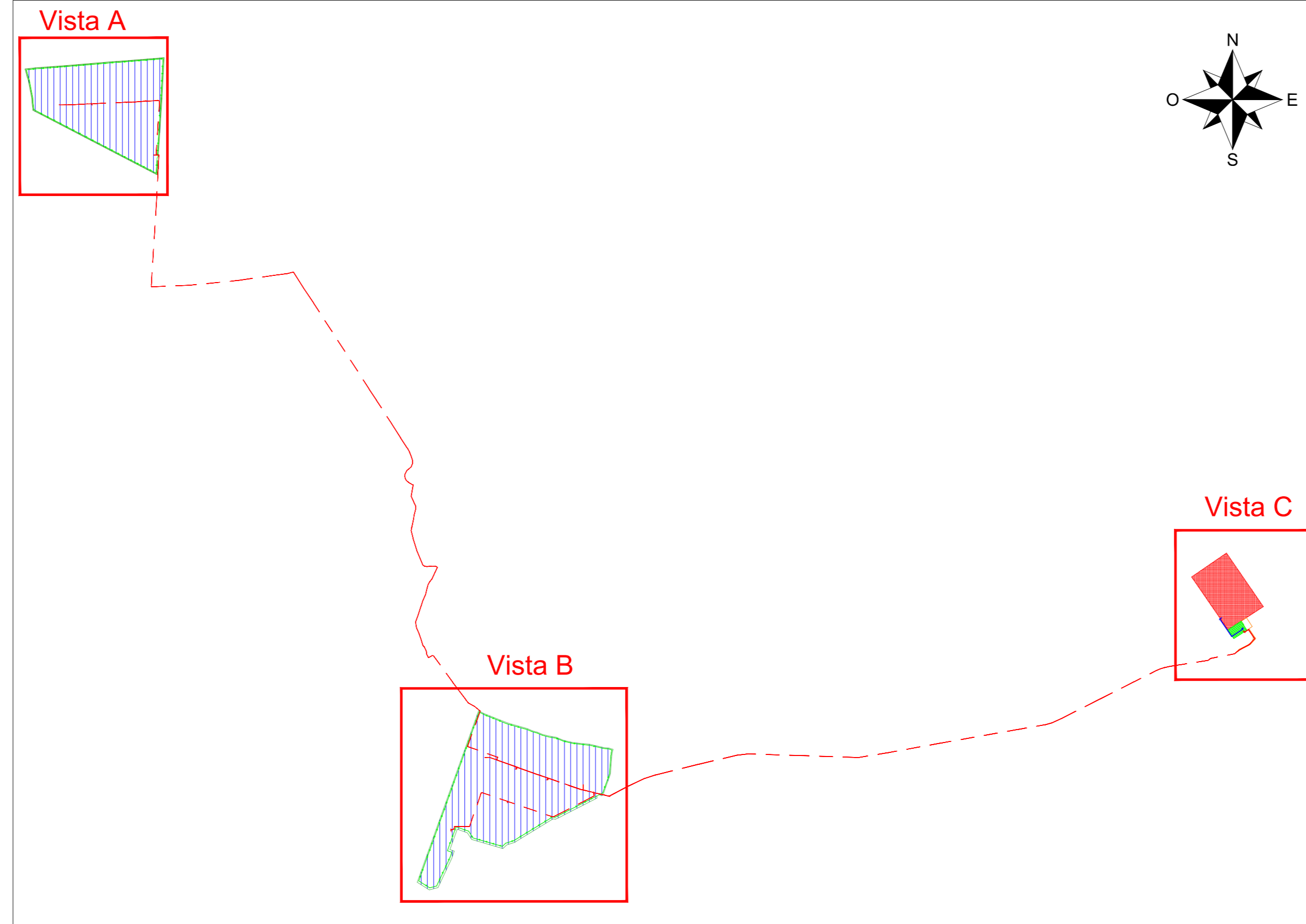
Layout impianto - Scala 1:20000
