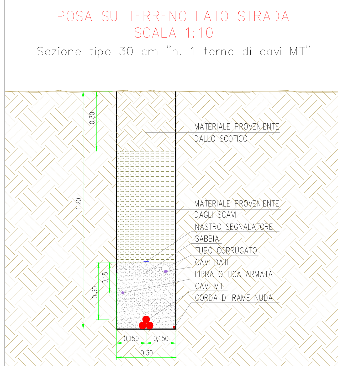
Posa MT - sezione tipo 30 cm - SCALA 1:10
