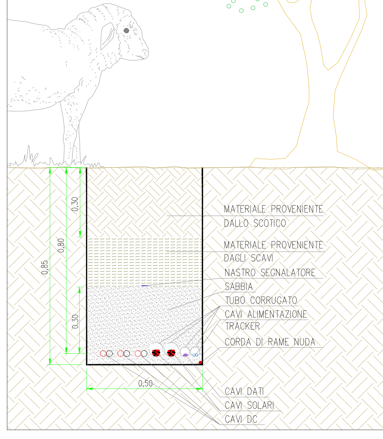
Posa su terreno agricolo - sezione tipo 50 cm - SCALA 1:10
