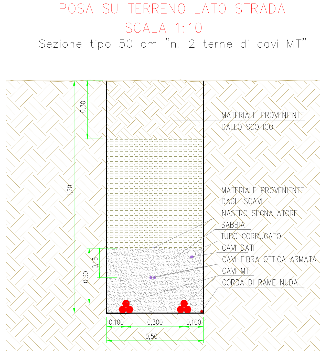
Posa MT - sezione tipo 50 cm - SCALA 1:10
