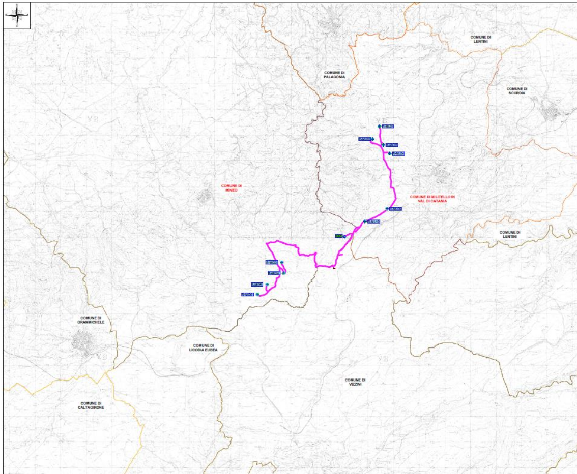
Fig.2- Inquadramento impianto su IGM 1:25.000
