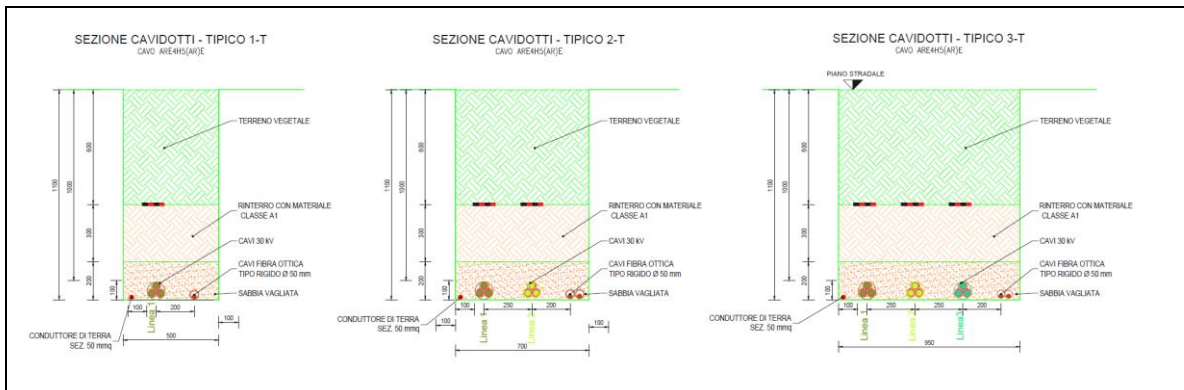
Fig. 19 – Sezioni tipo di scavo su terreno vegetale
