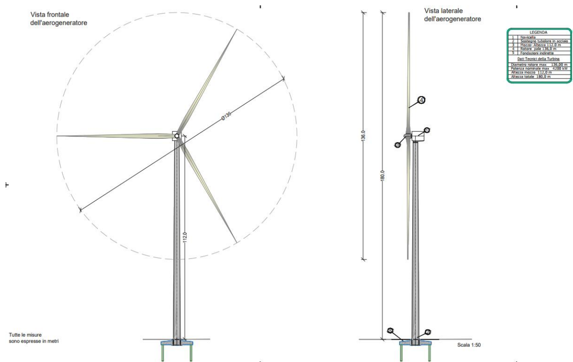
Fig.4 Schema tipo aerogeneratore
