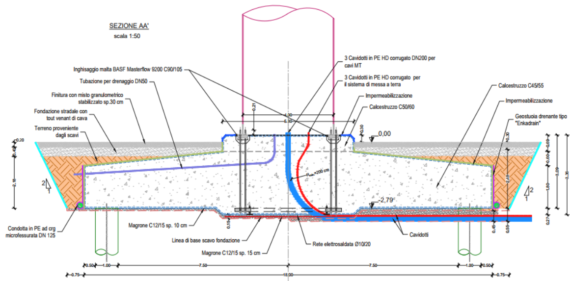
Fig.11 Sezione del plinto
