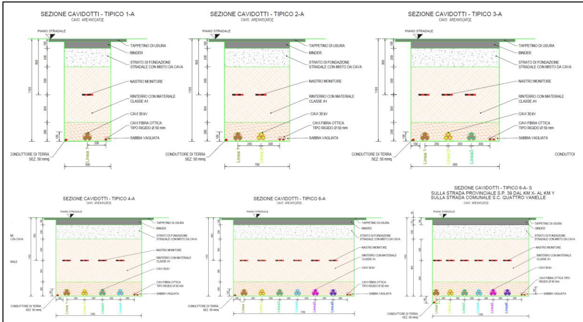
Fig. 17 – Sezioni tipo di scavo su strade asfaltate
