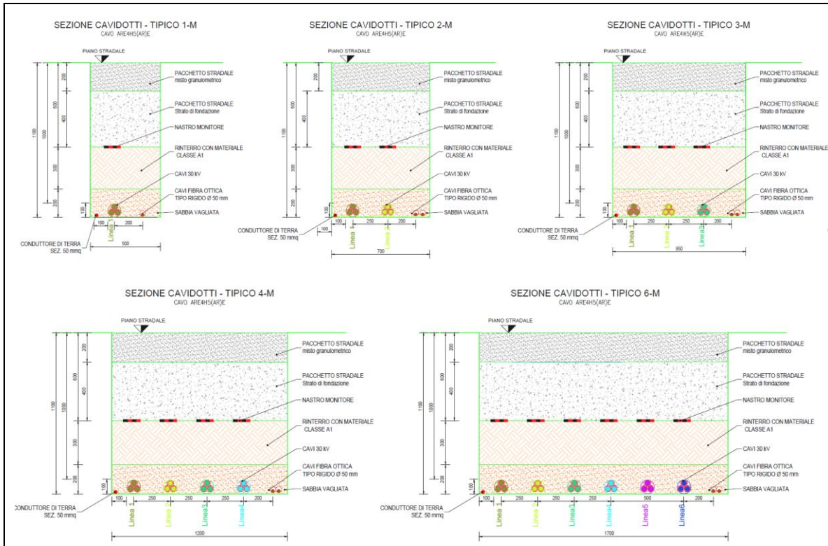
Fig. 18 – Sezioni tipo di scavo su strade sterrate
