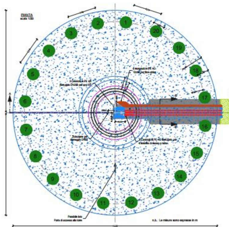
Fig.10 Pianta del plinto con indicazione dei pali di fondazione (n.20 del diametro 100 cm)
