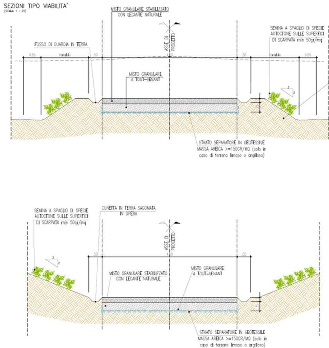
Figura 5: Sezioni stradali tipo
