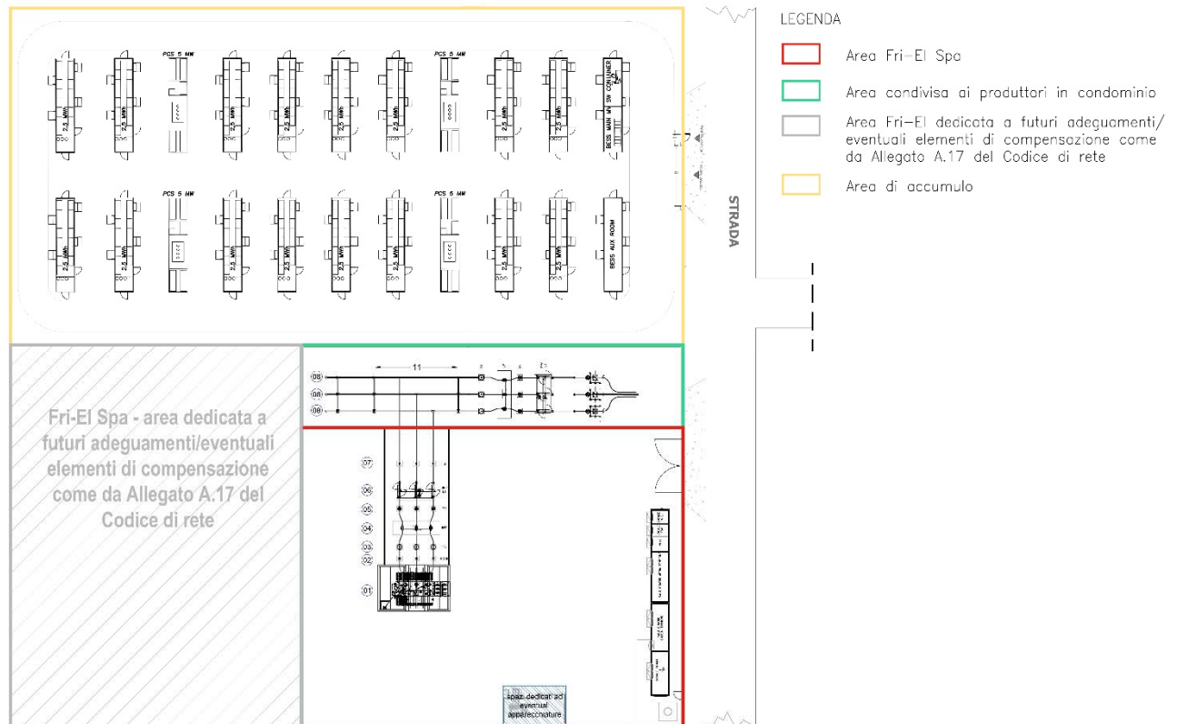
Figura 6: Planimetria SET
