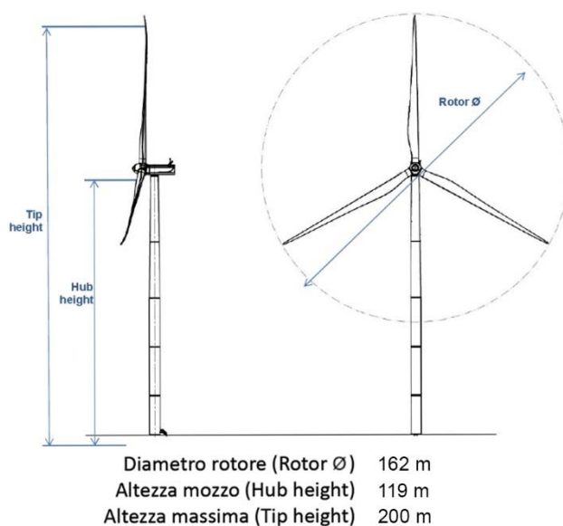
Figura 4: Vista aerogeneratore
