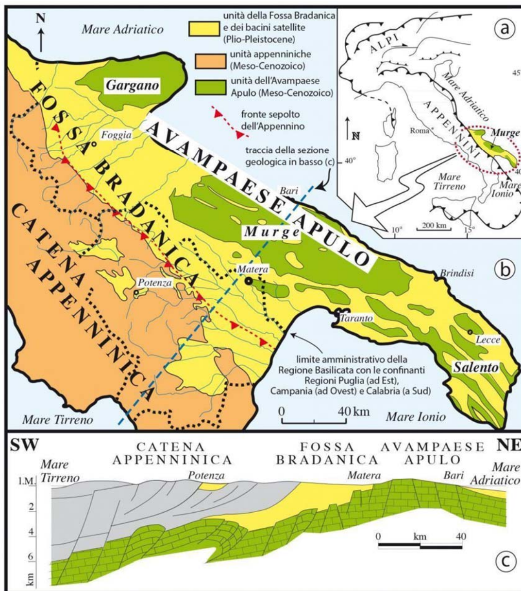
Figura 8 Carta geologica schematica della Puglia e delle aree limitrofe
