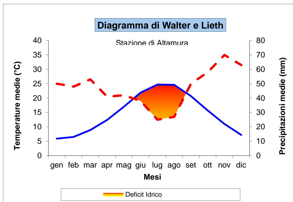
Figura 7: diagramma di Walter e Lieth
